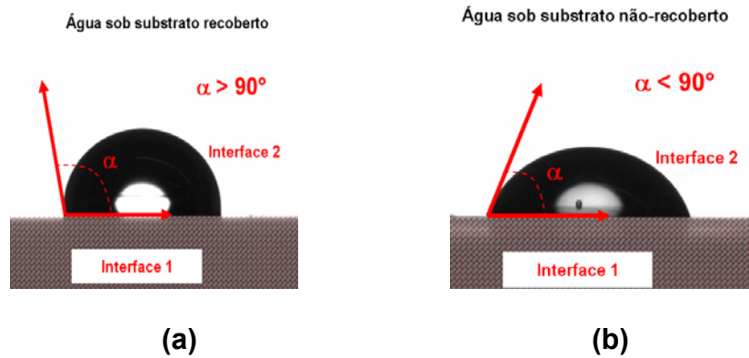
Figura 24. Ângulo de molhamento de uma gota de água destilada sobre: (a) filme de PET com revestimento de silicone, (b) filme de PET sem recobrimento de silicone.
