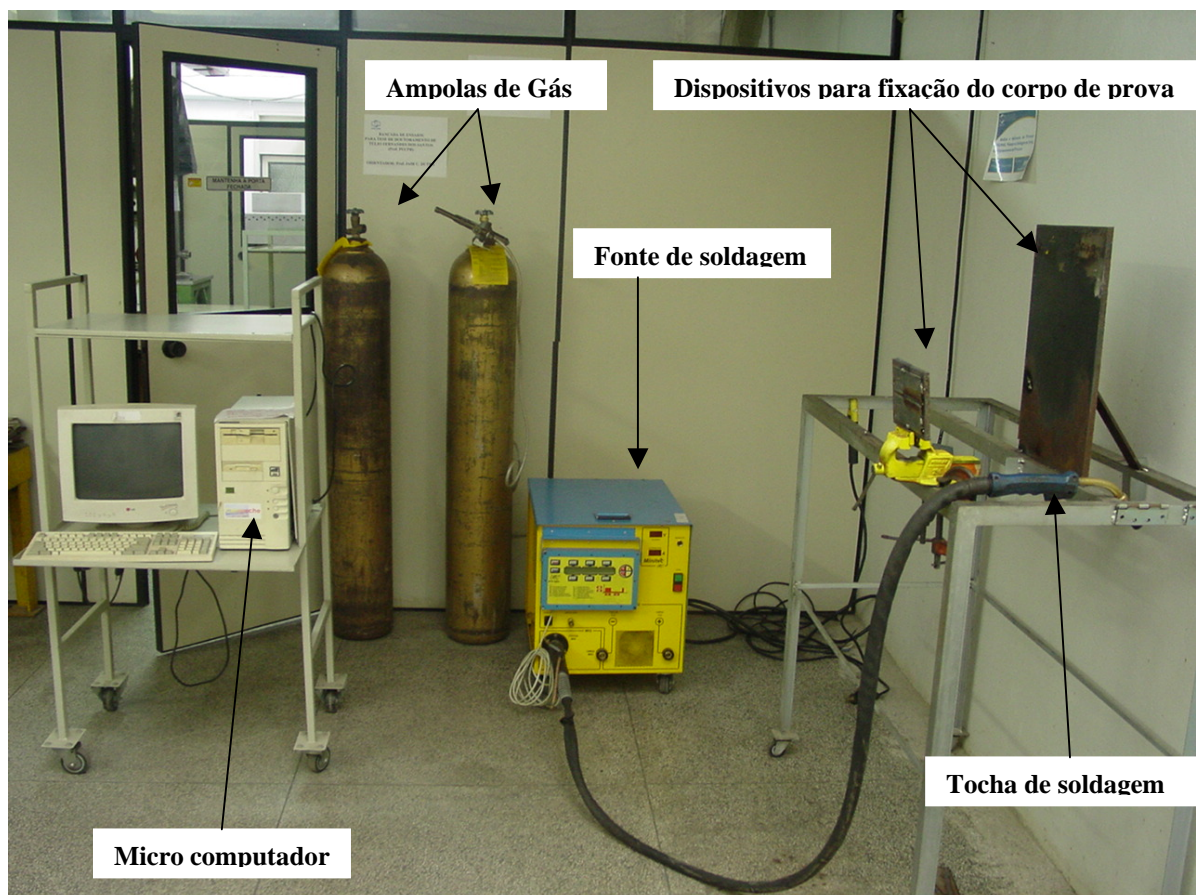
Figura 22 – Bancada de ensaios
