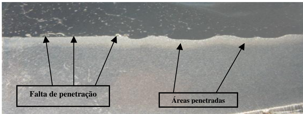
Figura 43 – Corte longitudinal de amostra do MAG-PT mostrando áreas com penetração e sem penetração (aumento 5x)
