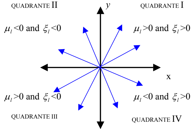
Figura 3.11- O domínio angular e seus 4 quadrantes.
