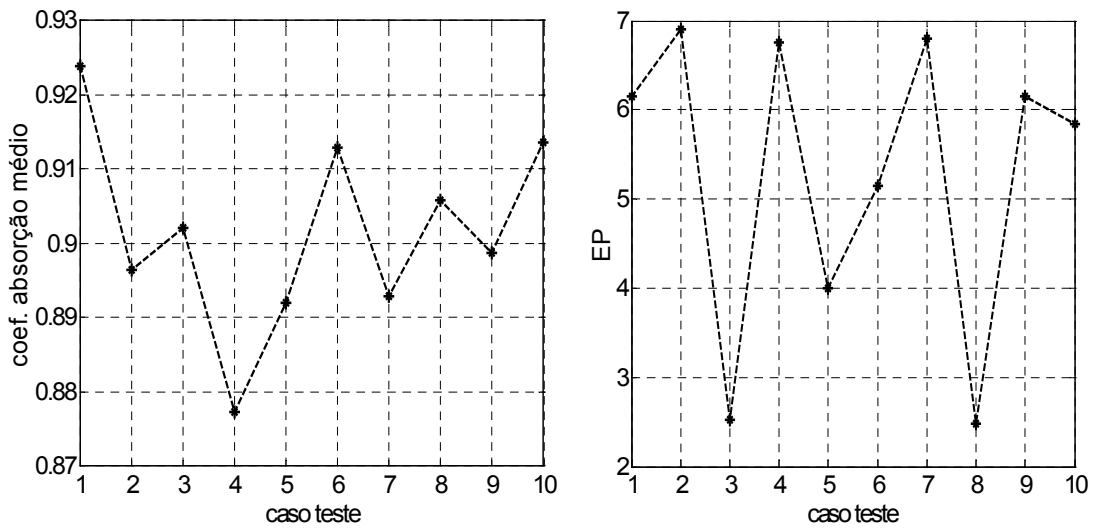
Fig. 5.15c – Estimativa de \sigma_a . Exemplo 2, meio homogêneo, com DE=6.
