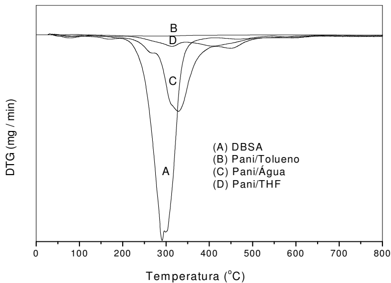
Figura 15. Derivada do TGA para o DBSA e Pani sintetizada em tolueno, água ou THF.
