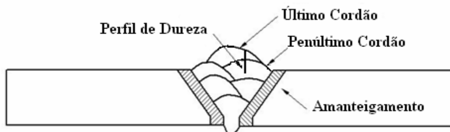
Figura 34 - Esquema da macroestrutura da solda e do cordão onde foram realizados os ensaios.
