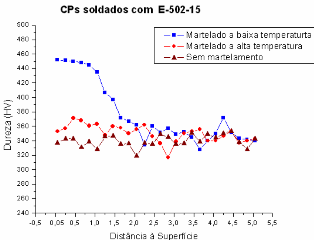
Figura 63 – Valores das microdurezas realizadas nos CPs E-502-15.
