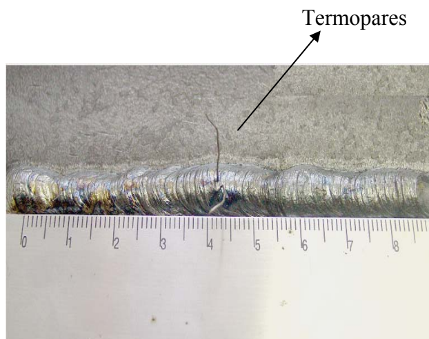
Figura 35 – Região onde o termopar foi imerso para a aquisição da taxa de resfriamento, E-7018, T= 20 segundos, I= 125A.
