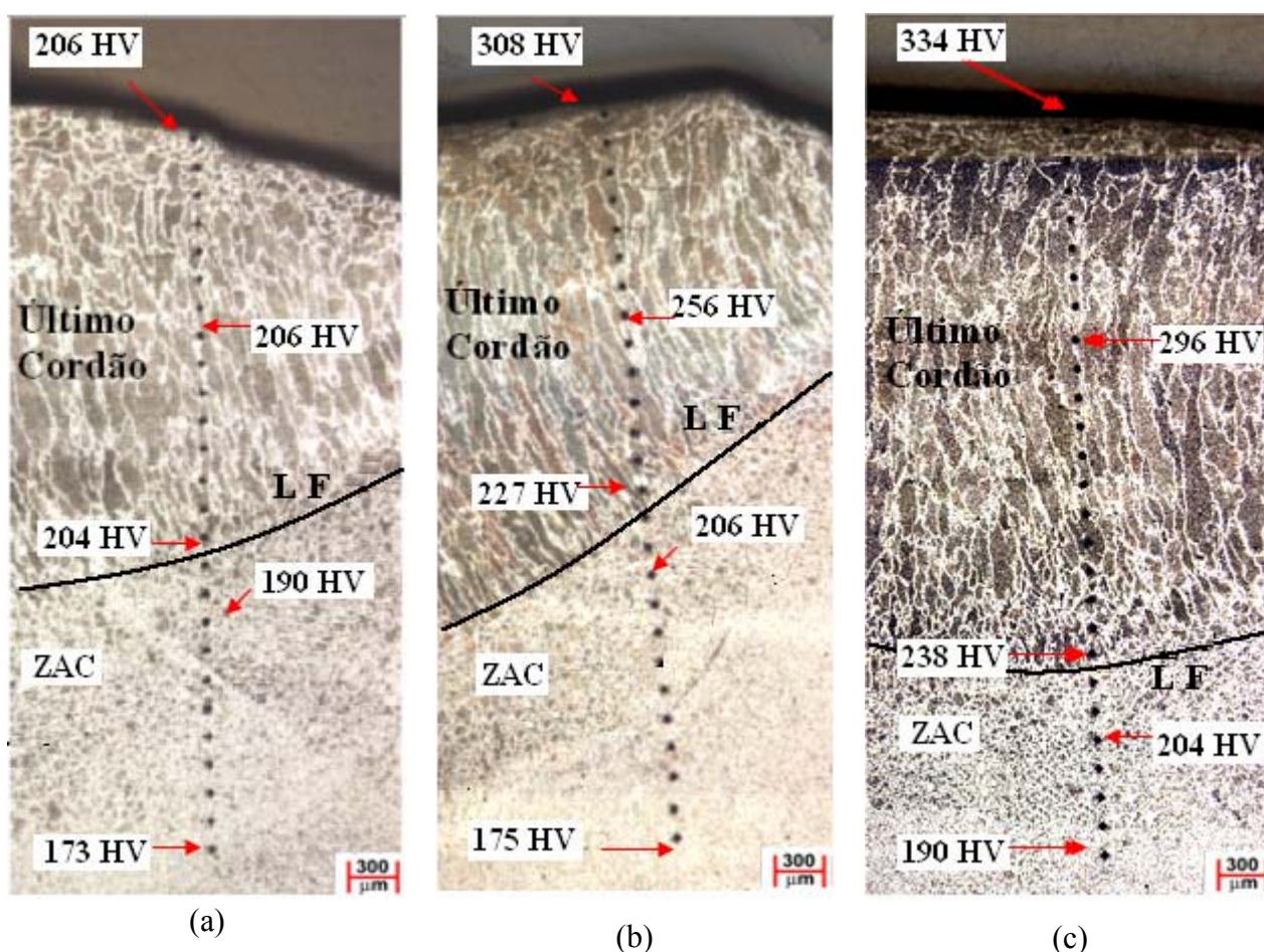
Figura 45 – Micrografias do último cordão onde podem ser observadas as impressões de dureza: (a) CP sem Martelamento, (b) CP martelado a alta temperatura, (c) CP martelado a baixa temperatura.
