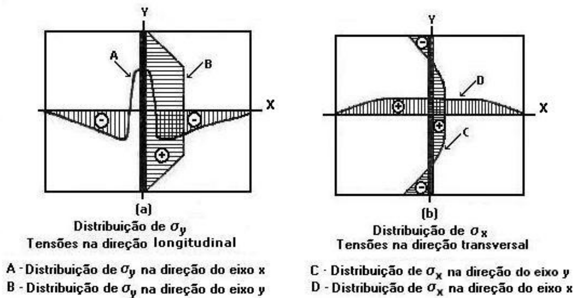
Figura 3 - Distribuição típica de tensões residuais em uma união de topo [4].
