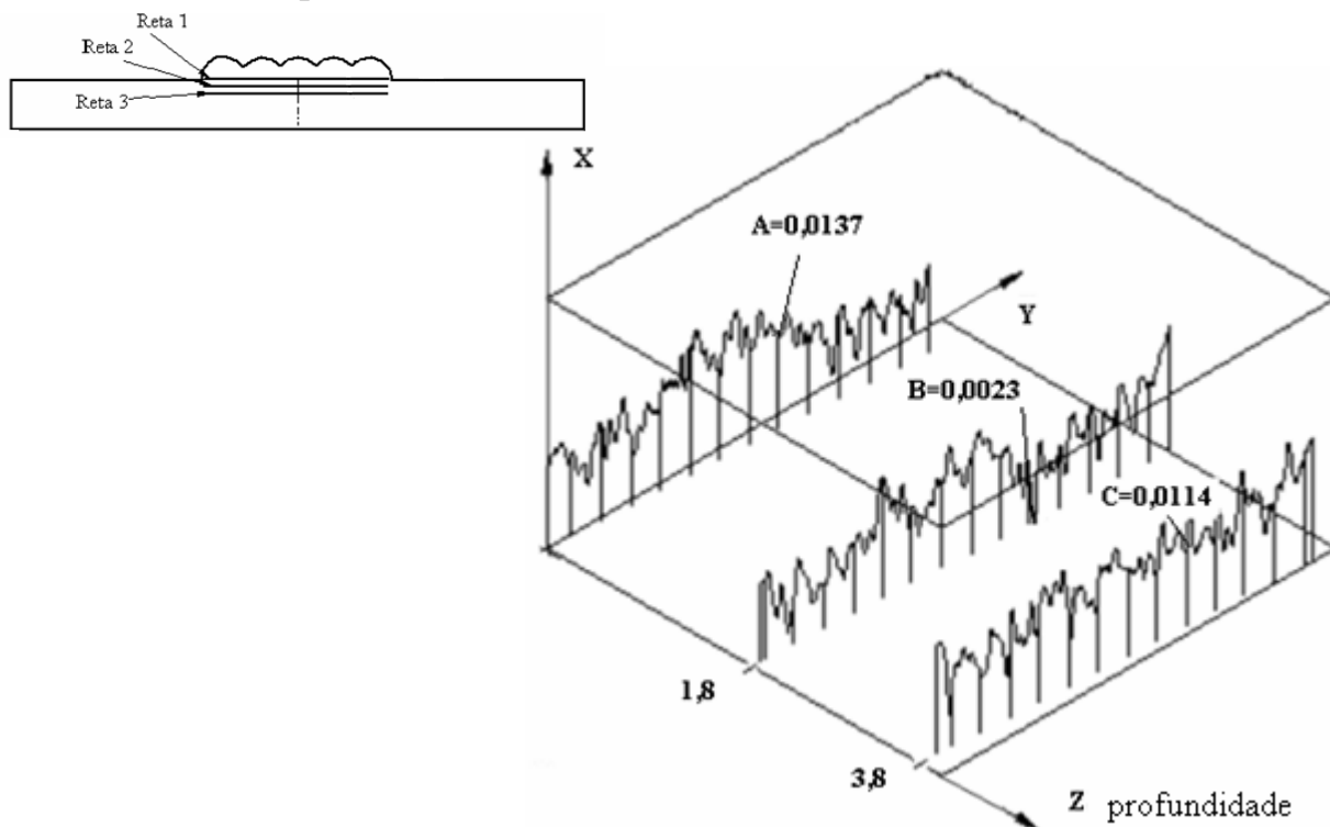
Figura 39 – Gráficos tridimensionais da planicidade encontrados em cada face (1-F 1 ; 2- F 1 ) espelhada, correspondendo ao martelamento a baixa temperatura.
