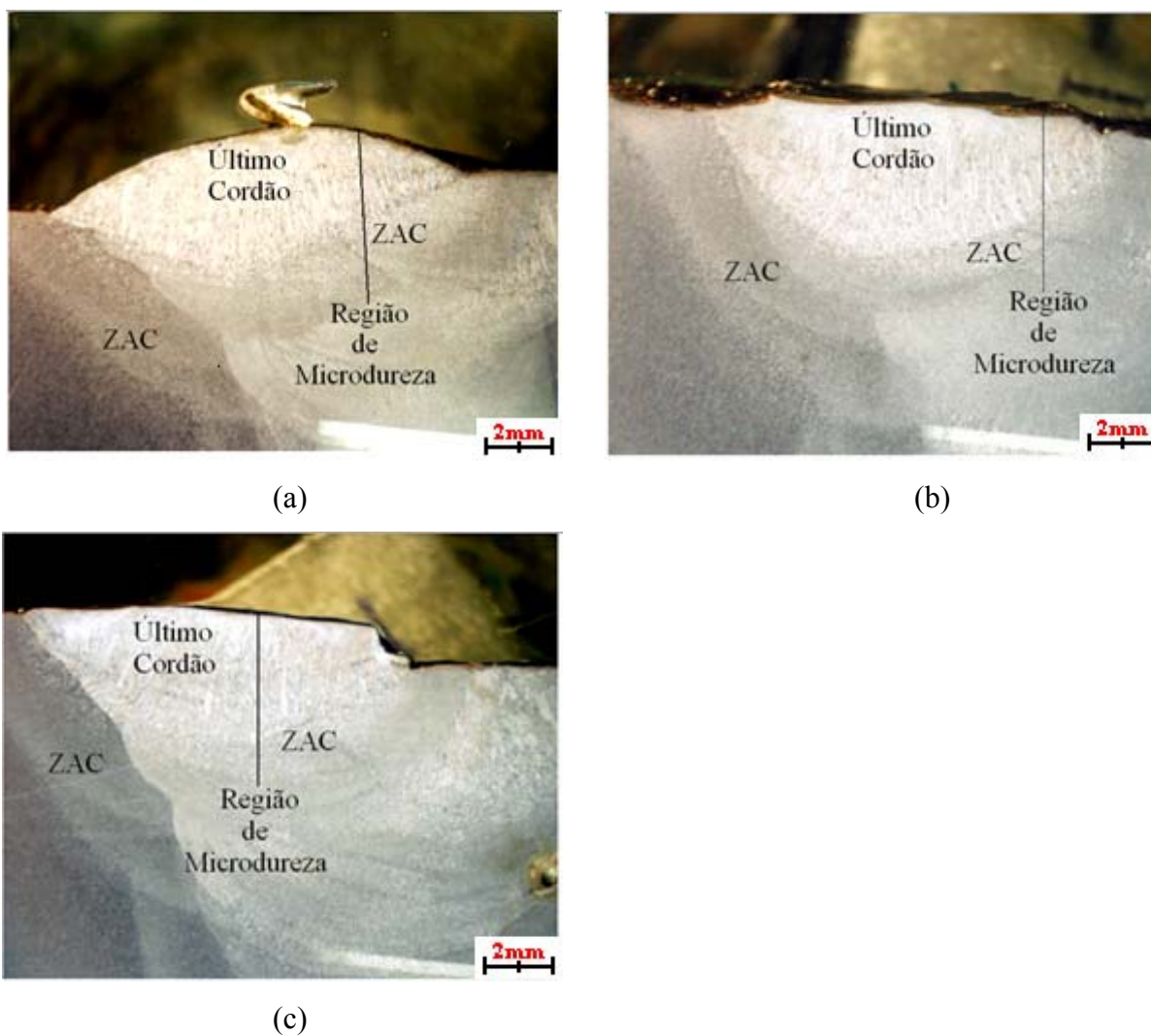
Figura 41 – Macrografias a 10x das soldas realizadas com metal de adição E-7018 ; (a) Sem martelamento; (b) com martelamento a alta temperatura; (c) com martelamento a baixa temperatura.
