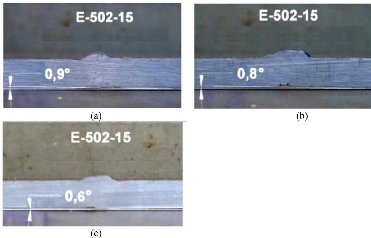
Figura 57 – Distorções angulares dos CPs soldados com eletrodo E-502-15; (a) Sem martelar; (b) Martelado a alta temperatura; (c) Martelado a baixa temperatura .
