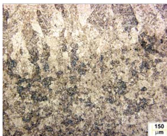
Figura 59 – Microestruturas na solda realizada sem martelamento; (a) Região próxima à superfície do cordão observada com dois aumentos diferentes; (1a) Região próxima à superfície do último cordão; (b) região central do cordão; (c) Linha de fusão entre o penúltimo e último cordões. Ataque Nital 2%
