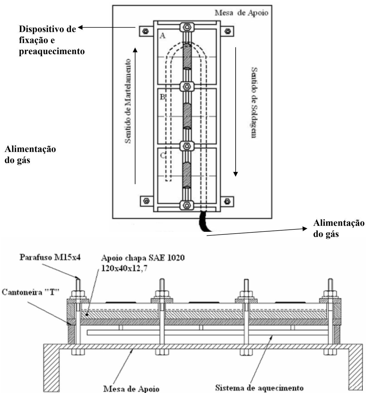
Figura 30 – Dispositivo utilizado para fixação e preaquecimento dos CPs.
