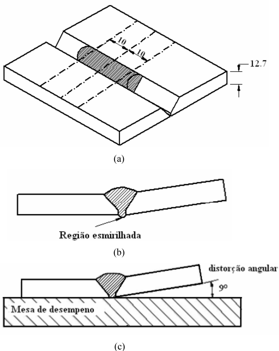
Figura 33 - Preparação das secções de corte onde serão avaliadas as distorções angulares: (a) Corte da secção transversal; (b) desbaste do excesso de material do passe de raiz; (c) medição da distorção.
