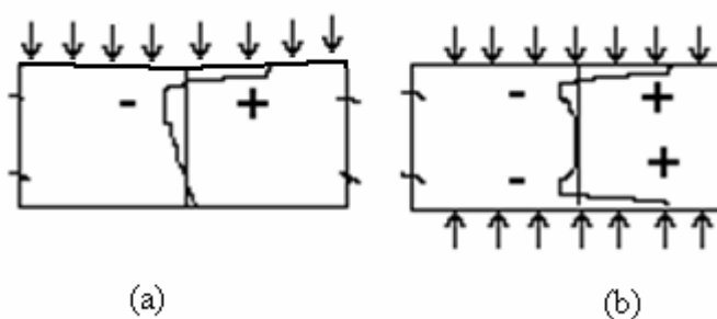
Figura 13 – Distribuição das tensões produzidas numa chapa jateada: (a) pelo lado suspenso; (b) pelos os dois lados.
