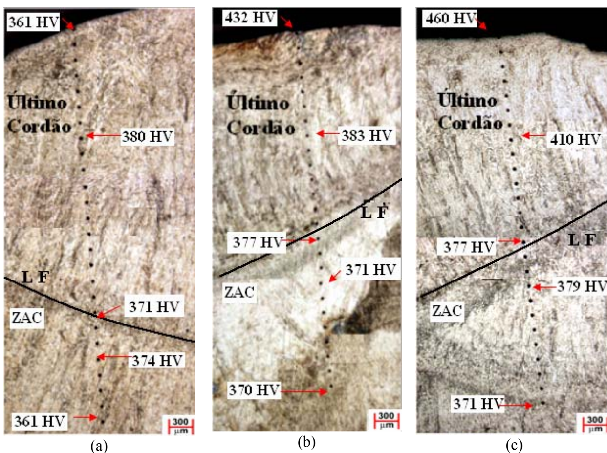
Figura 70 - Micrografias do último cordão onde podem ser observadas as impressões de dureza: (a) CP sem Martelamento, (b) CP martelado a alta temperatura, (c) CP martelado a baixa temperatura.
