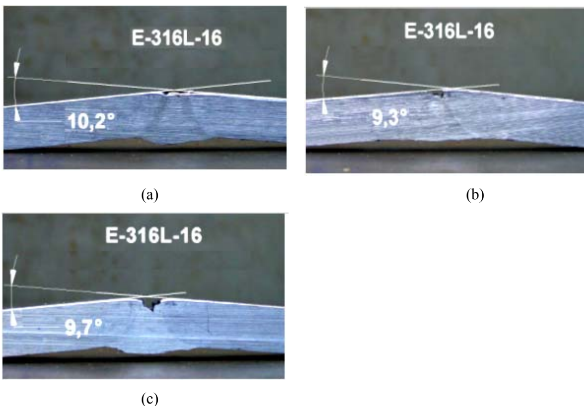
Figura 48 – Distorções angulares dos CPs soldados com eletrodo E-316L-16; (a) Sem martelar; (b) Martelado a alta temperatura; (c) Martelado a baixa temperatura .
