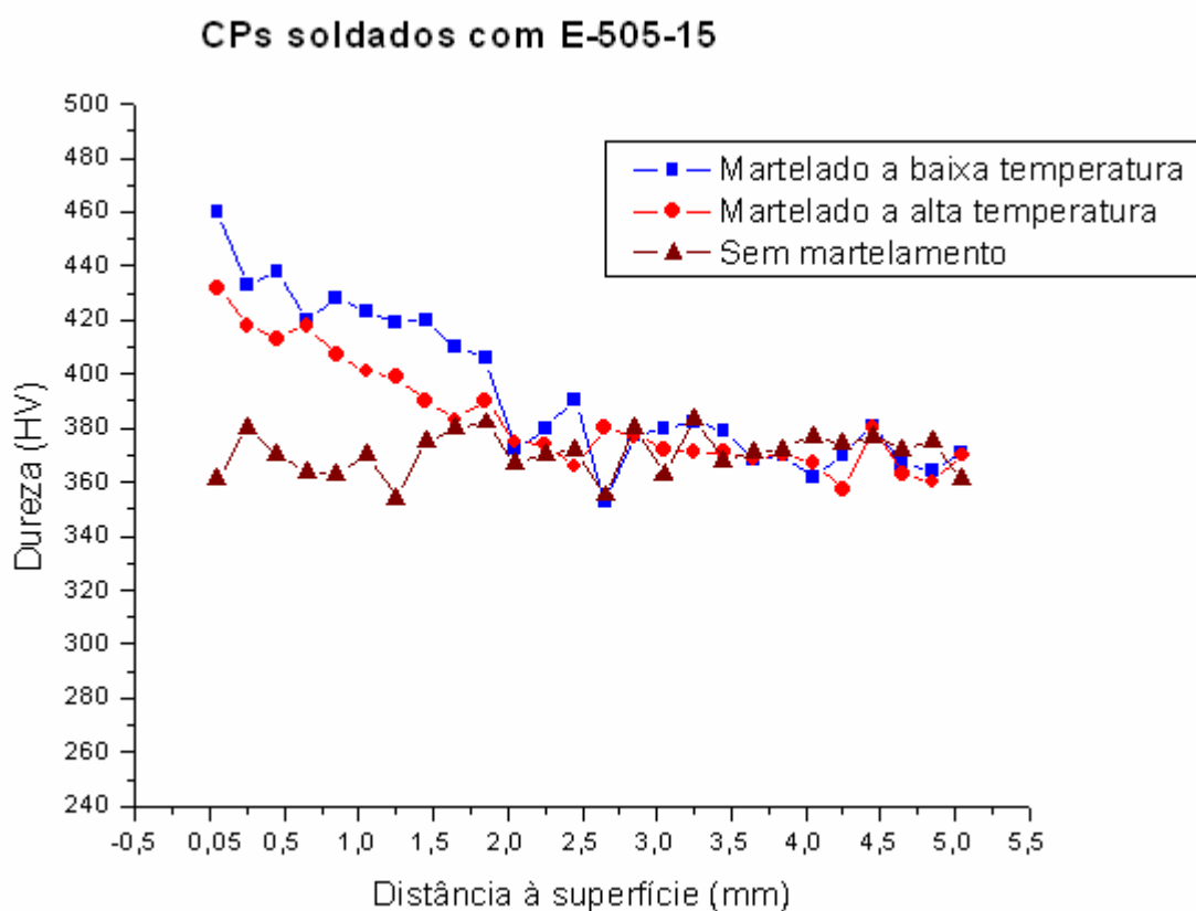
Figura 71 - Valores das microdurezas realizadas nos CPs E-505-15.
