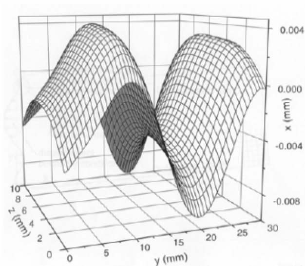
Figura 11 – Exemplo de uma superfície curva, obtida pelo medidor de coordenadas [12].
