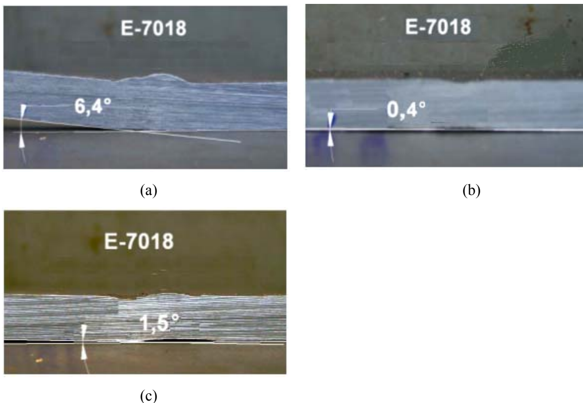
Figura 40 – Distorção angular dos corpos de provas devido às tensões geradas na soldagem, em CPs soldados com eletrodo E-7018; (a) Sem martelar; (b) Martelado a alta temperatura; (c) Martelado a baixa temperatura.
