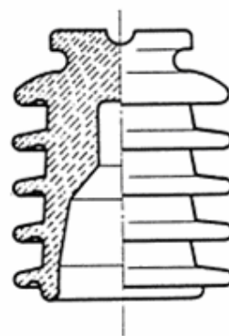
Figura 2 – Isolador elétrico para névoa (Gomes, 2005)
