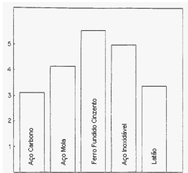
Figura 2.26 – Fatores de aumento da vida de brocas para a usinagem de diversos materiais obtidos através da comparação entre a vida de ferramentas sem a aplicação de revestimentos e ferramentas revestidas com TiN (STRAFFORD, 1996).
