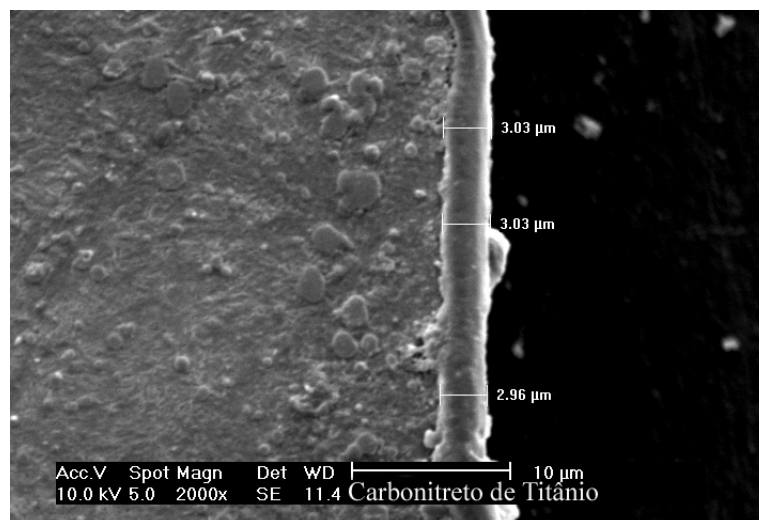
Figura 4.6 – Micrografia da camada limite da matriz de recorte com revestimento de carbonitreto de titânio.
