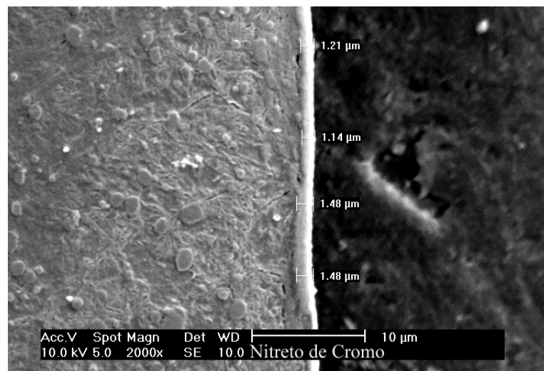
Figura 4.7 – Micrografia da camada limite da matriz de recorte com revestimento de nitreto de cromo.
