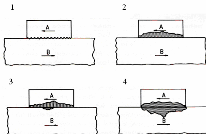
Figura 2.20 – Ruptura das junções por adesão: (1)Na interface; (2)No material A, de resistência mais baixa; (3)Predominantemente no material A, de resistência mais baixa, mas também no material B e (4)Em partes iguais, nos materiais A e B (ZUM GAHR, 1987).
