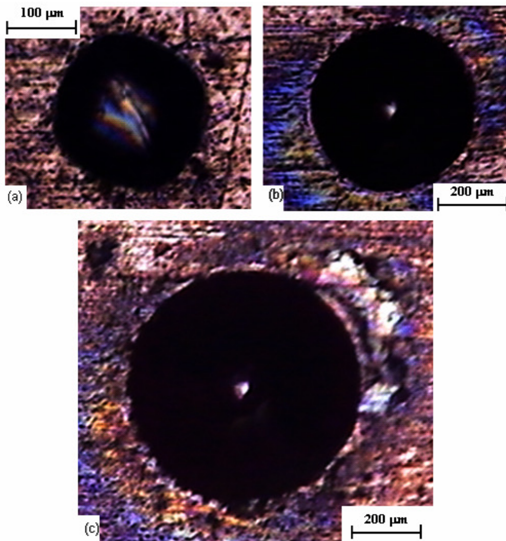
Figura 4.5 – Micrografias das indentações realizadas nos corpos de prova revestidos com carbonitreto de titânio: (a)15 kgf (100x), (b)30 kgf (50x) e (c)45 kgf (50x).
