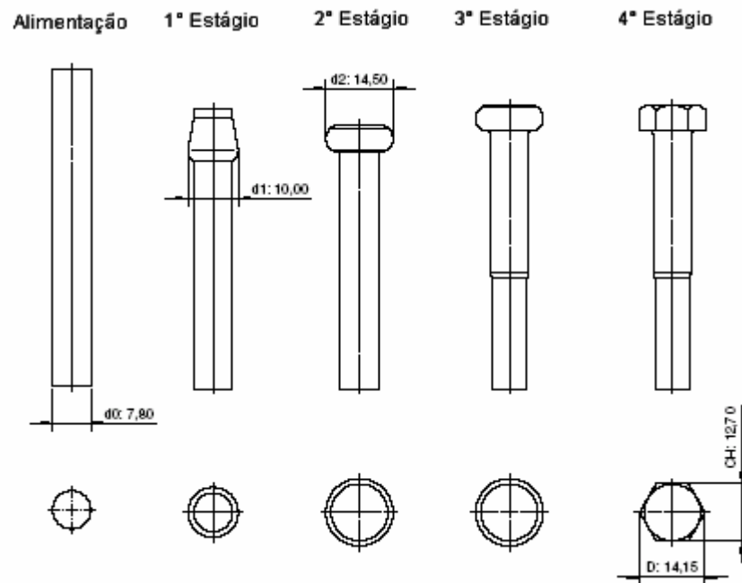
Figura 8.1 – Representação esquemática da seqüência de conformação de um parafuso sextavado (PADRÃO DE PRODUÇÃO 547/2, 2005).
