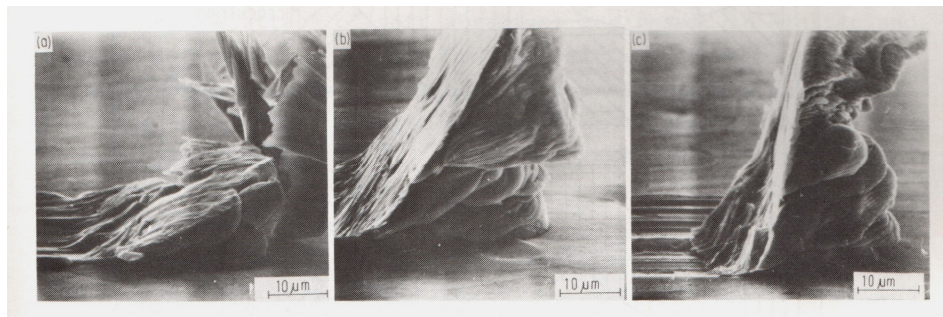
Figura 2.15 – Micrografias de ferro Armco com diferentes ângulos de ataque da partícula abrasiva: (a)30°; (b)60° e (c)90° (ZUM GAHR, 1987).
