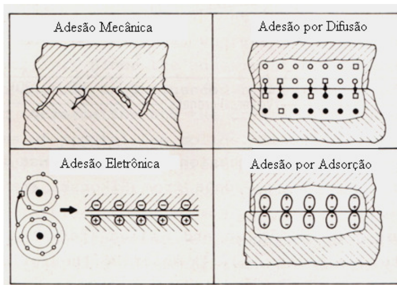
Figura 2.22 – Representação esquemática dos mecanismos de adesão, segundo Kinloch (1980).
