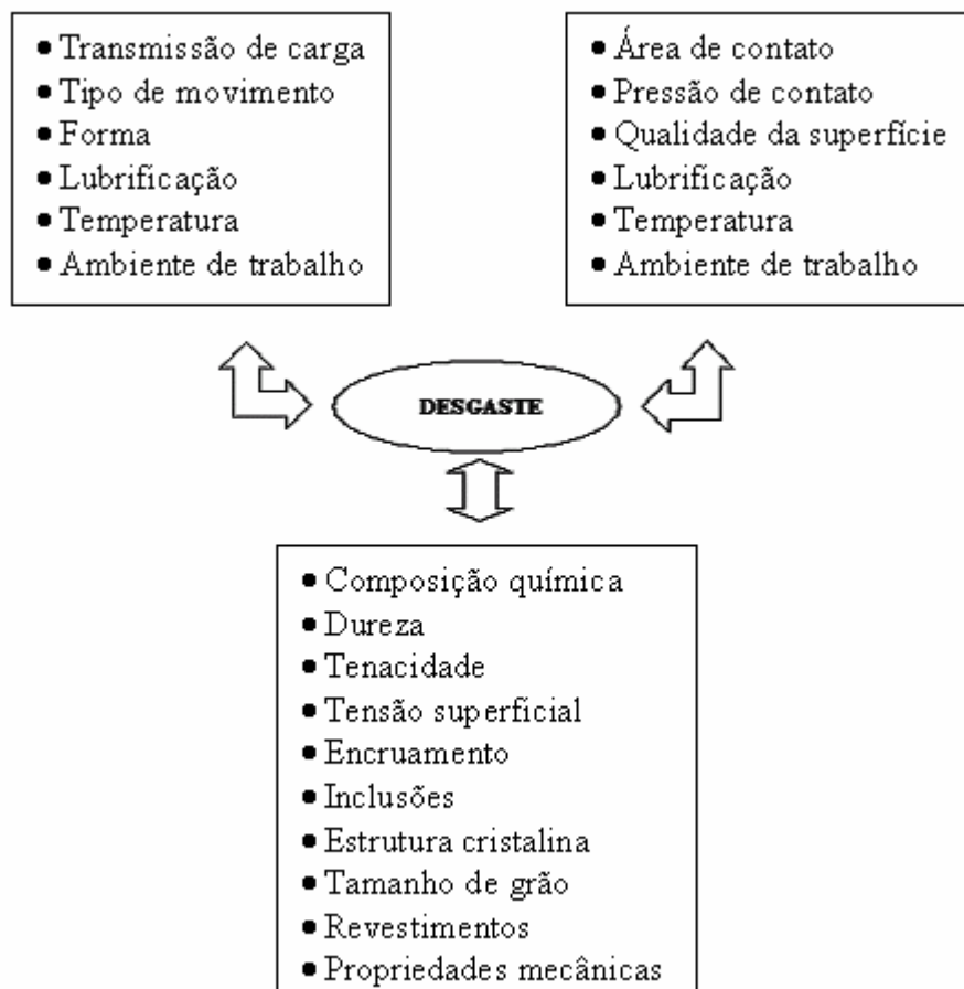
Figura 2.4 – Parâmetros tribológicos que afetam o desgaste (DE MELLO, 1994).
