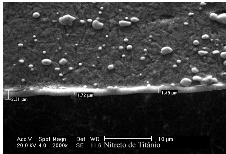
Figura 4.8 – Micrografia da camada limite da matriz de recorte com revestimento de nitreto de titânio.
