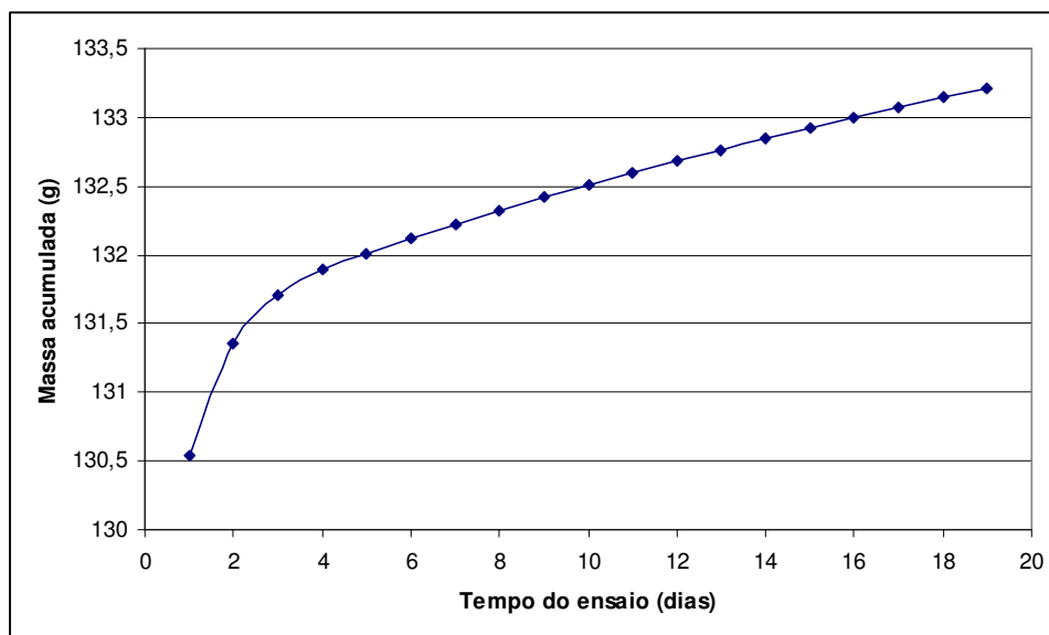
Figura 35 – Evolução do fluxo de umidade acumulativo.
