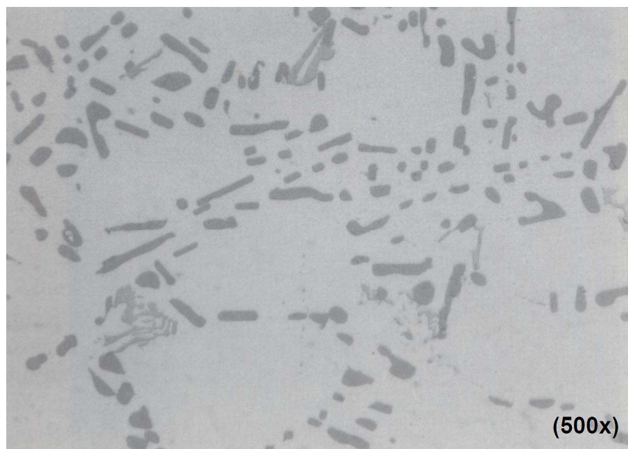
Figura 2.37: Partículas de Si esferoidizadas após o aquecimento durante 8 h a 540 °C (APELIAN; SHIVKUMAR; SIGWORTH, 1989).
