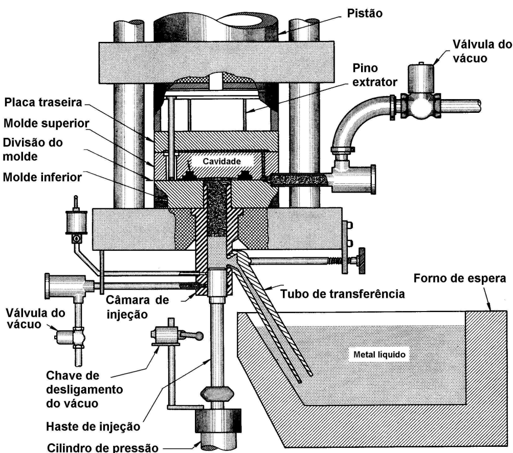
Figura 2.29: Esquema da máquina de fundição sob pressão com câmara fria vertical e molde com linha de partição horizontal (ASM HANDBOOK CASTING, 1970).
