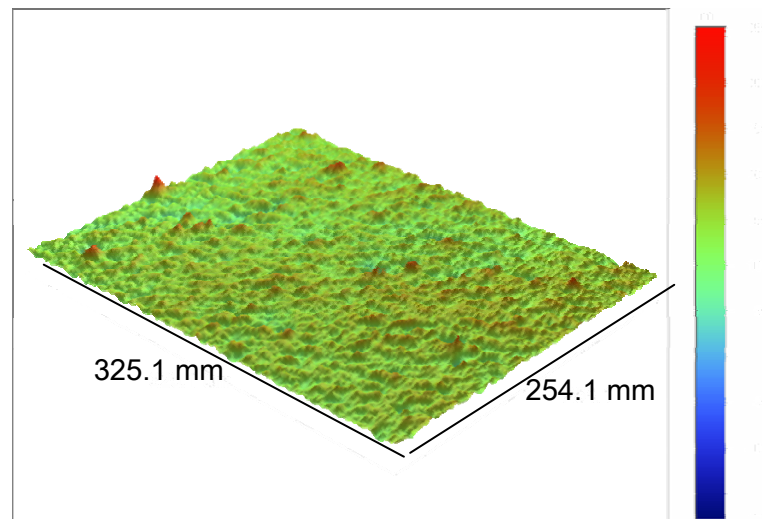
Figura 3.1 – Topografia de uma amostra lixada e polida obtida por interferometria ótica.
