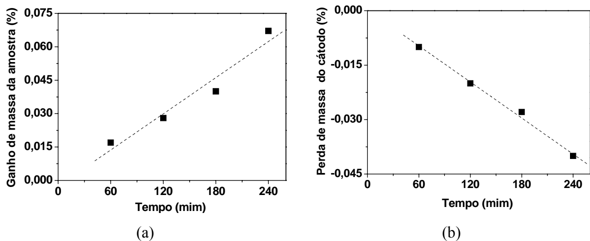
Figura 4.26 – (a) Ganho de massa da amostra; (b) Perda de massa do cátodo, em função do tempo de sulfetação.
