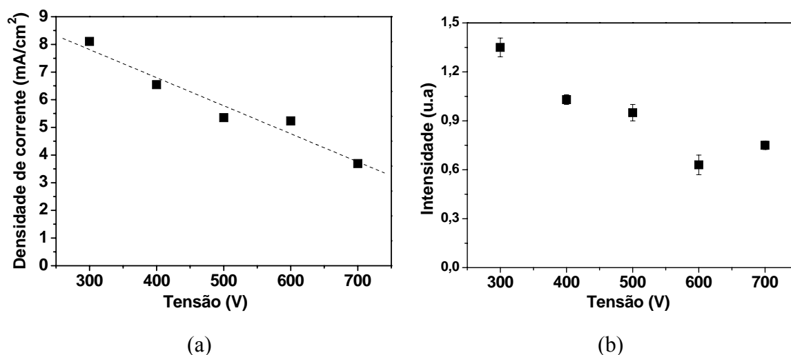
Figura 4.13 – (a) Densidade de corrente necessária para se atingir a temperatura de 500 °C nas tensões correspondentes; (b) intensidade do pico (S* 391 nm) versus tensão.
