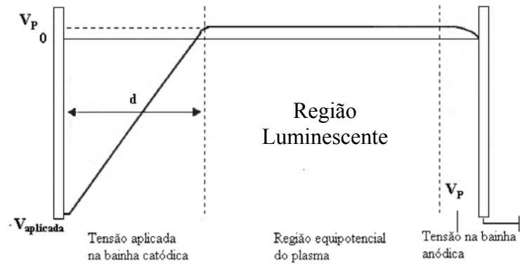
Figura 2.4 – Regiões de interesse no plasma e distribuição de potencial entre os eletrodos numa descarga luminescente anormal [9].
