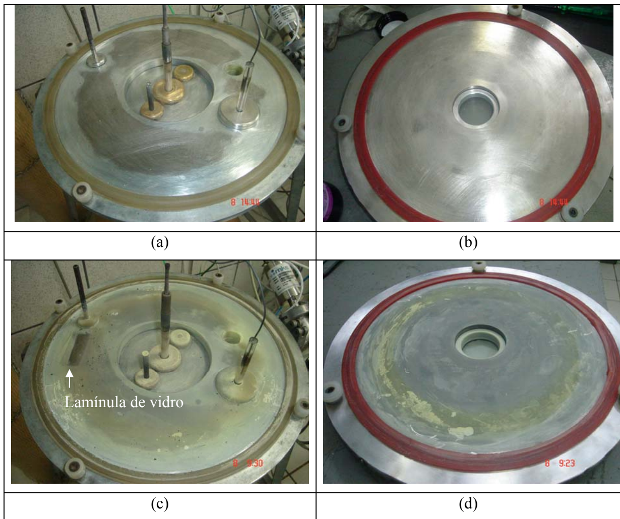
Figura 4.31 – Fotos do reator desmontado, base (a) e tampa (b) antes do ciclo de sulfetação, base (c) e tampa (d) após ciclo de sulfetação.
