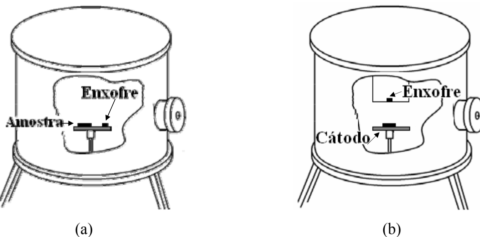
Figura 3.7 – Desenho esquemático da posição do enxofre no interior do reator.
