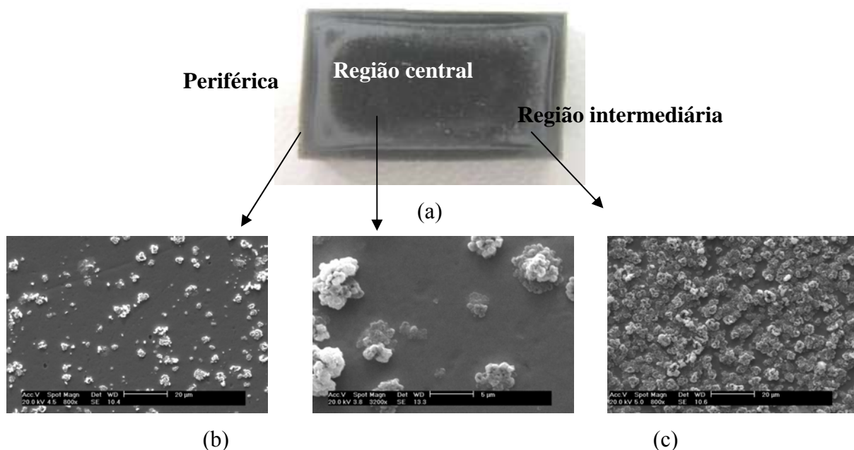
Figura 4.6 – Aspecto visual da amostras sulfetadas no cátodo (a), micrografias das superfícies nas região (b) intermediária (3200x) e periférica (800x) e (c) centro (800x).
