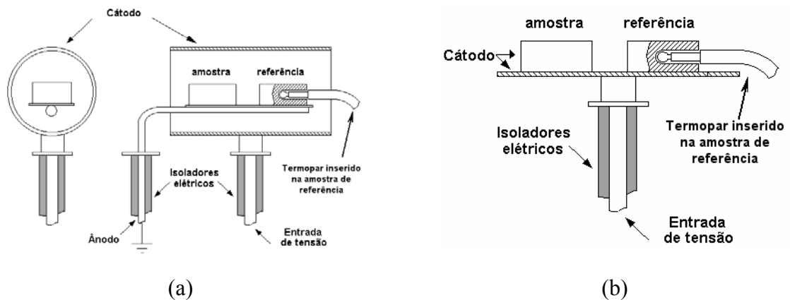
Figura 3.4 – Desenho esquemático dos eletrodos na configuração (a) ânodo-cátodo confinado e (b) cátodo plano.
