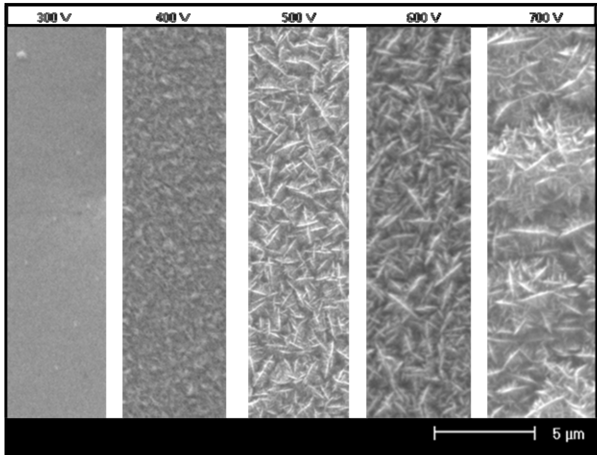
Figura 4.16 – Morfologia da camada das amostras sulfetadas variando a tensão.
