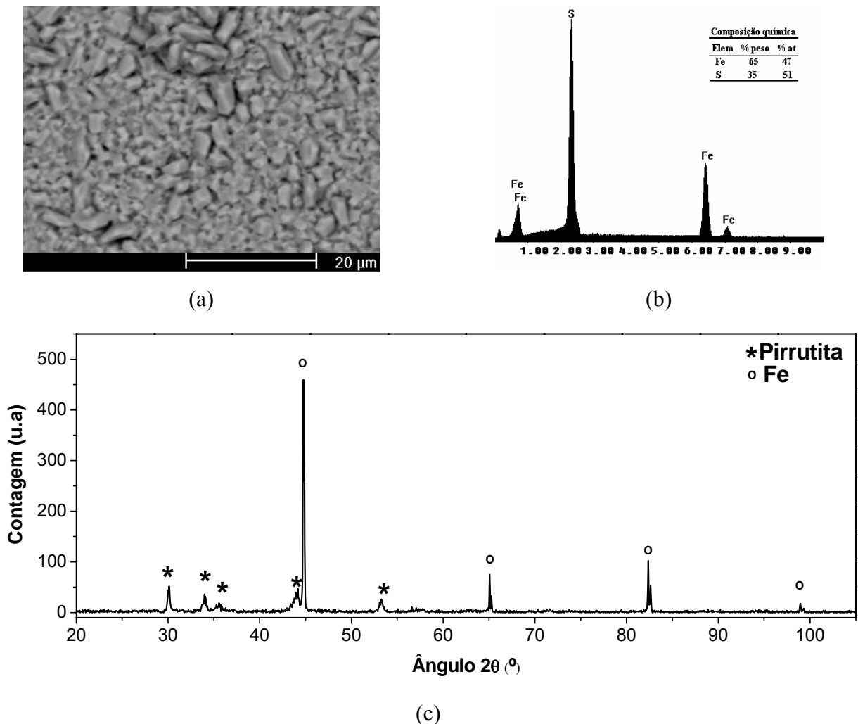
Figura 4.4 – Morfologia de superfície (a), análise química (b) e espectros de raios X, do cátodo de ferro após sulfetação.
