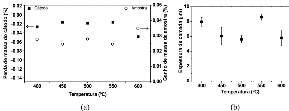
Figura 4.18 – Variação de massa do cátodo e amostra (a) e espessura da camada, em função da temperatura de sulfetação.
