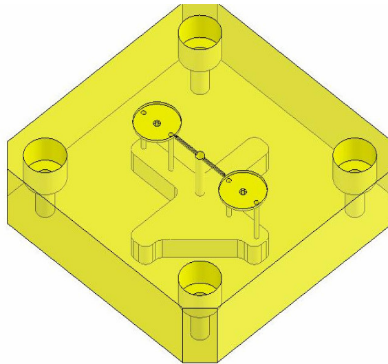
Figura 15 – Molde projetado para execução do trabalho.
