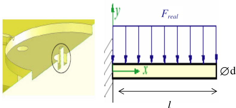
Figura 16 - Pino localizado no centro da cavidade, e perfil de carregamento em função da posição do canal de injeção.
