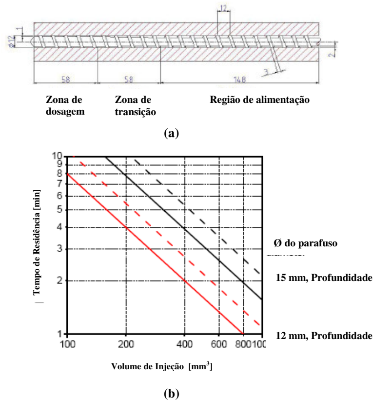
Figura 7 – Unidade de plastificação de uma micro-injetora (a). Tempo de permanência pelo volume do shot assumindo um ciclo de 10s (b) [37].
