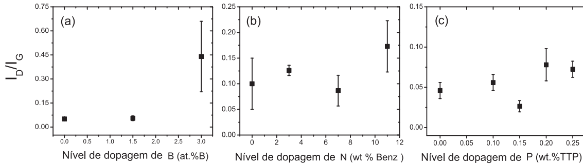
Fig. 4.3: Razão I_D/I_G para amostras dopadas com diferentes concentrações de (a) B, (b) N e (c) P no precursor, medidas com E_{laser}=2.41 \text{ eV} e potência de 0.2 mW. Os valores de I_D/I_G são a média de medidas feitas em diferentes locais da amostra.
