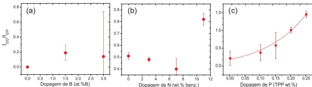
Fig. 6.10: Relações I_{G'_D}/I_{G'_P} para amostras dopadas com (a) B, (b) N e (c) P, medidas com E_{laser} = 2.41 eV, 0.2 mW.
