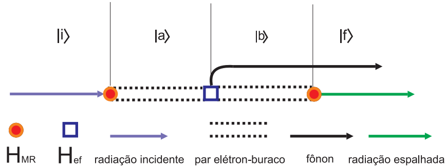
Fig. 3.1: Diagrama de Feynman associado a um processo Raman Stokes .
