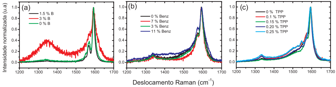
Fig. 4.2: Bandas G e D medidas com E_{Laser} = 2.41 \text{ eV} , com potência de 0.2 mW, para amostras dopadas com (a) B, (b) N e (c) P.
