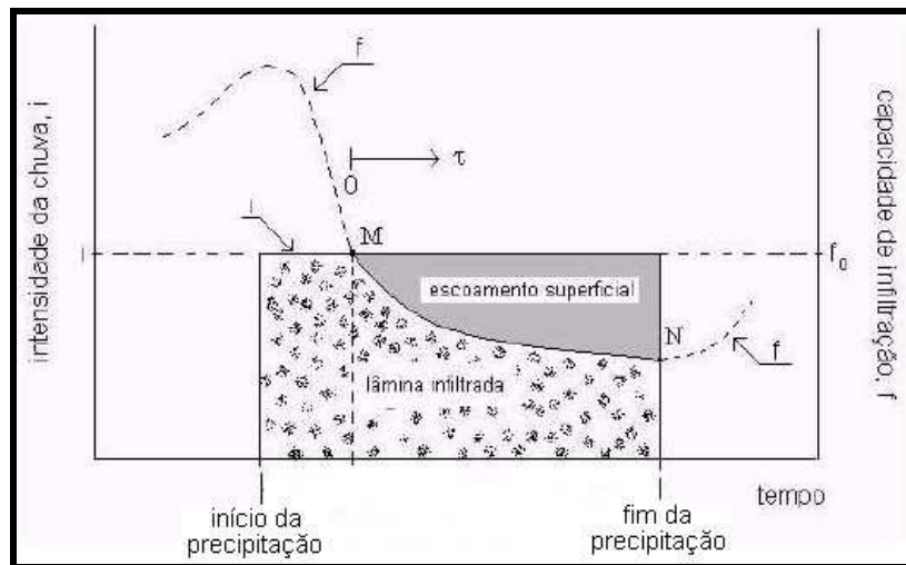
Figura 4. 8 – Variação de capacidade de infiltração durante uma precipitação (Barbosa Jr., 2002).
