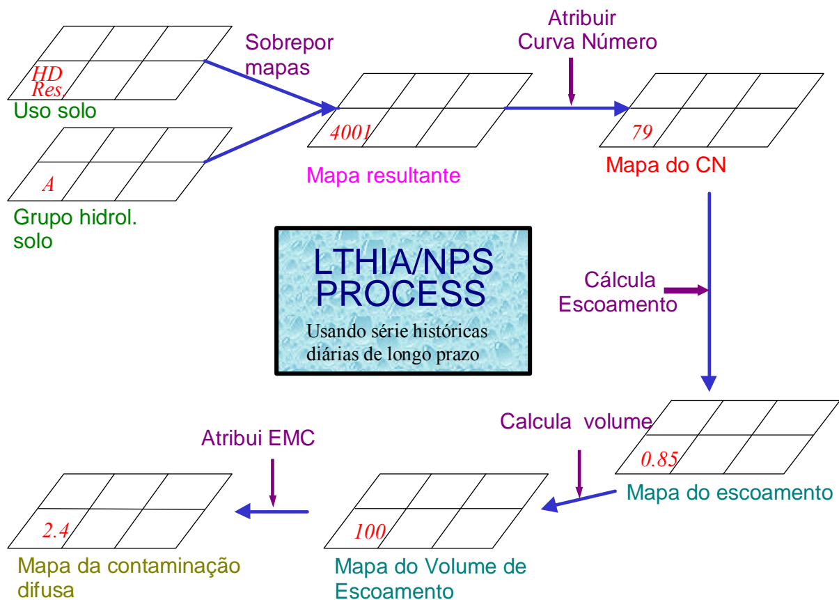
Figura 4.1 - Fluxograma modelo L-THIA (modificado-acesso internet 23/03/2007:
