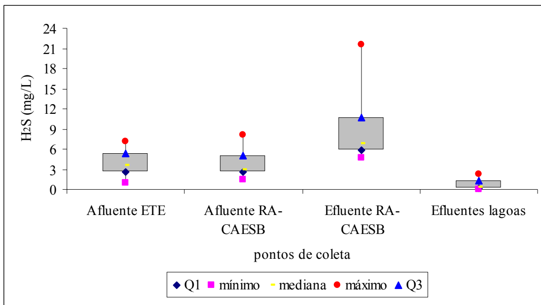
Figura 5.14 - Concentração de sulfeto de hidrogênio nos pontos de coleta na ETE Paranoá no período da manhã.
