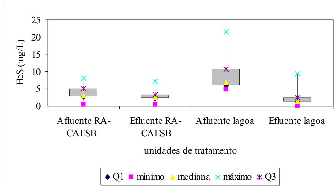
Figura 5.17 - Concentração de H_2S no afluyente (observada) e no efluente (predita pelo modelo WATER9) no RA - CAESB e na lagoa no período da manhã.
