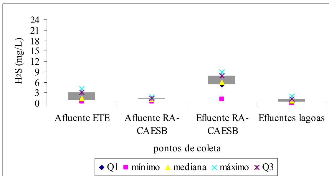
Figura 5.15 - Concentração de sulfeto de hidrogênio nos pontos de coleta na ETE – Paranoá no período da noite.
