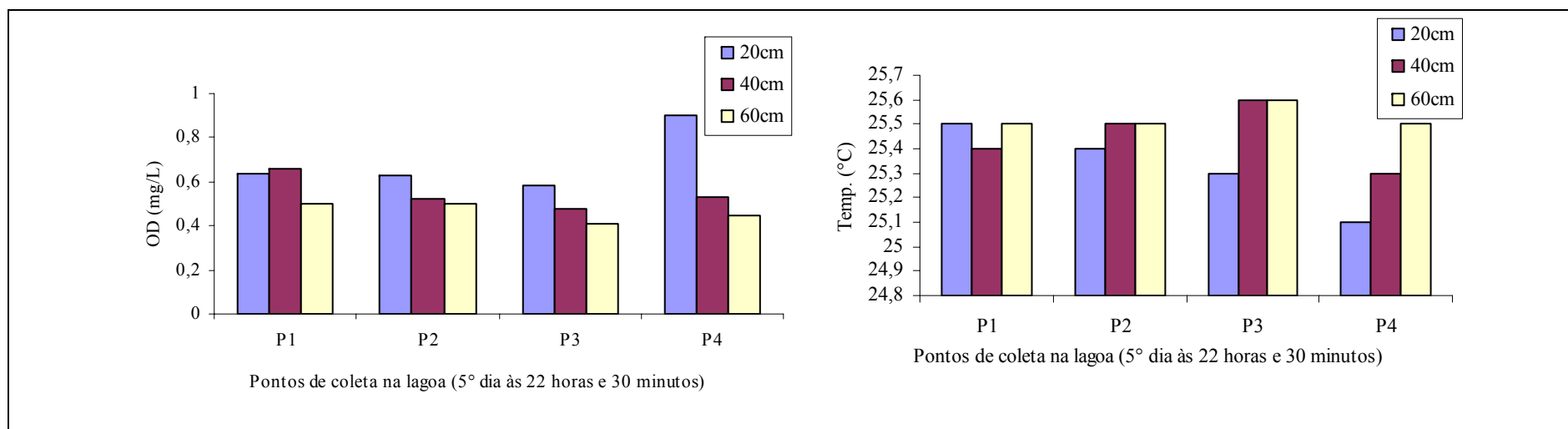
Figura 5.30 - Perfil de temperatura e OD nos pontos de coleta na lagoa no 5º dia.
