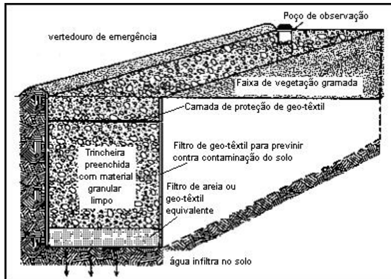
Figura 3.10 – Esquema de uma trincheira de infiltração (Souza, 2002).
