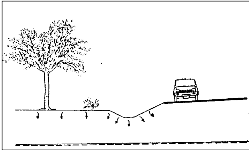
Figura 3.12 – Perfil de uma vala de infiltração (Urbonas e Stahre, 1993).
