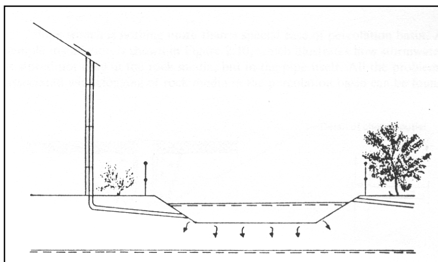
Figura 3.1 – Representação de uma Bacia de Infiltração (Urbonas e Stahre, 1993).
