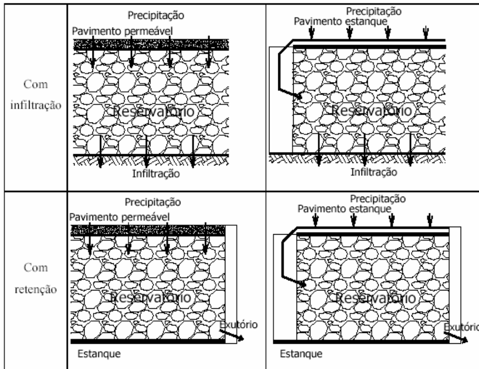
Figura 3.4. – Arranjos de pavimentos com estrutura de reservação (Azzout et al. 1994)
