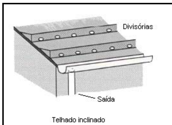
Figura 3.9 – Esquema de telhado armazenador inclinado (CETE DU SUD-OUEST, 2003)
