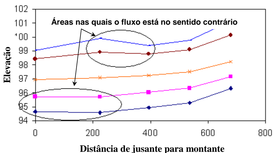
Figura A.2 - gráfico dos perfis longitudinais da elevação da superfície da água para seções transversais adjacente.
