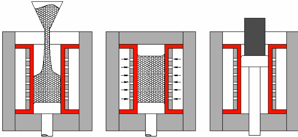
Figura 2.16 – Esquema do processo de prensagem isostática dry bag ou fixed bag . Da esquerda para a direita, as etapas de alimentação do molde, prensagem e extração do compactado (REED, 1995).
