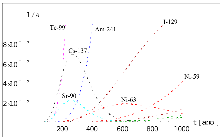
Figura 5.33 – Risco para a primeira infância para todos os radionuclídeos. Visão detalhada da Figura 5.31.
