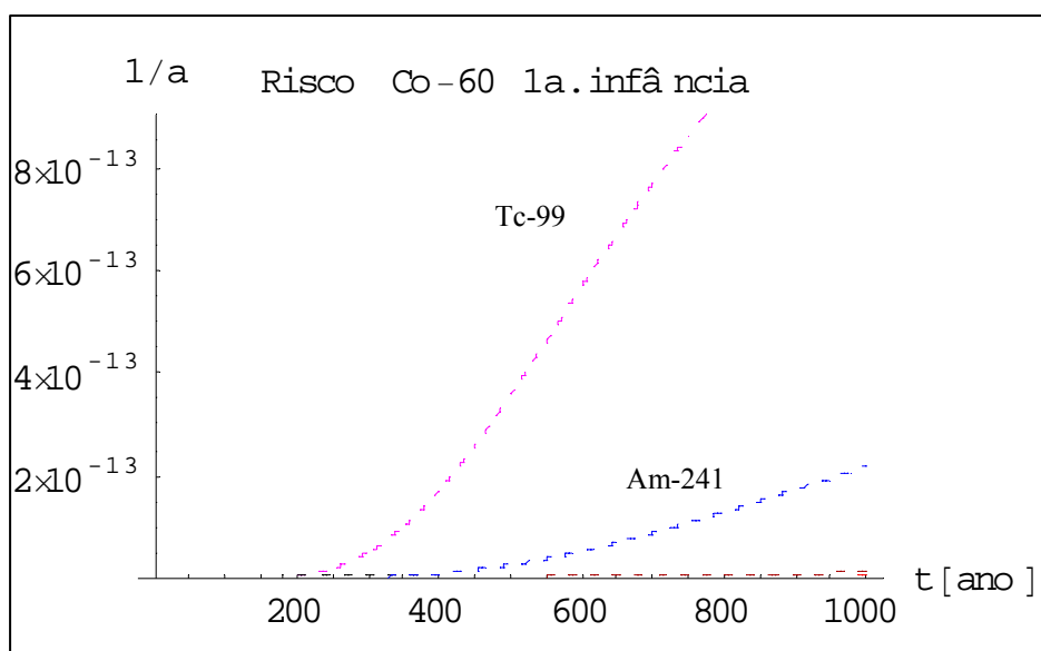
Figura C.15 – Risco de câncer fatal para a primeira infância para cada radionuclídeo.
