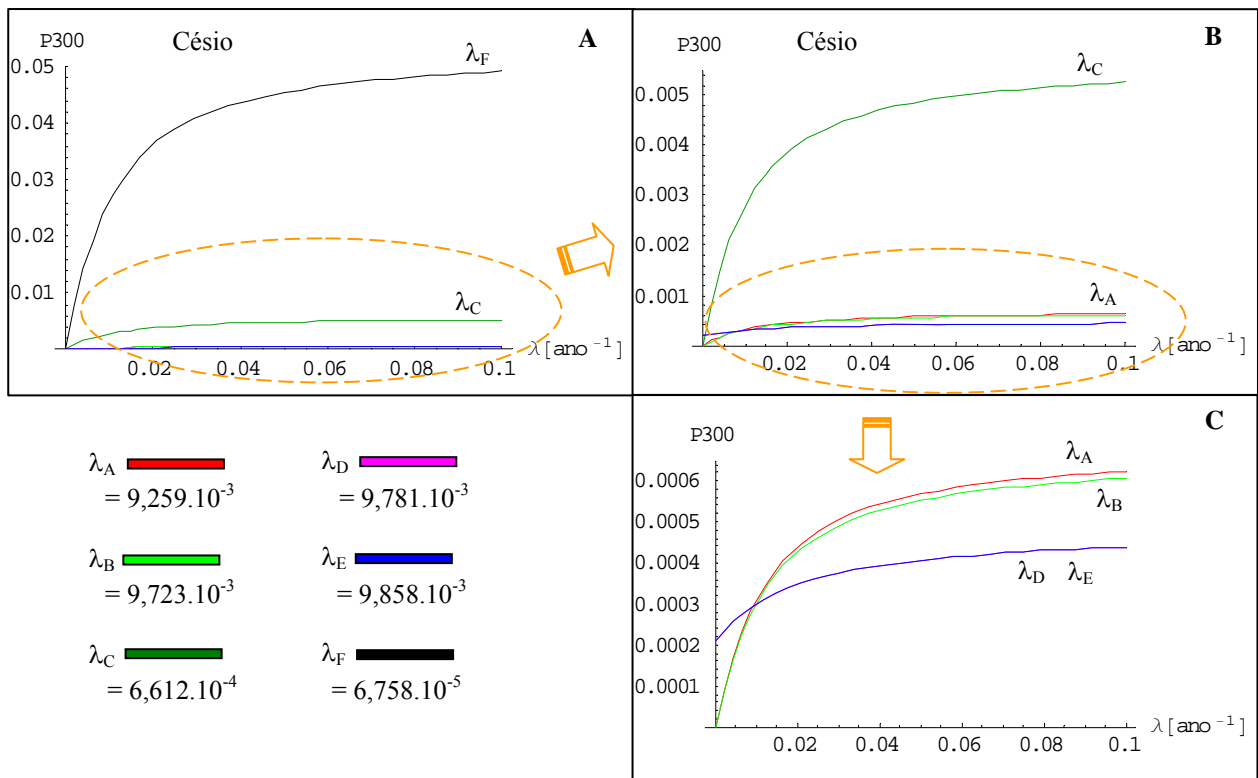
Figura 5.11 – Comportamento da probabilidade em 300 anos com a variação de uma única taxa de falha por vez para o Césio.
