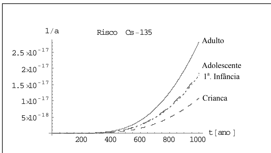
Figura C.7 – Risco de câncer fatal para o Cs-135 para cada faixa etária do grupo crítico.
