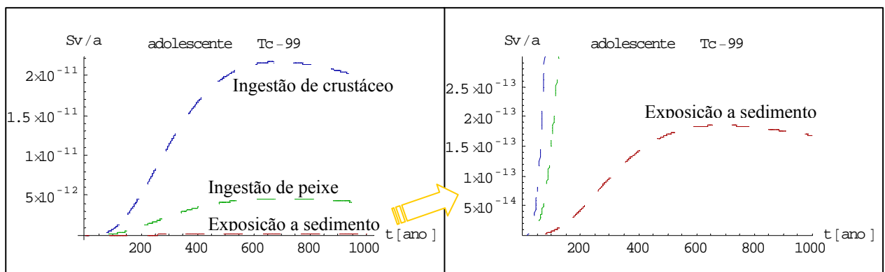
Figura 5.23 – Taxas de dose efetiva devido à ingestão do alimento (peixe e crustáceo) e ao contato com sedimentos de praia contaminados de Tc-99 para adolescente.
