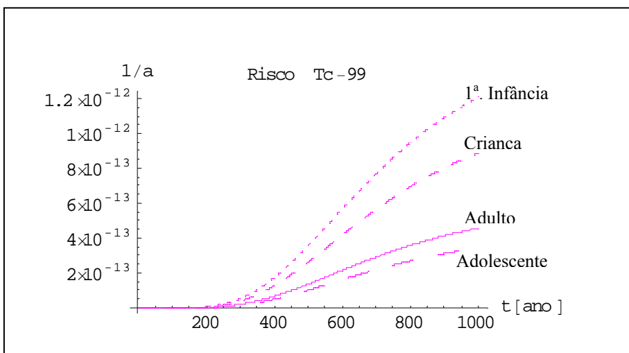
Figura C.5 – Risco de câncer fatal para o Tc-99 para cada faixa etária do grupo crítico.
