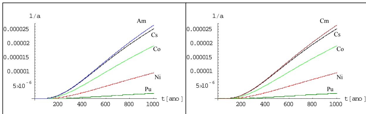
Figura 5.15 – Função densidade de probabilidade por grupos de radionuclídeos, excetuando os três radionuclídeos com maiores probabilidades de falha.
