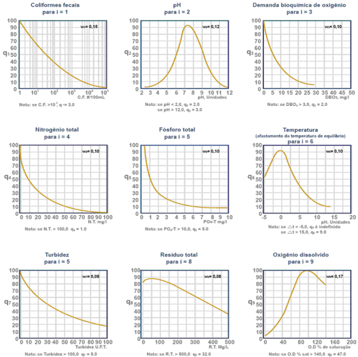
Figura 1. Curvas para o cálculo do Índice de Qualidade de Água (IQA) para coliformes fecais, pH, demanda bioquímica de oxigênio (DBO 5 ), nitrogênio total, fósforo total, temperatura, turbidez, resíduo total e oxigênio dissolvido (ANA, 2005).
