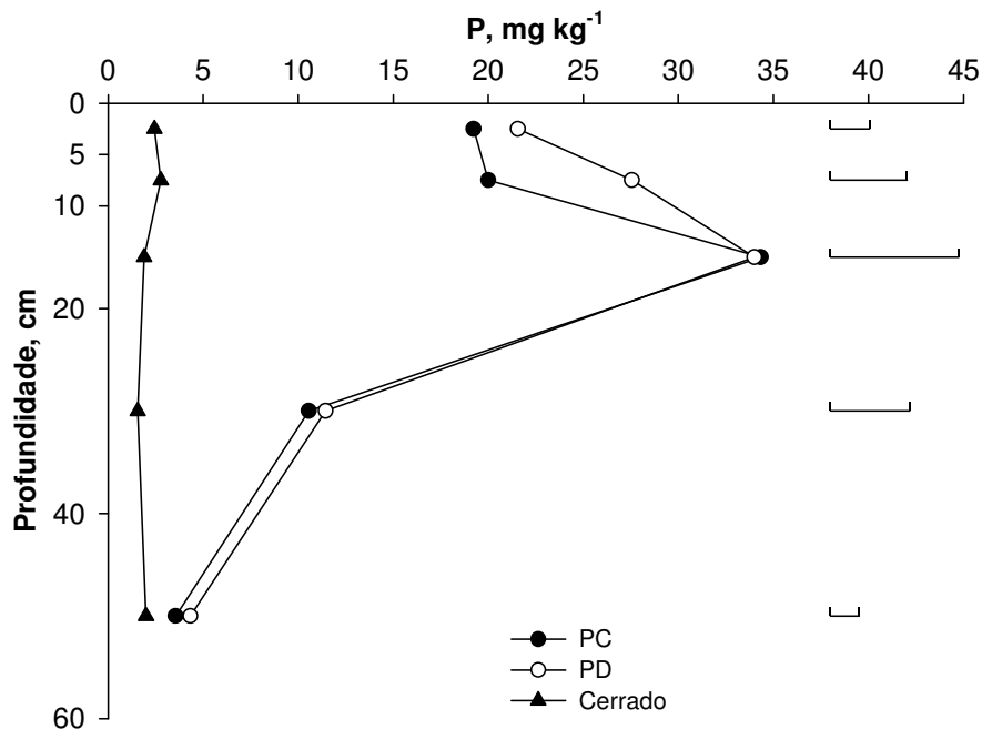
FIGURA 31. Teores de fósforo disponível no perfil do solo de Cerrado, amostrado em 2005, sob diferentes manejos (PC= preparo convencional e PD= plantio direto) e vegetação nativa em Tasso Fragoso-MA. Barras horizontais representam a diferença mínima significativa (Teste DMS 5%).
