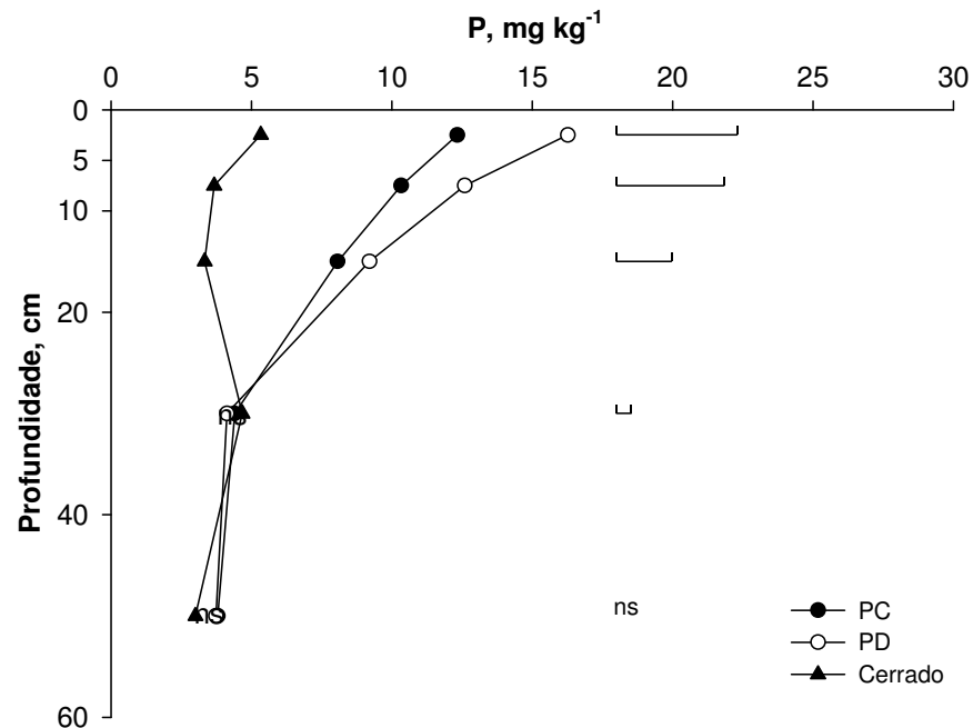
FIGURA 29. Teores de fósforo disponível no perfil do solo de Cerrado, amostrado em 2005, sob diferentes manejos (PC= preparo convencional e PD= plantio direto) e vegetação nativa em Costa Rica-MS. Barras horizontais representam a diferença mínima significativa (Teste DMS 5%). ns= não significativo.
