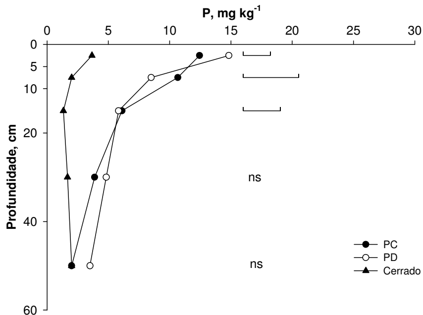
FIGURA 27. Teores de fósforo disponível no perfil do solo de Cerrado, amostrado em 2005, sob diferentes manejos (PC= preparo convencional e PD= plantio direto) e vegetação nativa em Luziânia-GO. Barras horizontais representam a diferença mínima significativa (Teste DMS 5%). ns= não significativo.
