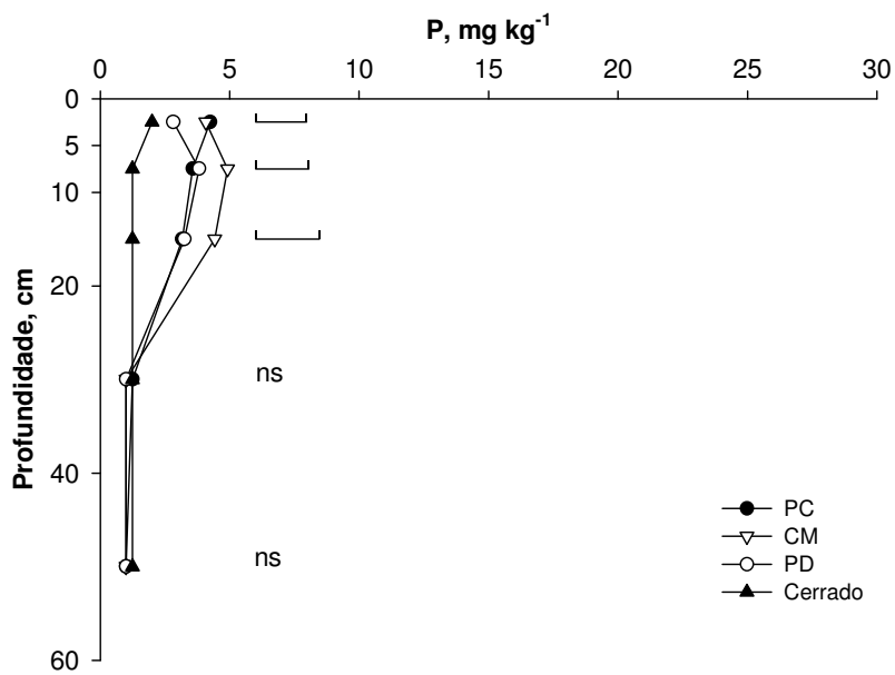
FIGURA 33. Teores de fósforo disponível no perfil do solo de Cerrado, amostrado em 2005, sob diferentes manejos (PC= preparo convencional, CM= cultivo mínimo e PD= plântio direto) e vegetação nativa em Sapezal-MT. Barras horizontais representam a diferença mínima significativa (Teste DMS 5%). ns= não significativo.
