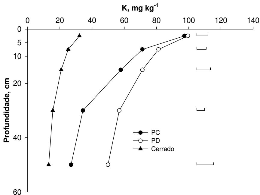
FIGURA 32. Teores de potássio disponível no perfil do solo de Cerrado, amostrado em 2005, sob diferentes manejos (PC= preparo convencional e PD= plantio direto) e vegetação nativa em Tasso Fragoso-MA. Barras horizontais representam a diferença mínima significativa (Teste DMS 5%).
