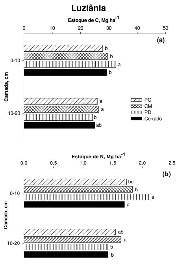
FIGURA 9. Estoques de carbono (a e c) e nitrogênio (b e d) do solo, avaliados em 2005, nos experimentos de Luziânia e Costa Rica. Barras seguidas da mesma letra dentro da mesma camada, não se diferenciam entre si pelo Teste DMS 5%. ns= não significativo.
