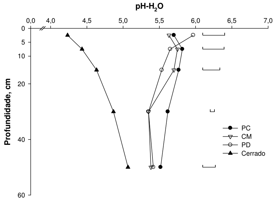
FIGURA 21. Valores de pH-H 2 O no perfil do solo de Cerrado, amostrado em 2005, sob diferentes manejos (PC= preparo convencional e PD= plantio direto) e vegetação nativa em Sapezal-MT. Barras horizontais representam a diferença mínima significativa (Teste DMS 5%).
