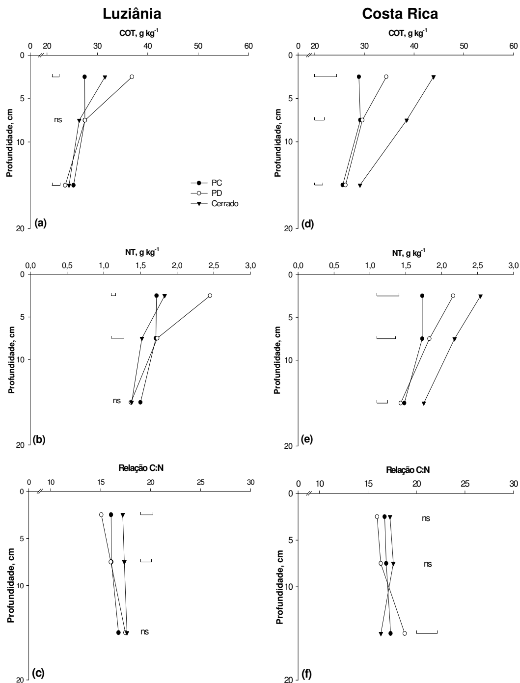
FIGURA 7. Teores de carbono orgânico total (a e d), nitrogênio total (b e e) e relação C:N (c e f) do solo, avaliados em 2005, nos experimentos de Luziânia e Costa Rica. Barras horizontais representam a diferença mínima significativa pelo Teste DMS 5%. ns= não significativo.
