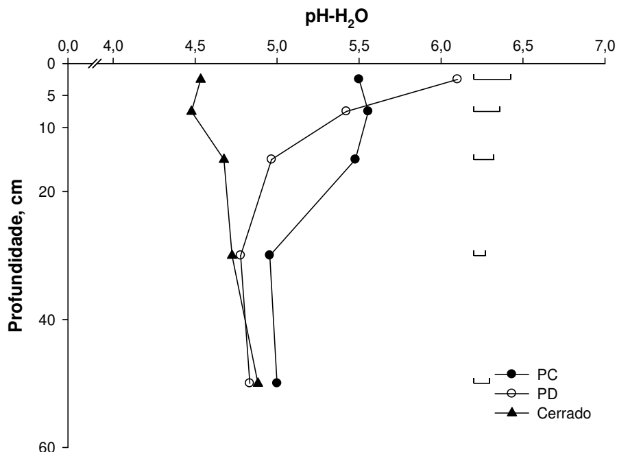
FIGURA 19. Valores de pH-H 2 O no perfil do solo de Cerrado, amostrado em 2005, sob diferentes manejos (PC= preparo convencional e PD= plantio direto) e vegetação nativa em Tasso Fragoso-MA. Barras horizontais representam a diferença mínima significativa (Teste DMS 5%).
