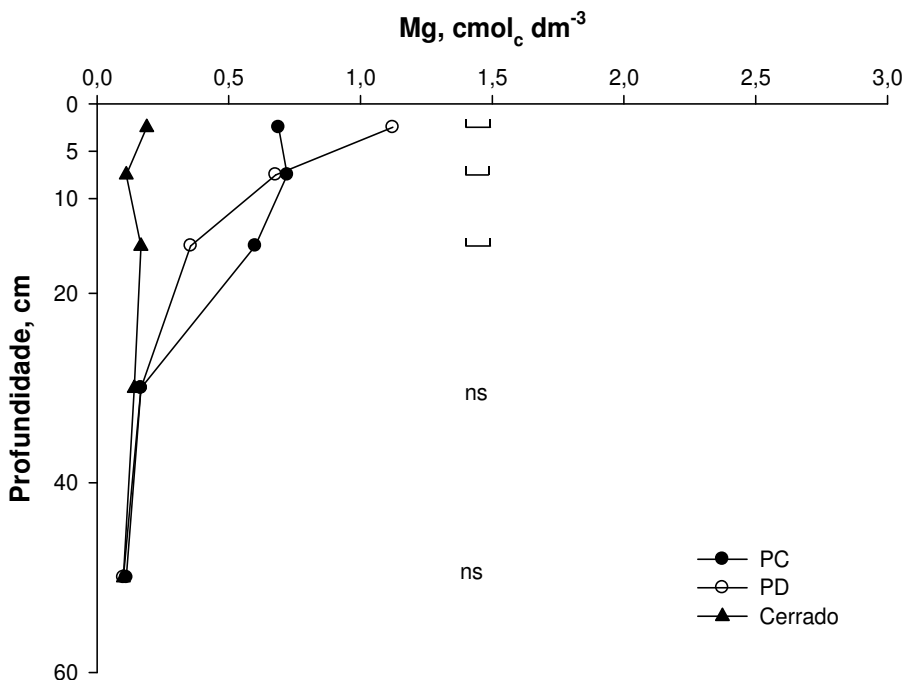
FIGURA 40. Teores de magnésio trocável no perfil do solo de Cerrado, amostrado em 2005, sob diferentes manejos (PC= preparo convencional e PD= plantio direto) e vegetação nativa em Tasso Fragoso-MA. Barras horizontais representam a diferença mínima significativa (Teste DMS 5%). ns= não significativo.
