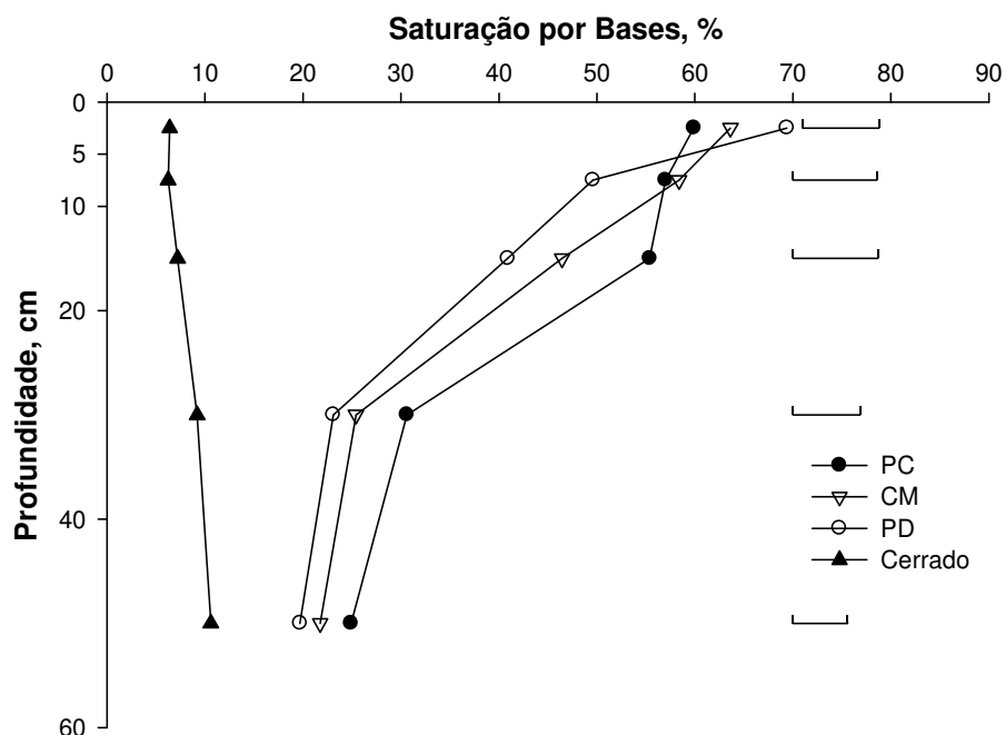
FIGURA 22. Saturação por bases no perfil do solo de Cerrado, amostrado em 2005, sob diferentes manejos (PC= preparo convencional e PD= plantio direto) e vegetação nativa em Sapezal-MT. Barras horizontais representam a diferença mínima significativa (Teste DMS 5%).
