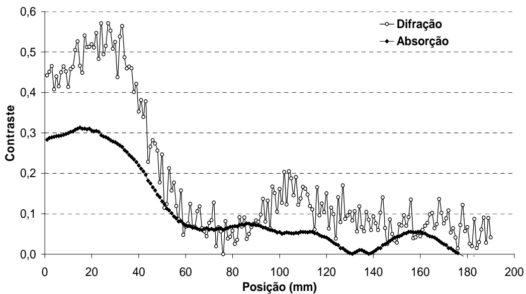
Figura IV.6. Contraste calculado para a varredura por difração e absorção para a amostra 3 (mama com carcinoma).
