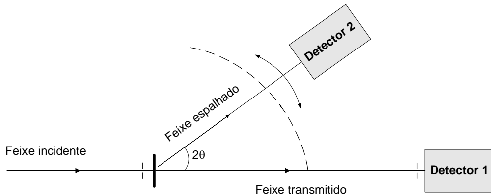
Figura III.4. Esquema experimental da geometria por transmissão para obtenção dos perfis de espalhamento.
