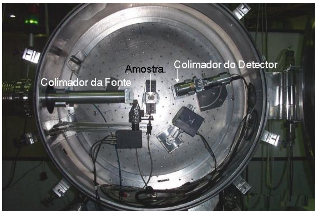
Figura III.6. Arranjo experimental mostrando os componentes.
