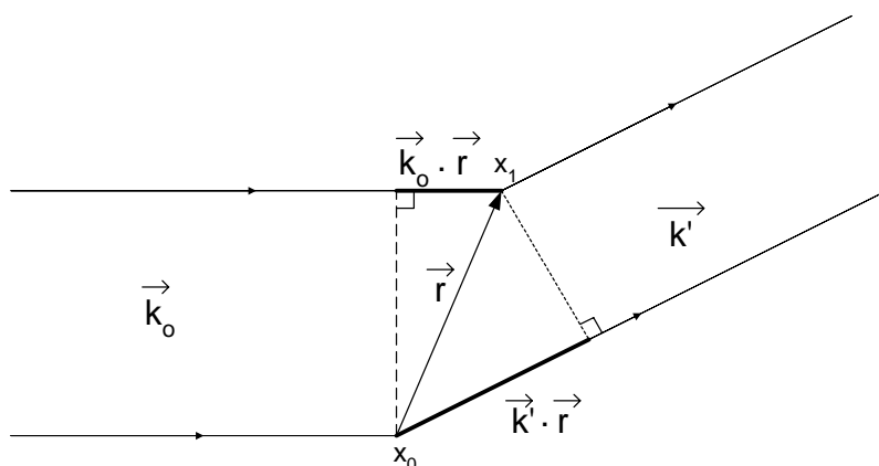
Figura II.8. Diferença de caminhos no espalhamento.
