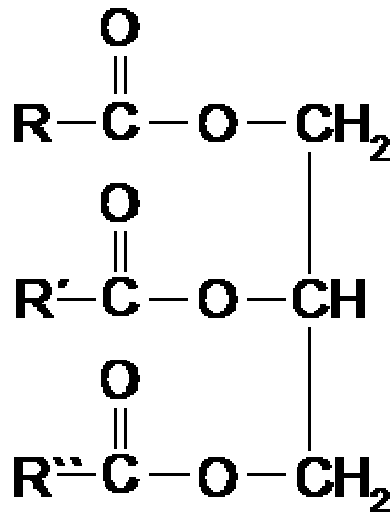
Figura V.2. Representação funcional da molécula de triglicerídeo.
