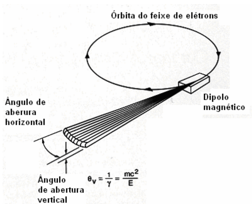
Figura II.13. Geometria laminar (sobre o plano da órbita) de um feixe de luz síncrotron.
