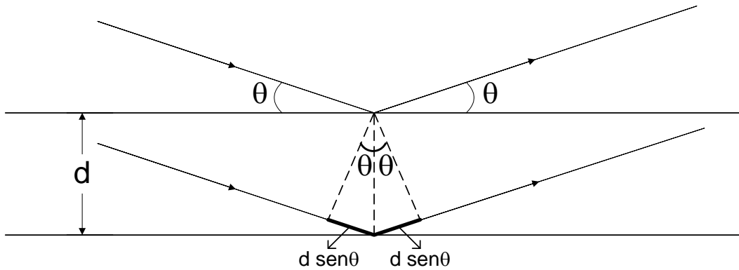
Figura II.5. Lei de Bragg.
