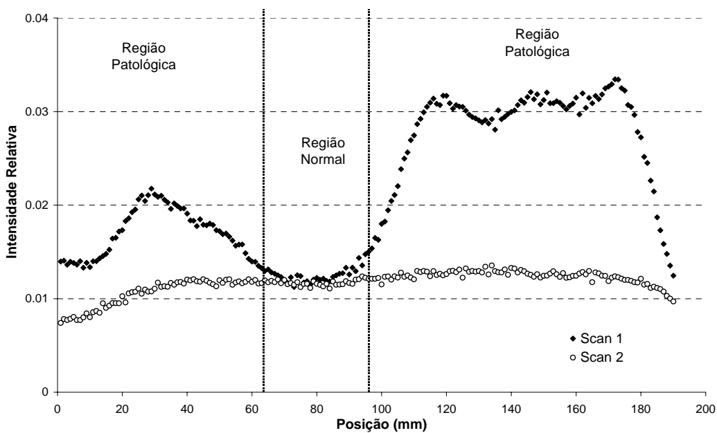
Figura IV.5. Varreduras de difração realizadas com o detector posicionado no ângulo característico para o tuberculoma ( \theta = 22,8^\circ ) para a amostra 4.
