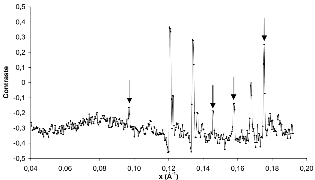
Figura IV.2. Perfil de difração para a amostra 4. As setas indicam as posições das principais reflexões.
