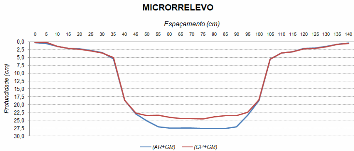
Figura 24. Microrrelevos médios nos tratamentos AR+GM e GP+GM.
