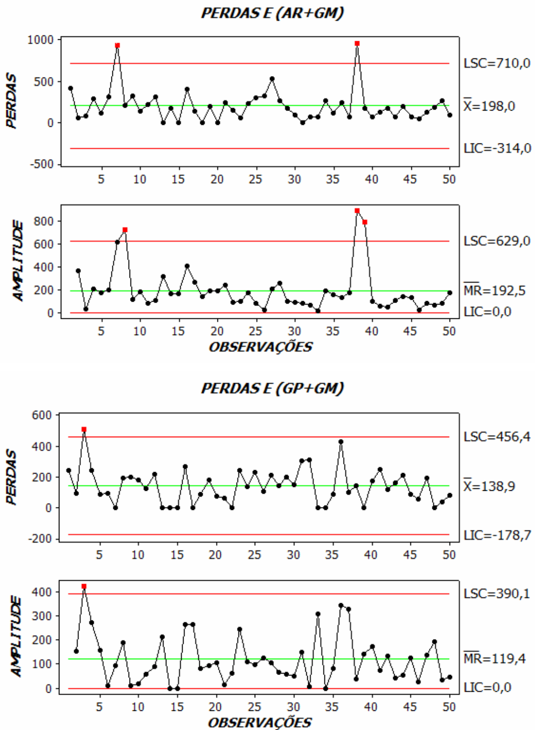
Figura 16. Cartas de controle para perdas de estilhaço ( \text{kg ha}^{-1} ).
