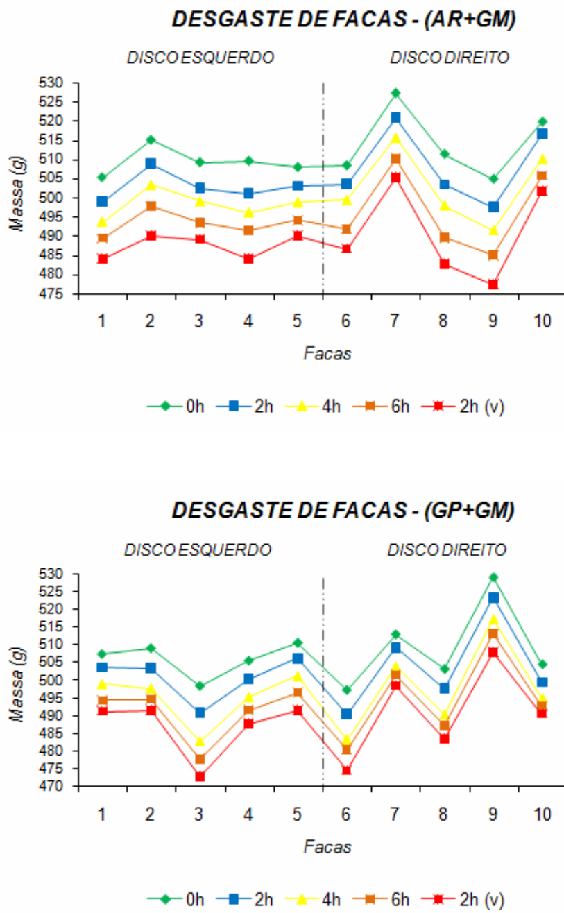
Figura 21. Desgaste das facas do corte basal nos tratamentos AR+GM e GP+GM.
