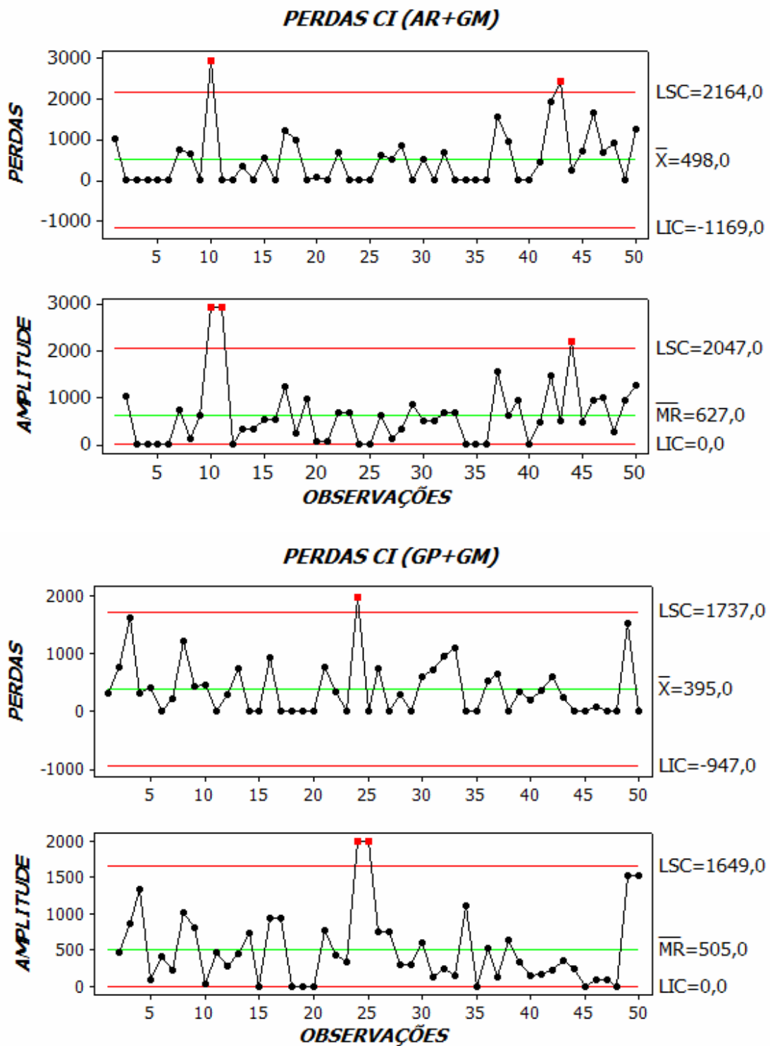
Figura 11. Cartas de controle para perdas de cana inteira ( \text{kg ha}^{-1} ).
