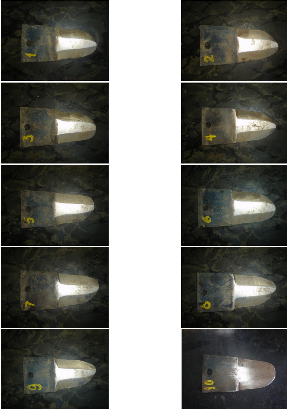
APÊNDICE 2. Facas utilizadas no tratamento AR+GM, em 8h de trabalho.
