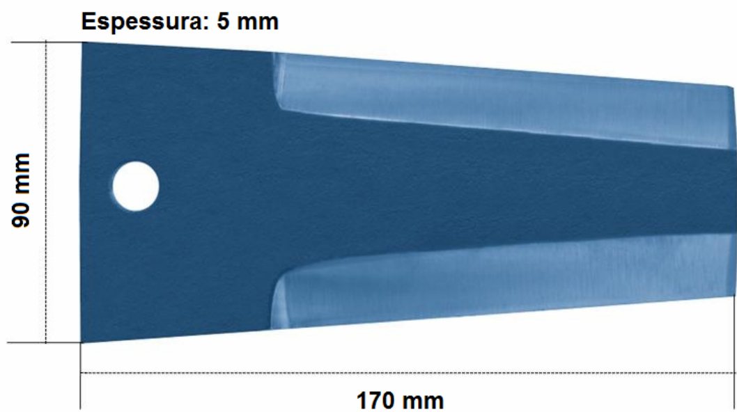
Figura 7. Faca do corte de base.
