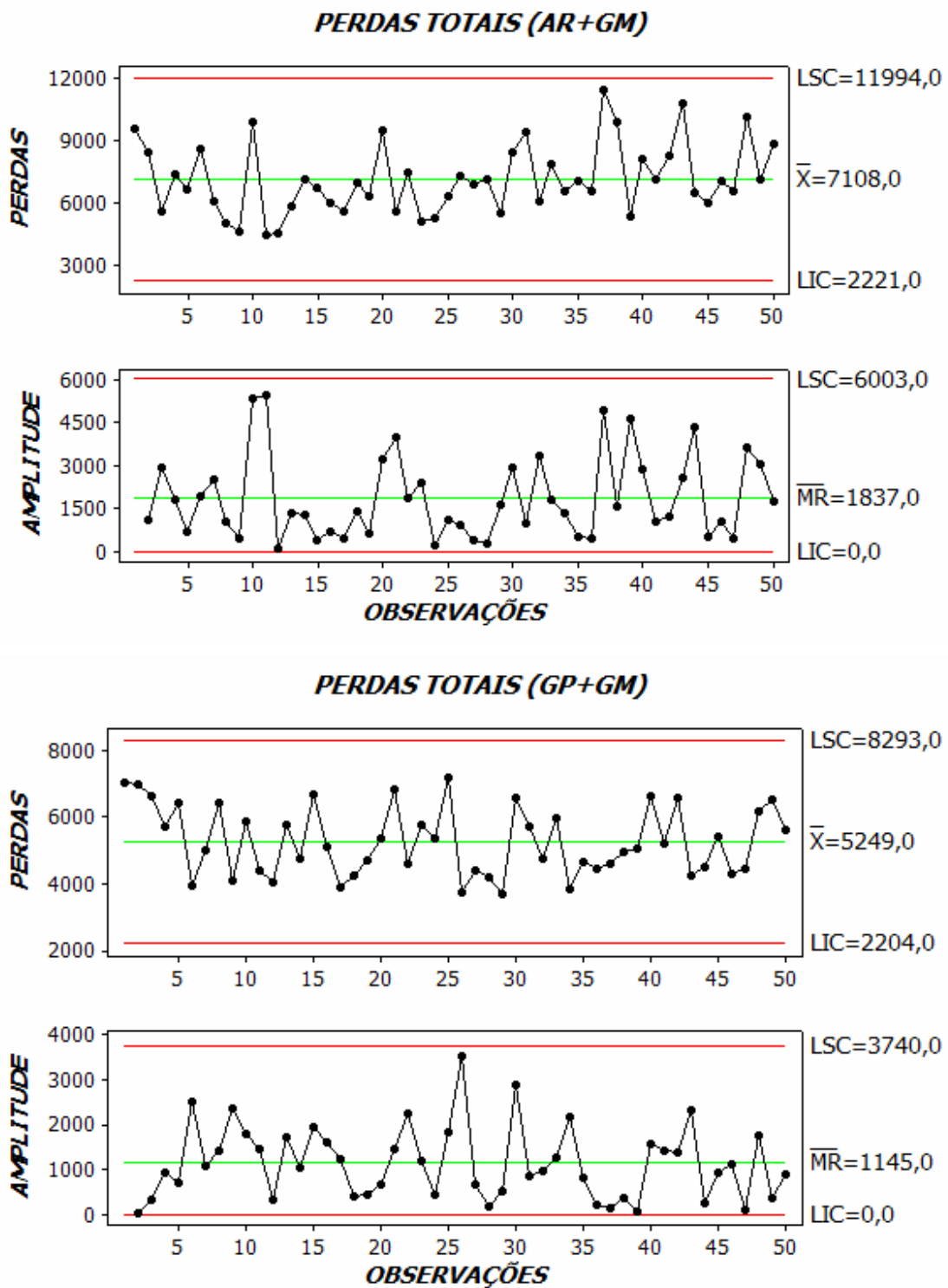
Figura 18. Cartas de controle para perdas totais ( \text{kg ha}^{-1} ).
