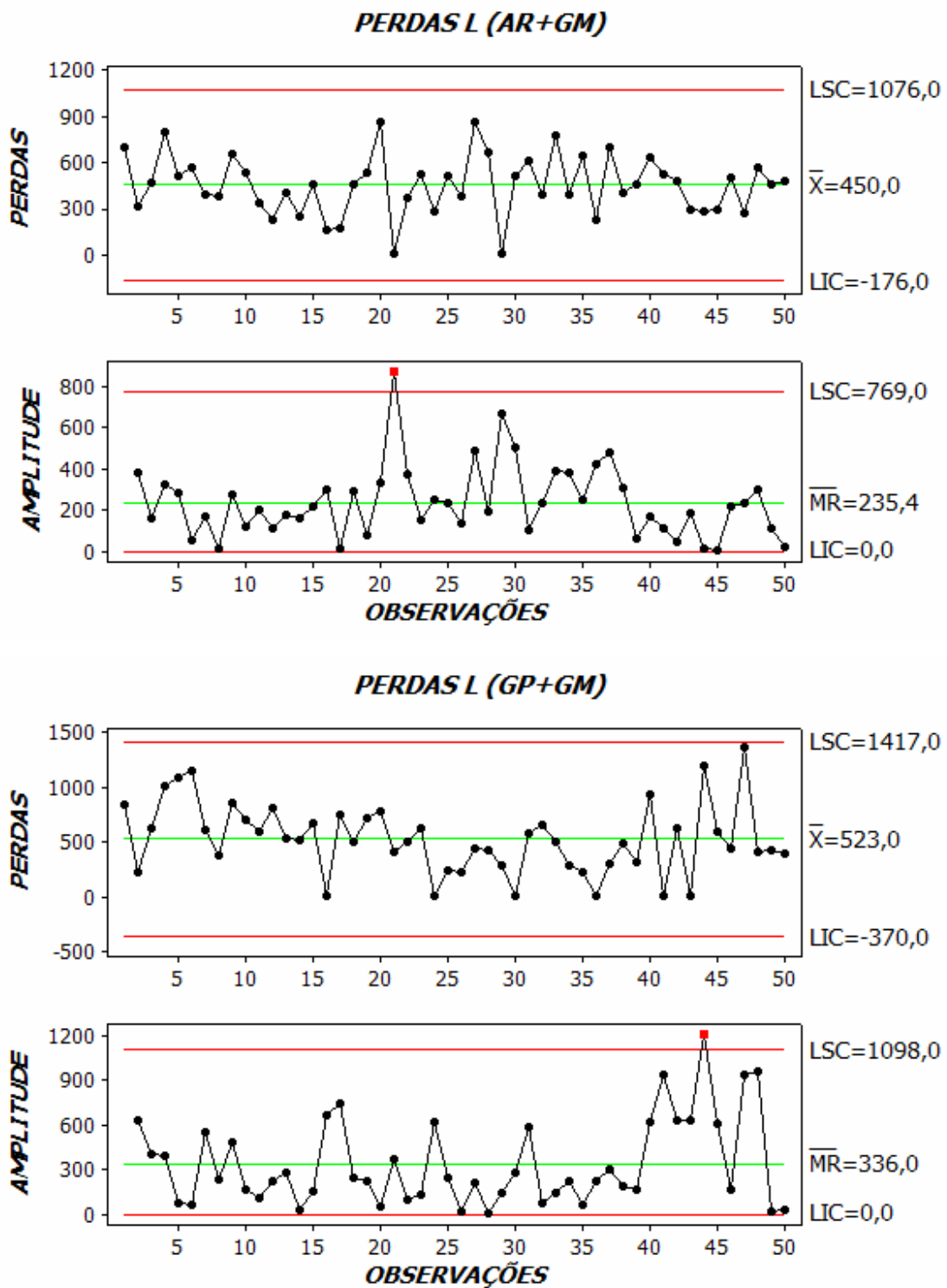
Figura 15. Cartas de controle para perdas de lasca ( \text{kg ha}^{-1} ).
