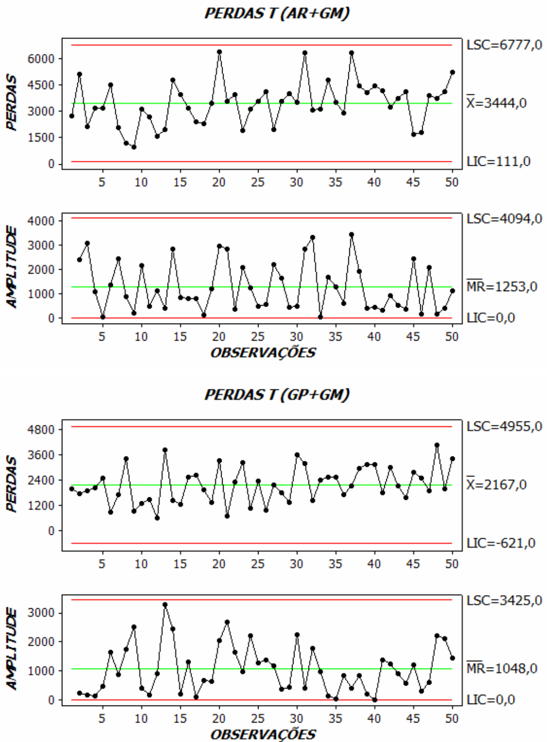
Figura 17. Cartas de controle para perdas de toco ( \text{kg ha}^{-1} ).
