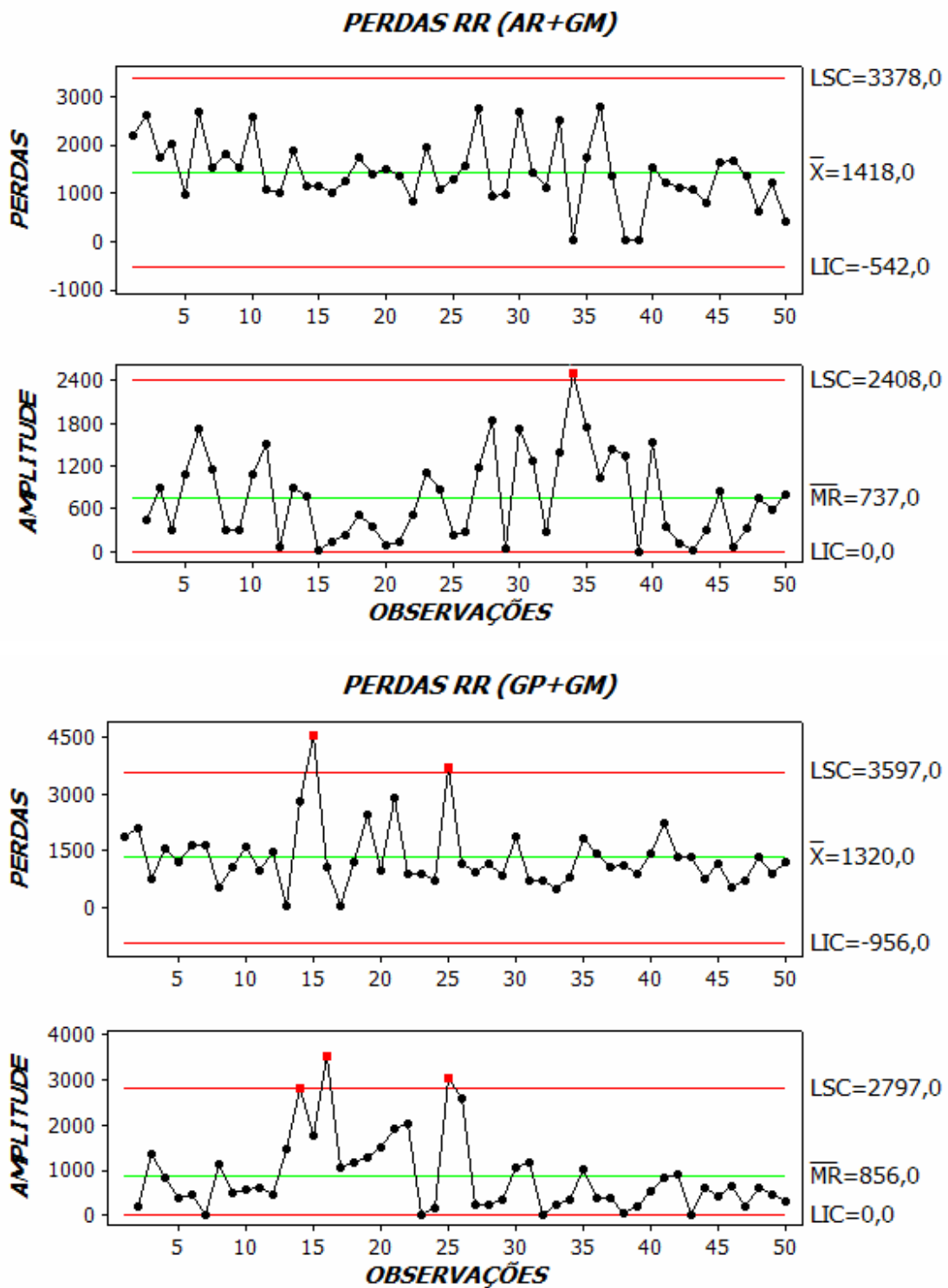
Figura 10. Cartas de controle para perdas de rebolo repicado ( \text{kg ha}^{-1} ).
