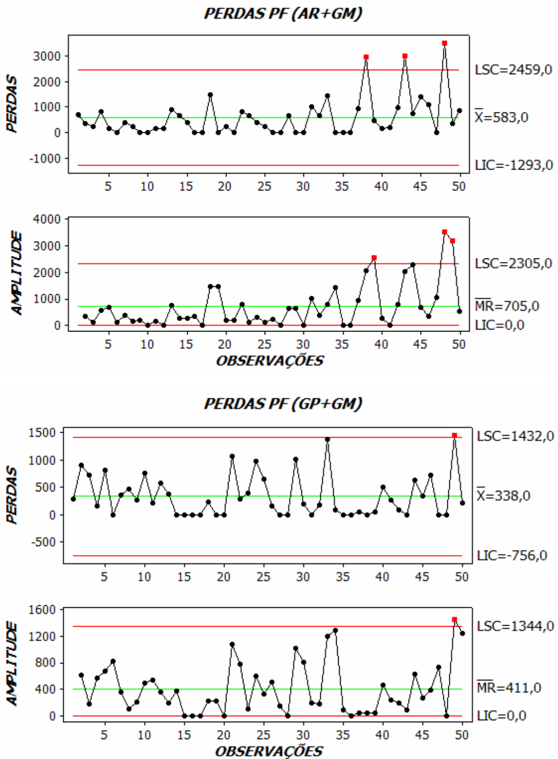
Figura 13. Cartas de controle para perdas de pedaço fixo ( \text{kg ha}^{-1} ).
