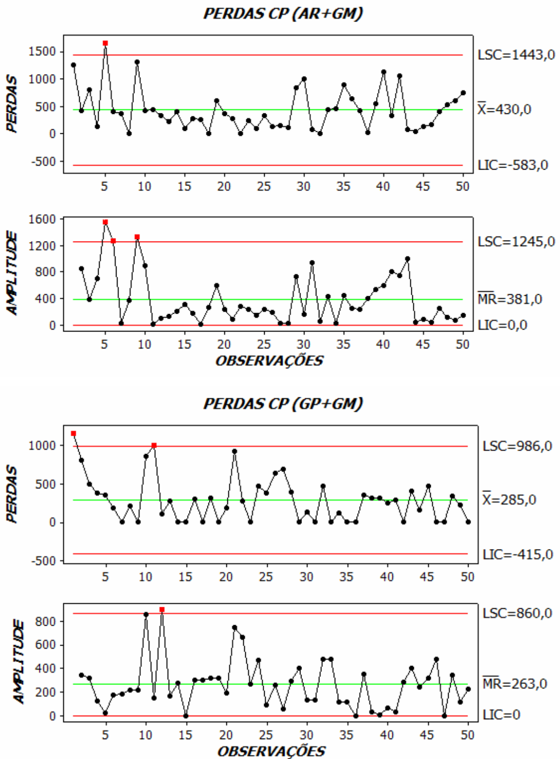
Figura 12. Cartas de controle para perdas de cana-ponta ( \text{kg ha}^{-1} ).
