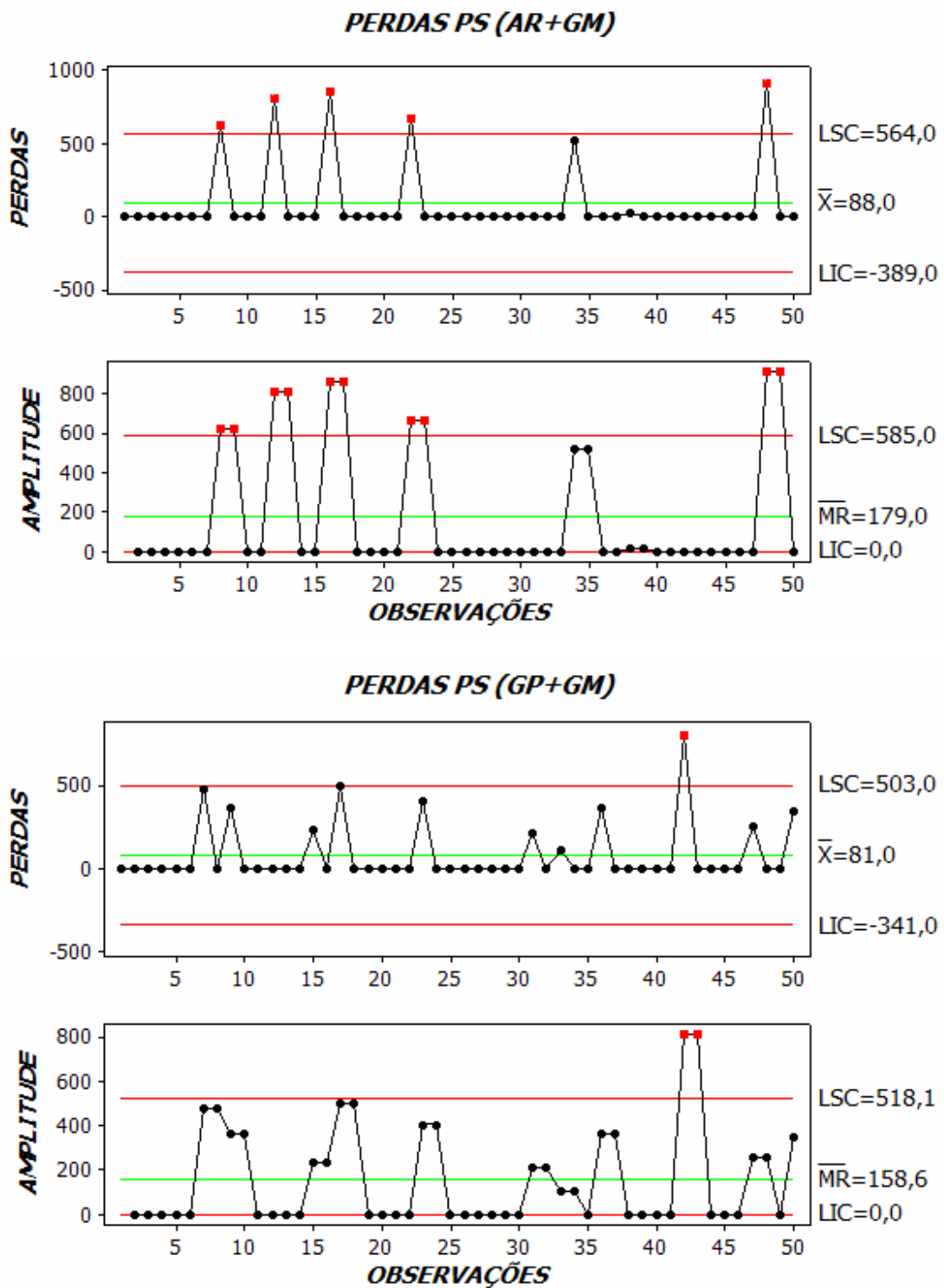
Figura 14. Cartas de controle para perdas de pedaço solto (kg ha -1 ).
