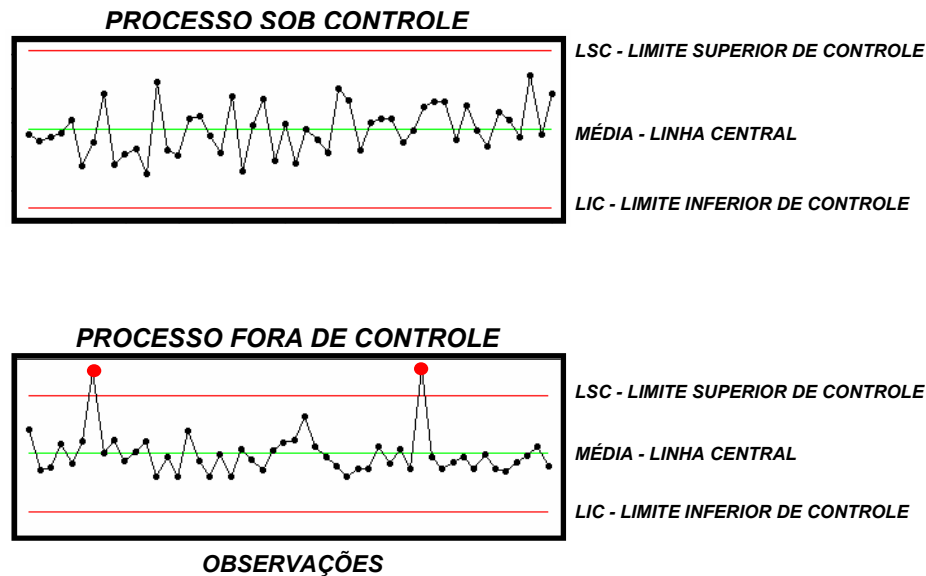
Figura 3. Estrutura das cartas de controle.
