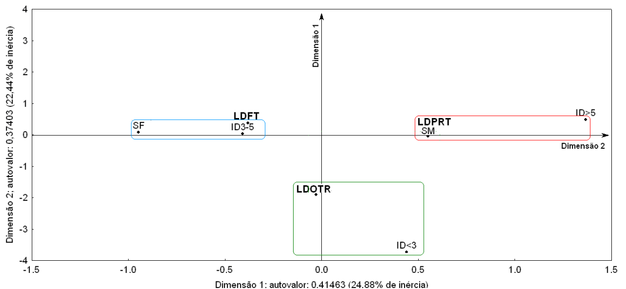
Figura 3. Mapa perceptual das variáveis sexo (SM, SF); idade (ID<3, ID3-5, ID>5) e laudo (LDFT, LDPRT, LDOTR); para a análise de correspondência multivariada da avaliação das lesões (primeira etapa) do ano de 2003.
