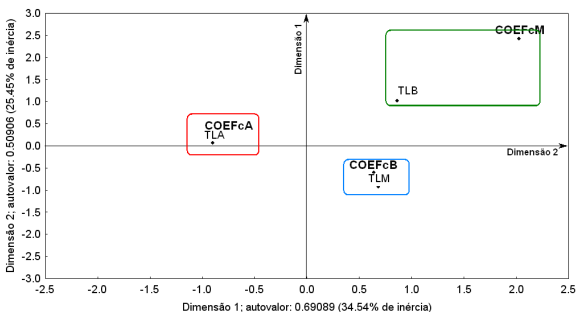
Figura 6. Mapa perceptual das variáveis COEFcA – alto coeficiente de comprometimento da lesão; COEFcM – médio coeficiente de comprometimento da lesão; COEFcB – baixo coeficiente de comprometimento da lesão; TLA – topografia da lesão alta; TLM - topografia da lesão média; TLB - topografia da lesão baixa; para a análise de correspondência multivariada da avaliação de campanha das fêmeas (segunda etapa) do ano de 2003.
