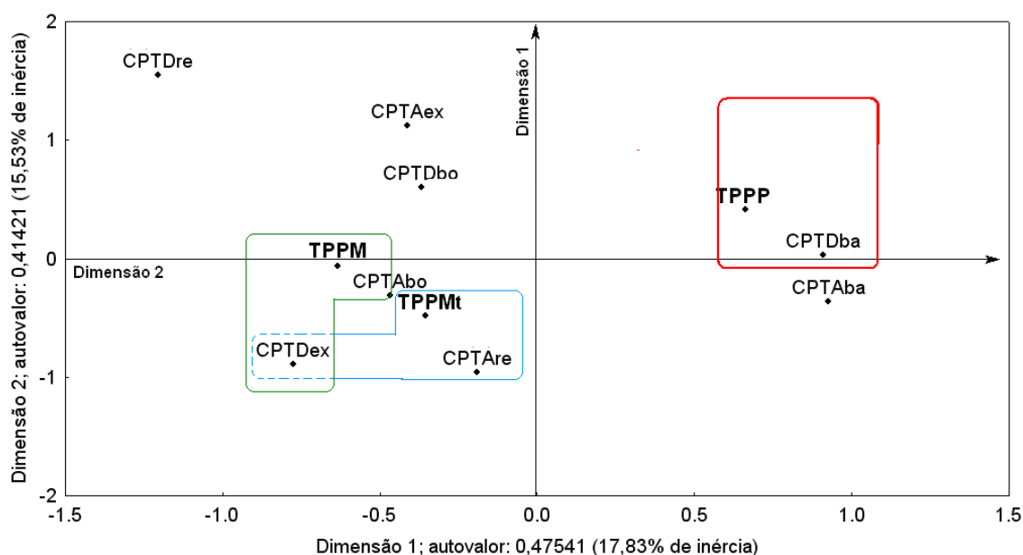
Figura 15. Mapa perceptual das variáveis classe de pontuação antes da lesão (CPTA: ex – excelente; bo - boa; re - regular; ba – baixa); classe de pontuação depois da lesão (CPTD: ex – excelente; bo - boa; re - regular; ba – baixa); tempo parado após a lesão (TPP: Mt – muito; M – médio; P – pouco); para a análise de correspondência multivariada da avaliação de campanha dos machos (segunda etapa) do ano de 2004.
