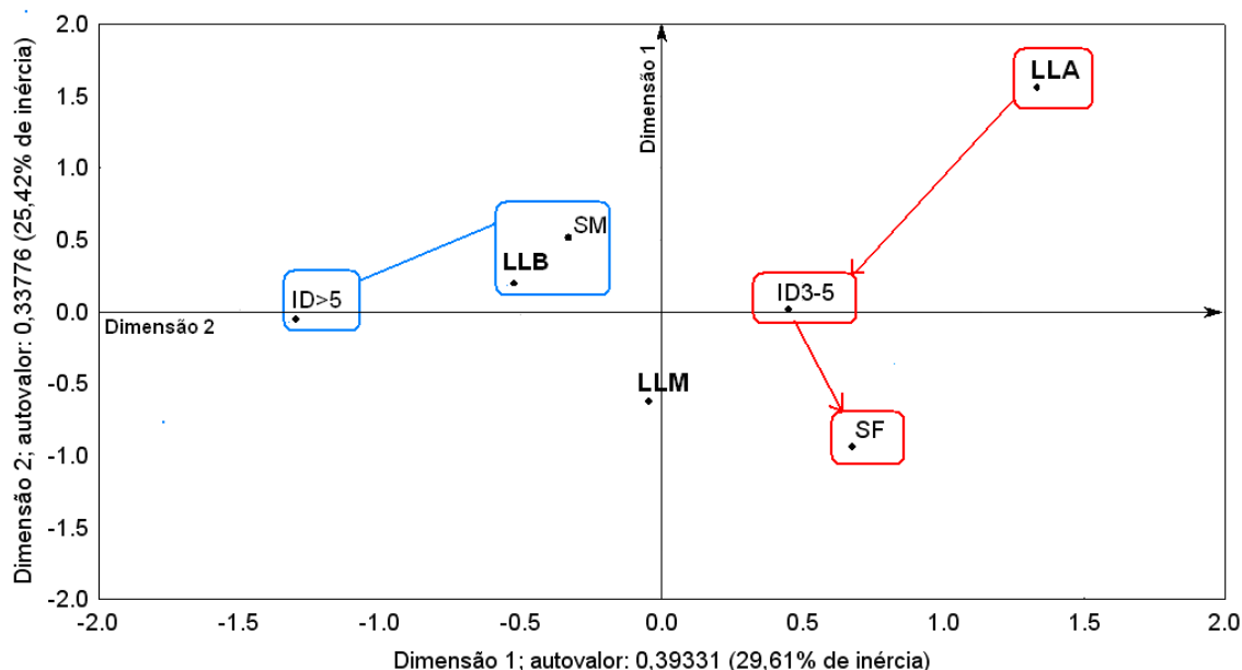
Figura 18. Mapa perceptual das variáveis sexo (SM, SF); idade (ID3-5, ID>5) e local da lesão (LLA, LLM, LLB); para a análise de correspondência multivariada da avaliação das lesões (primeira etapa) do ano de 2005.
