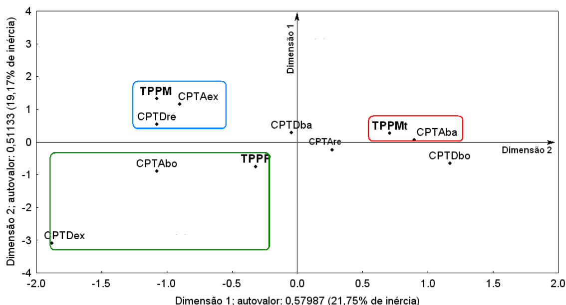
Figura 13. Mapa perceptual das variáveis CPTAex – classe de pontuação antes excelente; CPTAbo – classe de pontuação antes boa; CPTAre – classe de pontuação antes regular; CPTAba – classe de pontuação antes baixa; CPTDex – classe de pontuação depois excelente; CPTDbo – classe de pontuação depois boa; CPTDre – classe de pontuação depois regular; CPTDba – classe de pontuação depois baixa; TPPMt – muito tempo parado; TPPM – médio tempo parado; TPPP – pouco tempo parado; para a análise de correspondência multivariada da avaliação de campanha das fêmeas (segunda etapa) do ano de 2004.
