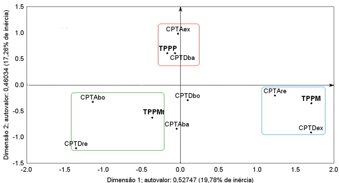
Figura 31. Mapa perceptual das variáveis classe de pontuação antes da lesão (CPTA: ex – excelente; bo - boa; re - regular; ba – baixa); classe de pontuação depois da lesão (CPTD: ex – excelente; bo - boa; re - regular; ba – baixa); tempo parado após a lesão (TPP: Mt – muito; M – médio; P – pouco); para a análise de correspondência multivariada da avaliação de campanha dos machos (segunda etapa) do ano de 2006.
