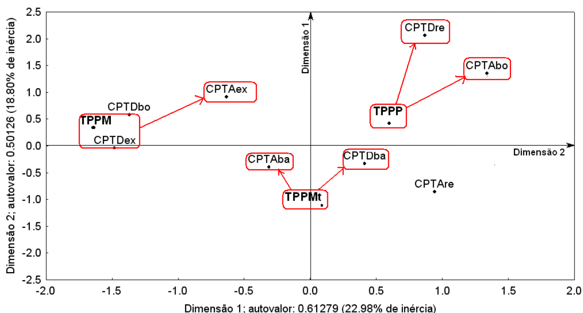
Figura 5. Mapa perceptual das variáveis CPTAex – classe de pontuação antes excelente; CPTAbo - classe de pontuação antes boa; CPTAre - classe de pontuação antes regular; CPTAba - classe de pontuação antes baixa; CPTDex – classe de pontuação depois excelente; CPTDbo - classe de pontuação depois boa; CPTDre - classe de pontuação depois regular; CPTDbA - classe de pontuação depois baixa; TPPMt – muito tempo parado; TPPM – médio tempo parado; TPPP – pouco tempo parado; para a análise de correspondência multivariada da avaliação de campanha das fêmeas (segunda etapa) do ano de 2003.
