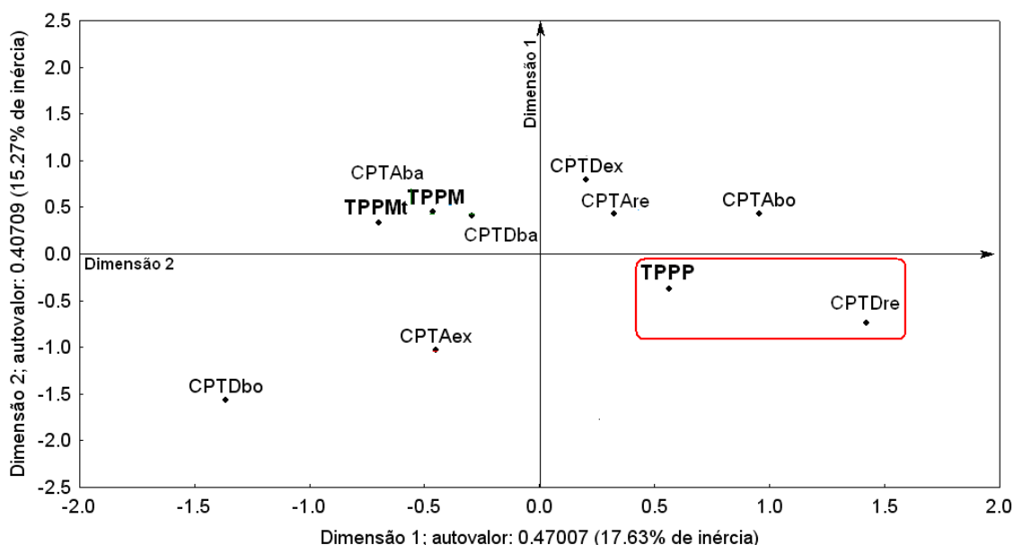
Figura 7. Mapa perceptual das variáveis CPTAex – classe de pontuação antes excelente; CPTAbo - classe de pontuação antes boa; CPTAre - classe de pontuação antes regular; CPTAba - classe de pontuação antes baixa; CPTDex – classe de pontuação depois excelente; CPTDbo - classe de pontuação depois boa; CPTDre - classe de pontuação depois regular; CPTDba - classe de pontuação depois baixa; TPPMt – muito tempo parado; TPPM – médio tempo parado; TPPP – pouco tempo parado; para a análise de correspondência multivariada da avaliação de campanha dos machos (segunda etapa) do ano de 2003.
