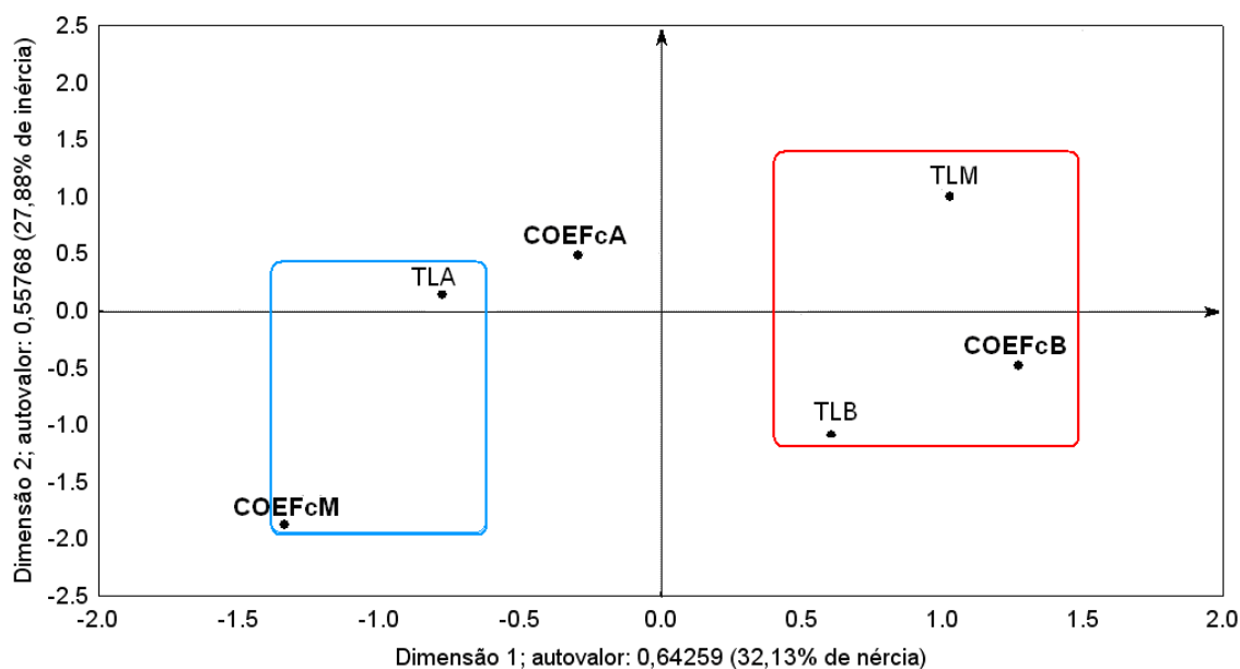
Figura 24. Mapa perceptual das variáveis COEFcA – alto coeficiente de comprometimento da lesão; COEFcM – médio coeficiente de comprometimento da lesão; TLA – topografia da lesão alta; TLM - topografia da lesão média; TLB - topografia da lesão baixa; para a análise de correspondência multivariada da avaliação de campanha dos machos (segunda etapa) do ano de 2005.
