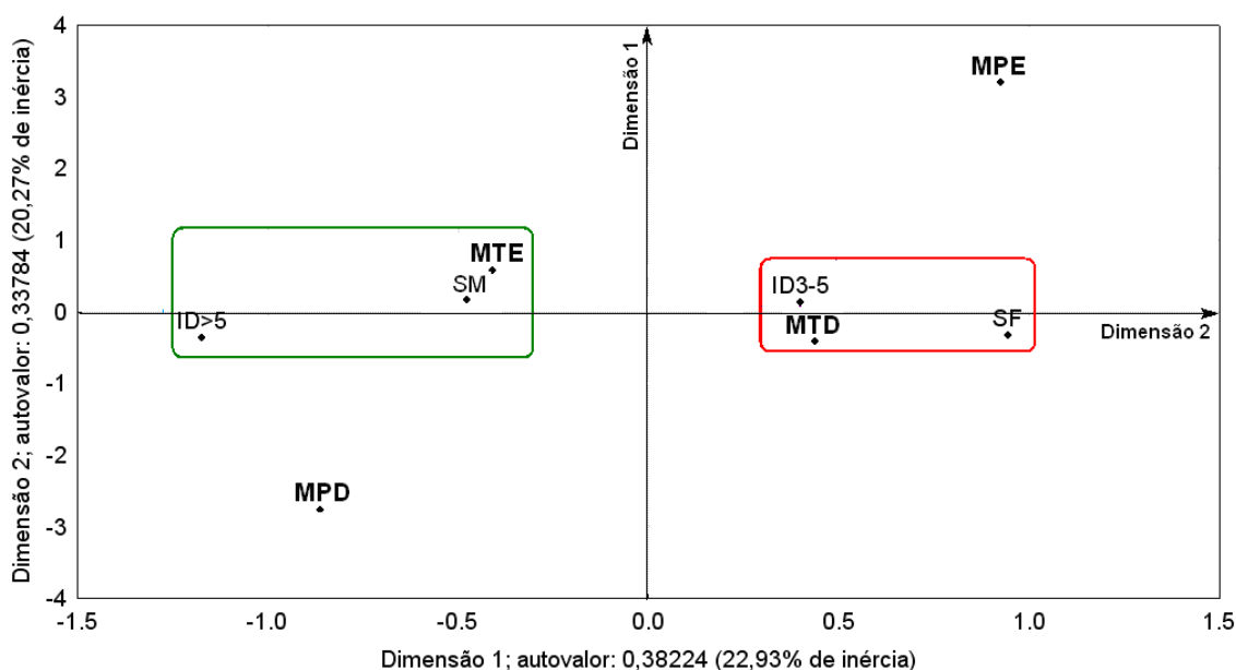
Figura 17. Mapa perceptual das variáveis sexo (SM, SF); idade (ID3-5, ID>5) e membro lesionado (MTD, MTE, MPD, MPE); para a análise de correspondência multivariada da avaliação das lesões (primeira etapa) do ano de 2005.
