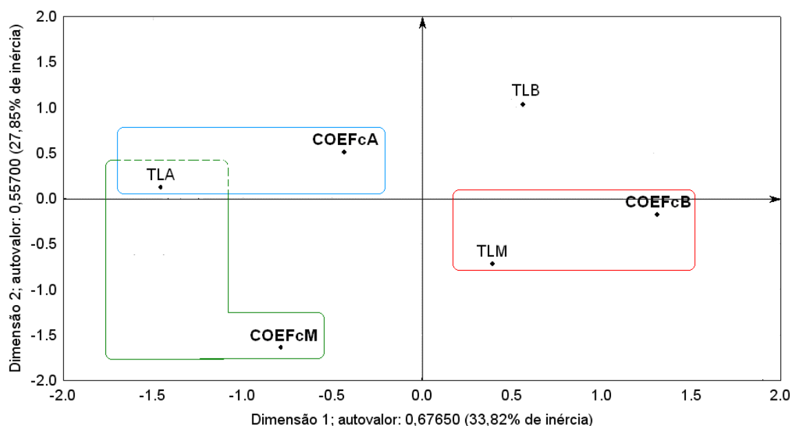
Figura 32. Mapa perceptual das variáveis COEFcA – alto coeficiente de comprometimento da lesão; COEFcM – médio coeficiente de comprometimento da lesão; COEFcB – baixo coeficiente de comprometimento da lesão; TLA – topografia da lesão alta; TLM - topografia da lesão média; TLB - topografia da lesão baixa; para a análise de correspondência multivariada da avaliação de campanha das machos (segunda etapa) do ano de 2006.
