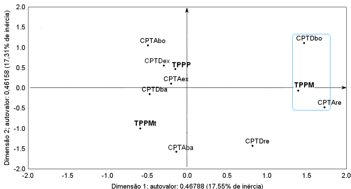
Figura 23. Mapa perceptual das variáveis CPTAex – classe de pontuação antes excelente; CPTAbo - classe de pontuação antes boa; CPTAre - classe de pontuação antes regular; CPTAba - classe de pontuação antes baixa; CPTDex – classe de pontuação depois excelente; CPTDbo - classe de pontuação depois boa; CPTDre - classe de pontuação depois regular; CPTDbA - classe de pontuação depois baixa; TPPMt – muito tempo parado; TPPM – médio tempo parado; TPPP – pouco tempo parado; para a análise de correspondência multivariada da avaliação de campanha dos machos (segunda etapa) do ano de 2005.
