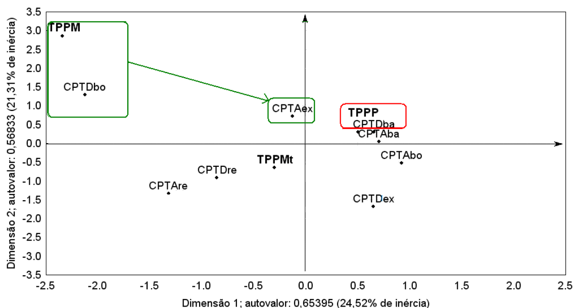
Figura 21. Mapa perceptual das variáveis CPTAex – classe de pontuação antes excelente; CPTAbo - classe de pontuação antes boa; CPTAre - classe de pontuação antes regular; CPTAba - classe de pontuação antes baixa; CPTDex – classe de pontuação depois excelente; CPTDbo - classe de pontuação depois boa; CPTDre - classe de pontuação depois regular; CPTDba - classe de pontuação depois baixa; TPPMt – muito tempo parado; TPPM – médio tempo parado; TPPP – pouco tempo parado; para a análise de correspondência multivariada da avaliação de campanha das fêmeas (segunda etapa) do ano de 2005.
