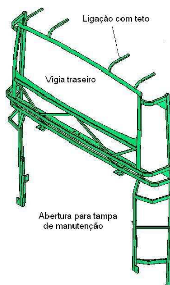
Figura 4.12 – Estrutura traseira
