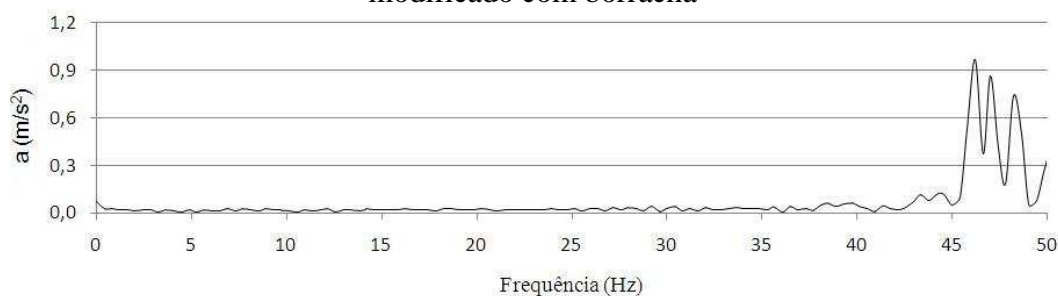
Figura 6.76 – Aceleração vertical estrutura poltrona, asfalto bom estado, projeto modificado com borracha
