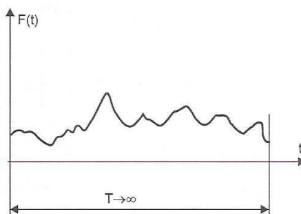
Figura 3.15 – Representação de uma função não periódica qualquer
