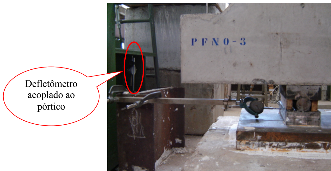
Figura 3.19 – Detalhe do defletômetro no pórtico
