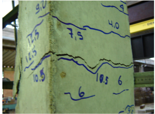
Figura 4.13 – Ruptura do pilar PFN60-3
