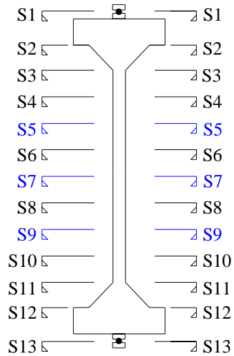
Figura 5.14 – Disposição das seções no pilar
