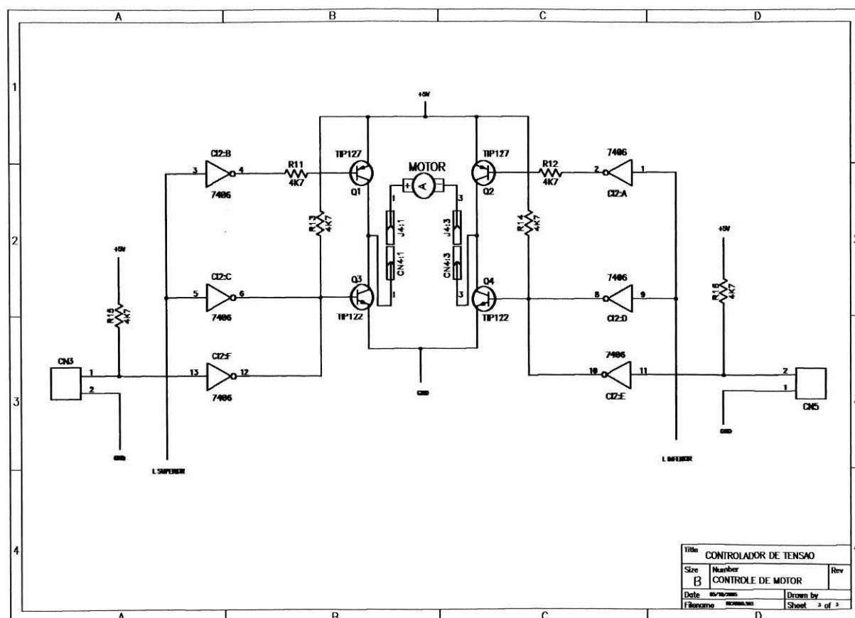
Figura I.1 – Controlador de tensão: etapa de controle de motor do atuador.
