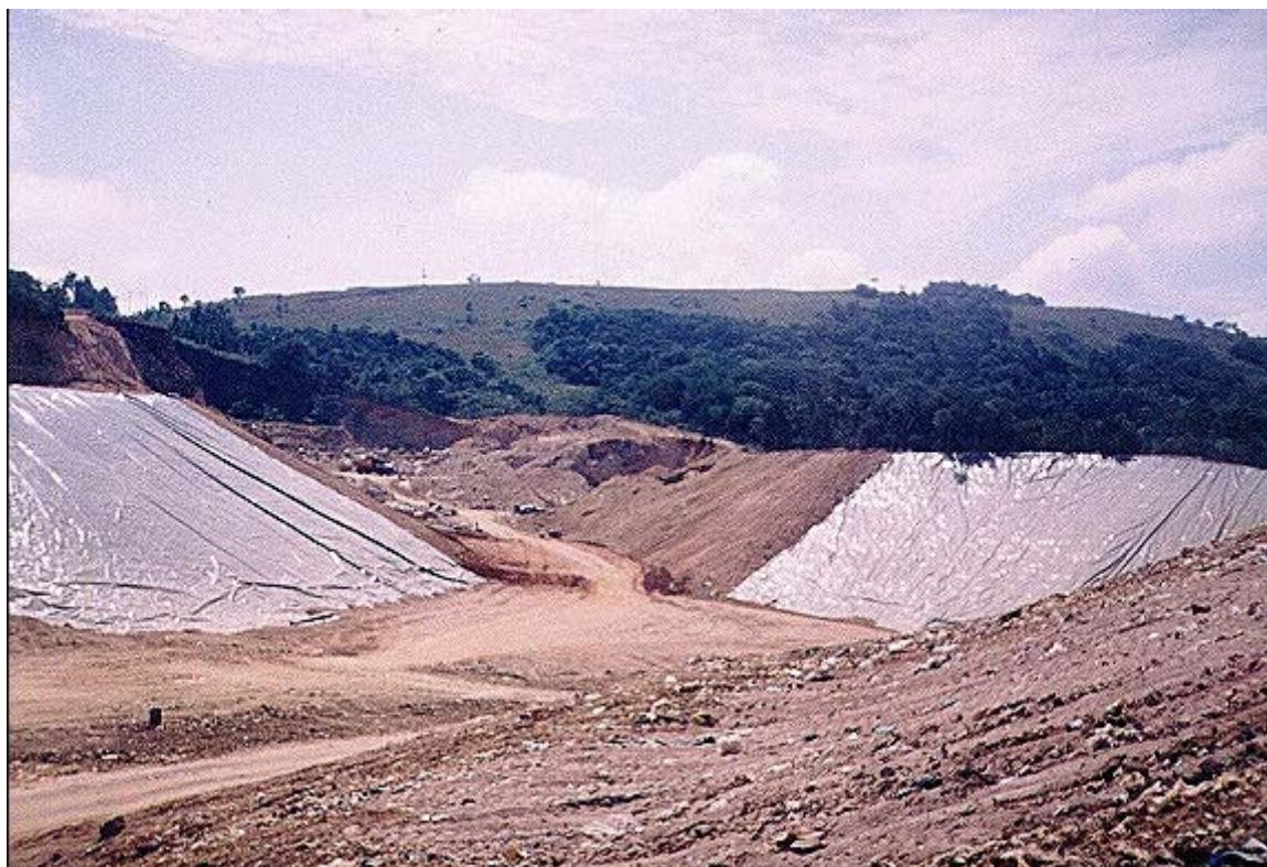
Figura 2.10 – Vista da impermeabilização do aterro. Fonte DMLU.
