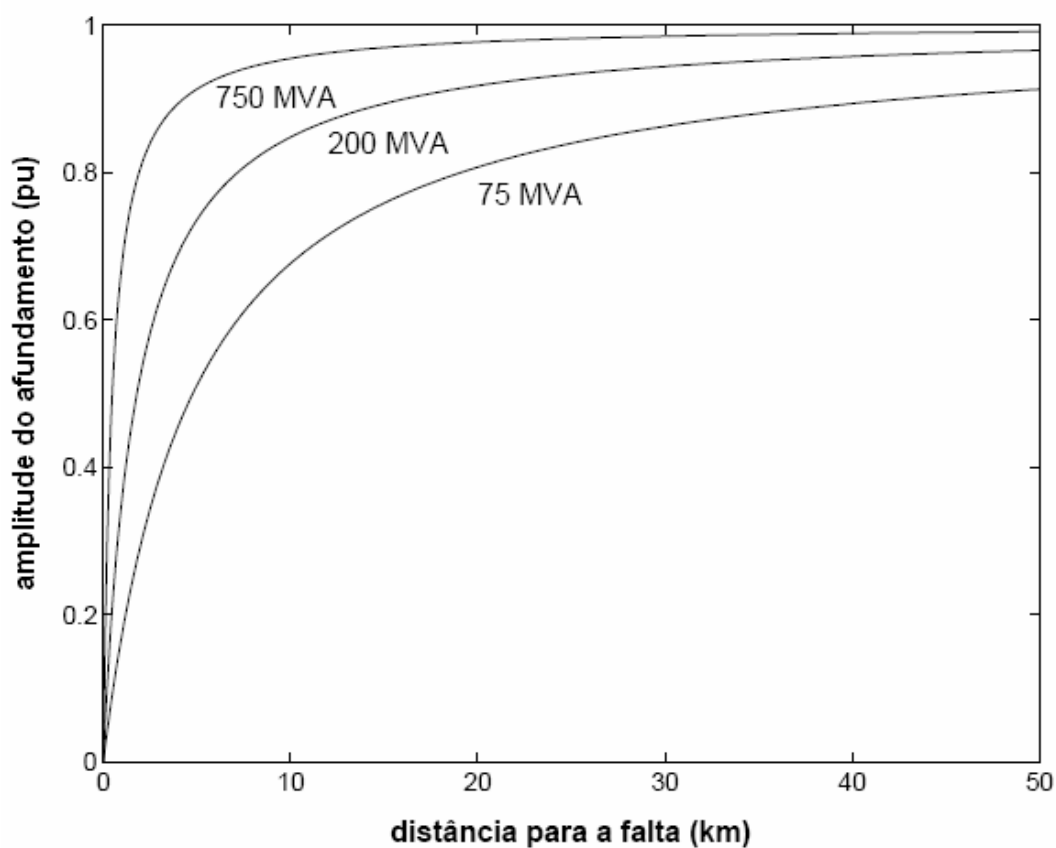
Figura 2.5 – Amplitude do afundamento como função da distância para a falta.
