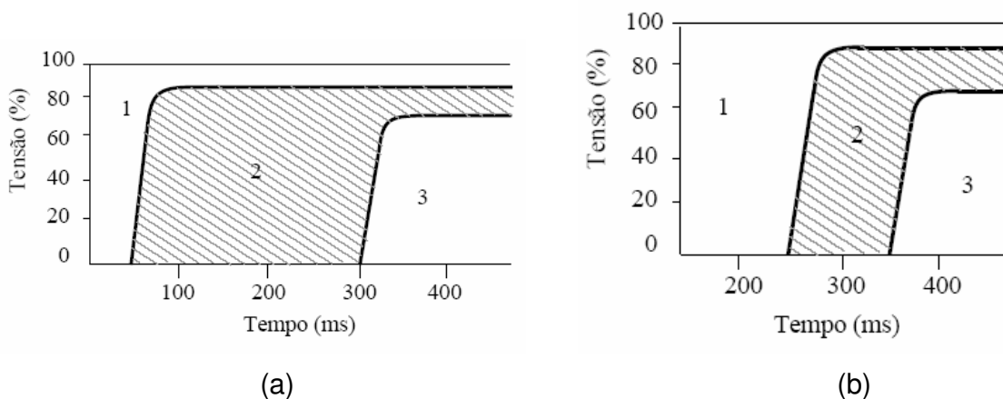
Figura 2.13 – (a) Faixa de sensibilidade do AVV; (b) Faixa de sensibilidade do CLP.
