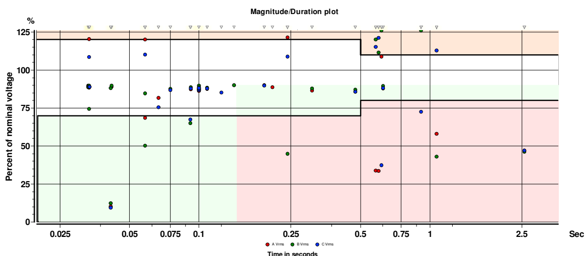
Figura 5.5 – Curvas ITIC sobreposta aos pontos de ocorrência.
