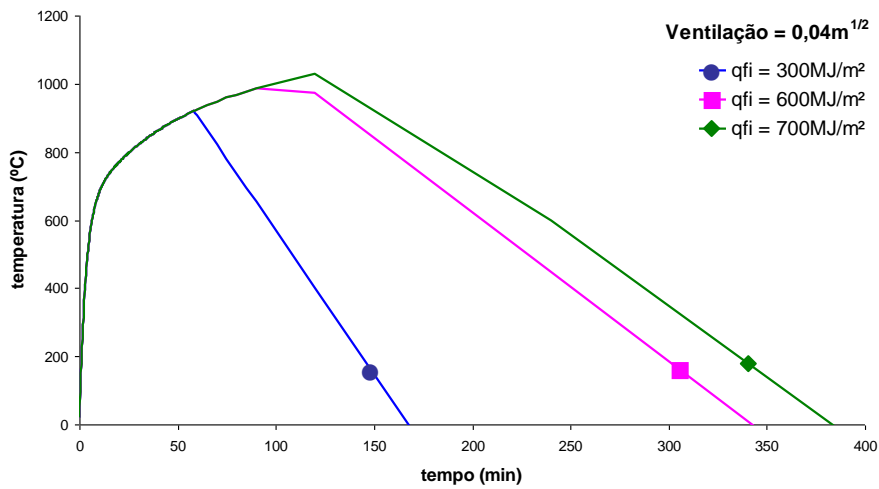
Figura 2.10 – Incêndio natural – Curvas temperatura x tempo (Ventilação = 0,04m 1/2 )
