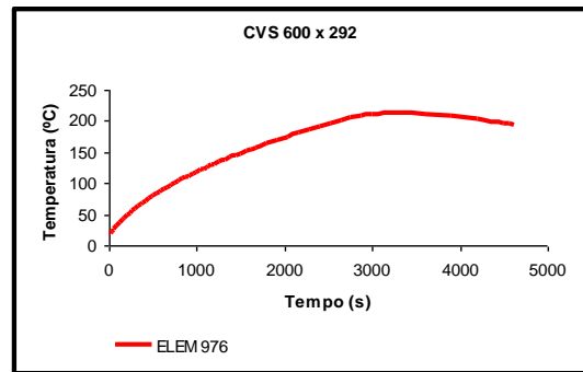
Figura 7.19 – Temperatura dos elementos escolhidos para o perfil CVS 600x292 Incêndio natural 3 - ANSYS
