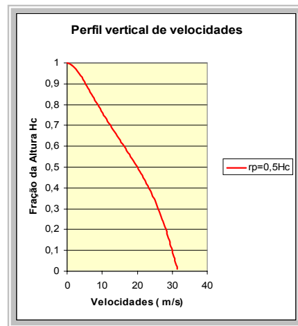
Figura 5.3 - Perfil das velocidades para r_p = 0,5h
