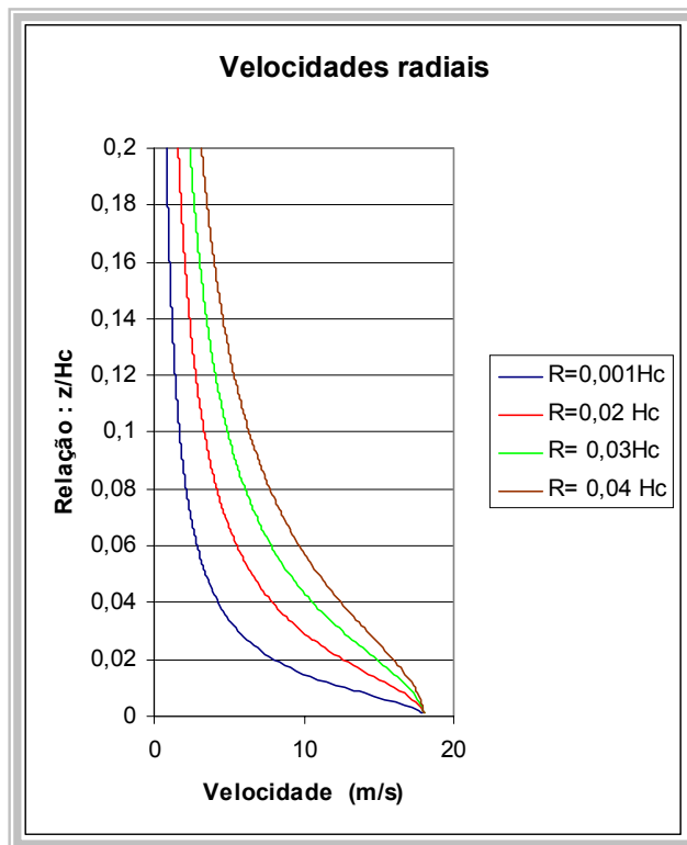
Figura 4.8 - Velocidades radiais
