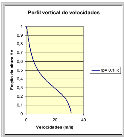
Figura 5.2- Perfil das velocidades para r_p = 0,1h
