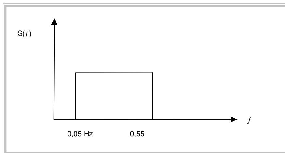
Figura 6.1– Ruído branco em faixa ( frequência em Hz)
