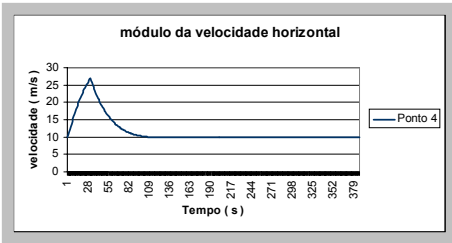
Figuras 7.6– Módulos das velocidades Ponto 4
