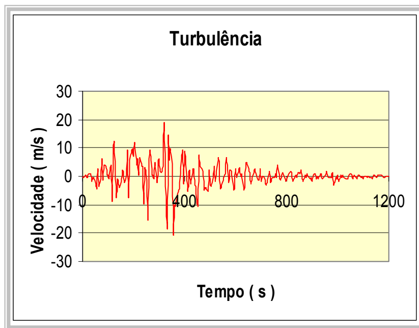
Figura 6.2 - Componente flutuante
