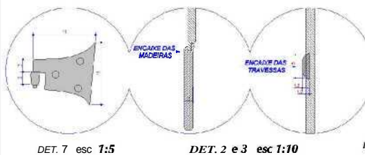
DET. 7 esc 1:5
