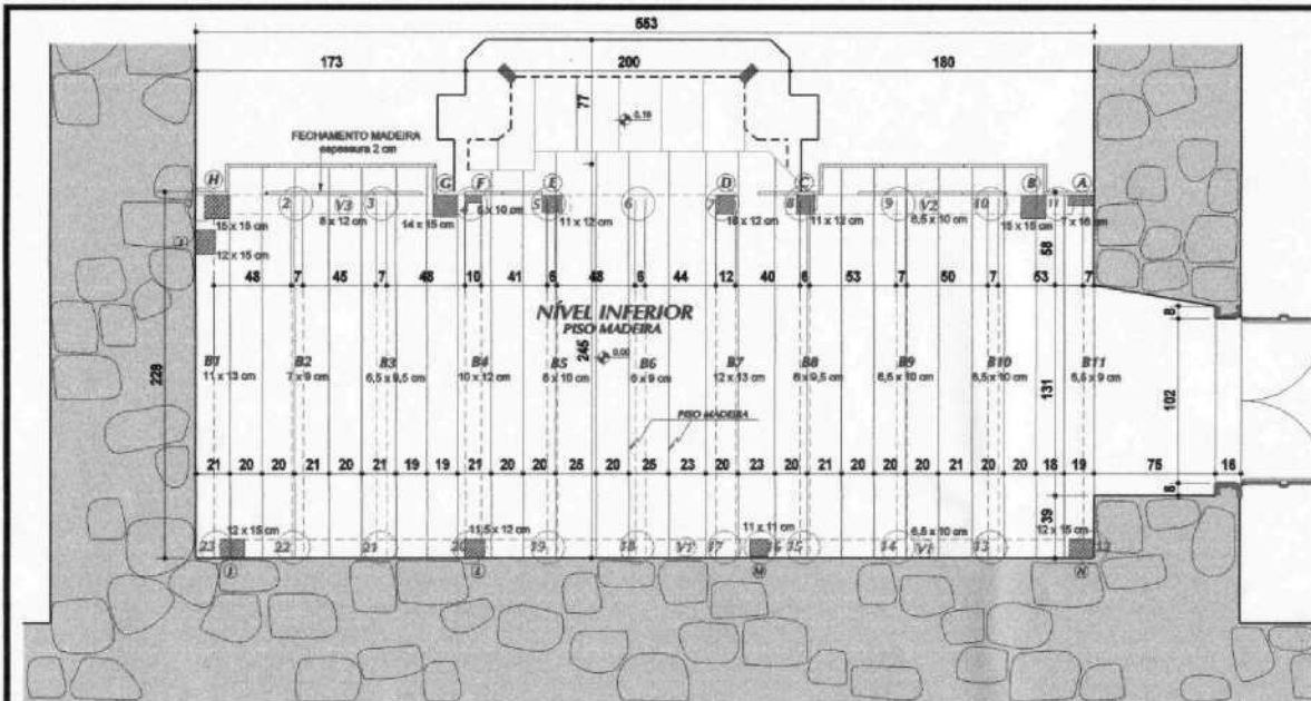
PLANTA BAIXA NÍVEL INFERIOR/ BARROTEAMENTO DO ASSOALHO DA TRIBUNA
