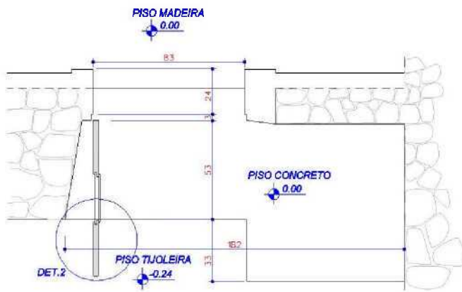
CORTE HORIZONTAL esc 1:25
