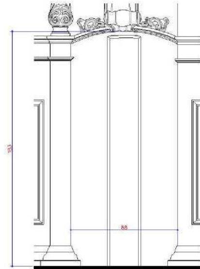
VISTA EXTERNA esc 1:25
