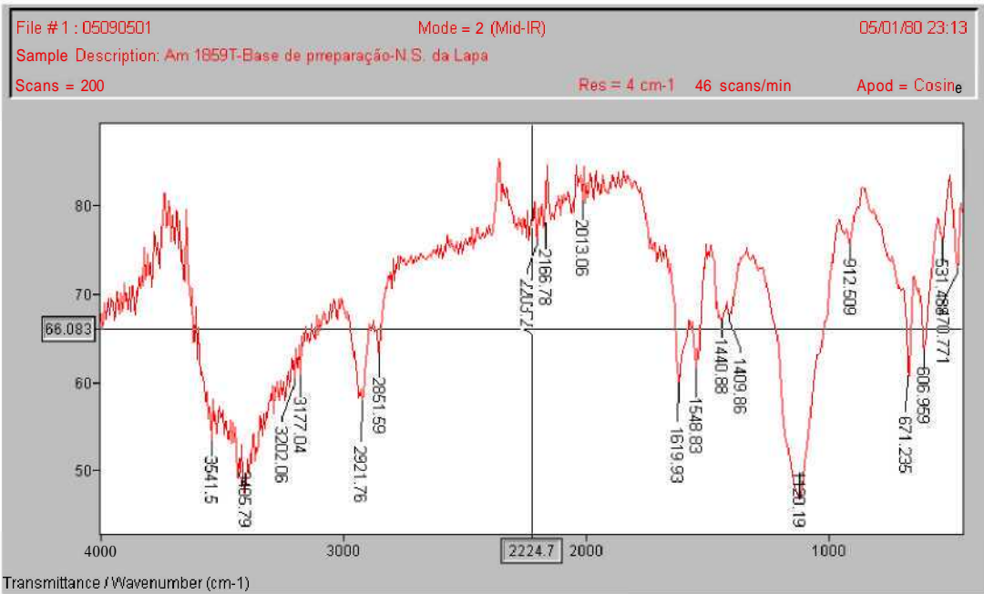
Dustração - Espectro da base de preparação, da amostra 1859T. Igreja Nossa Senhora da Lapa. Fonte - LACICOR, CECOR, UFMG, 2005.
