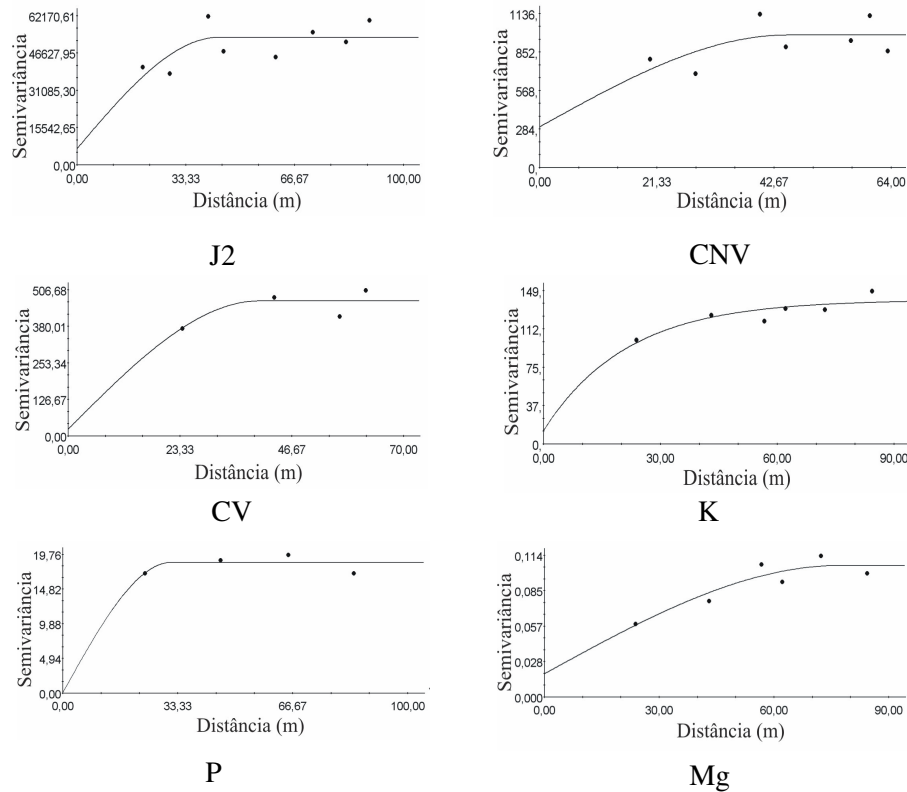
Figura 1. Semivariogramas isotrópicos experimentais da infestação do nematóide do cisto da soja ( N^{\circ}/100\text{ cm}^3 ) e do teor de nutrientes no solo ajustados para (J2) Juvenis de segundo estágio; (CNV) Cistos não viáveis; (CV) Cistos viáveis; (d) Potássio ( \text{mg dm}^{-3} ); (e) Fósforo ( \text{mg dm}^{-3} ) e (f) Magnésio ( \text{cmol}_c\text{ dm}^{-3} ). UFLA, Lavras, Mg, 2008.
