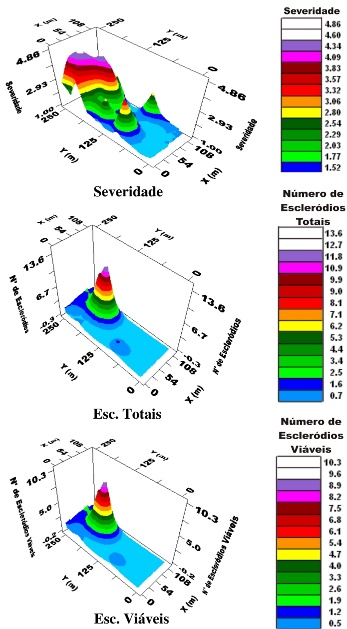
Figura 2. Mapas de krigagem ordinária para a severidade do mofo branco; Esc. Totais - número total de escleródios por Kg de solo; Esc. Viáveis - número de escleródios viáveis por kg de solo na área não colhida. UFLA, Lavras - MG, 2008.
