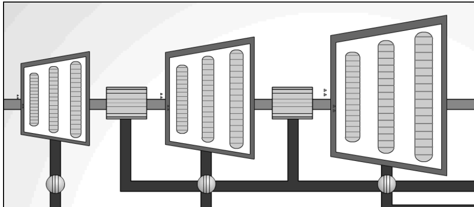
Figura 4.7 – Representação das Turbinas de Baixa e Alta pressão do Secundário
