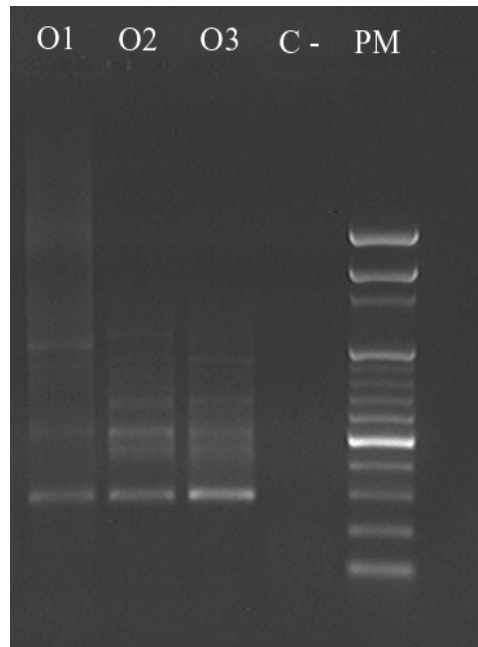
Figura 21 Eletroforese dos amplicons da nested-PCR – Experimento 4
