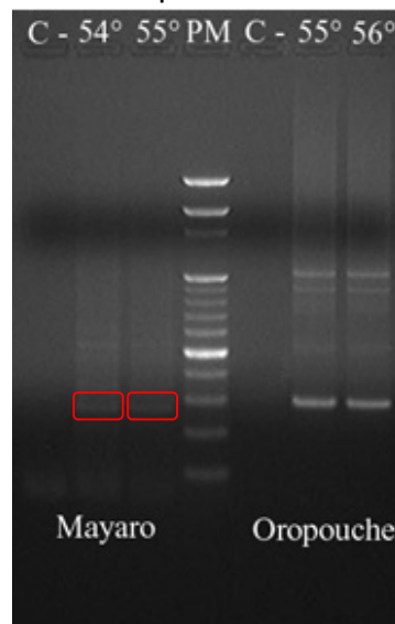
Figura 20. Eletroforese dos amplicons da nested-PCR – Experimento 3
