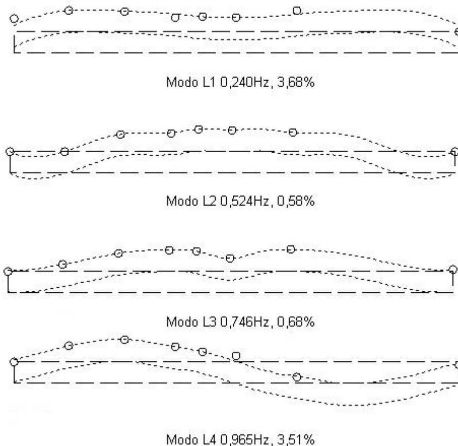
Figura 7. 48 – Modos laterais de vibração – IWCM (L1 – L4).
