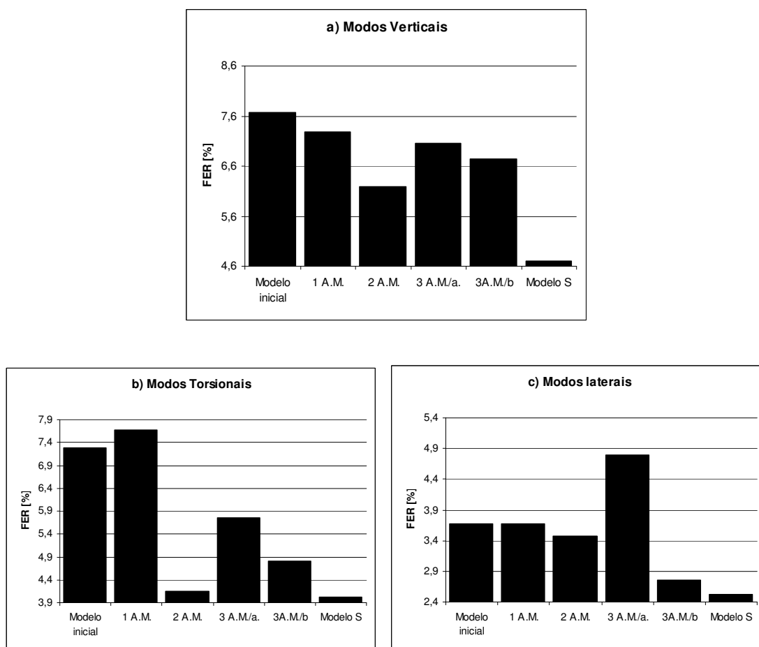
Figura 7. 57 –Porcentagem de variação de frequência média entre todos os a) modos verticais, b) modos torsionais e c) modos laterais.
