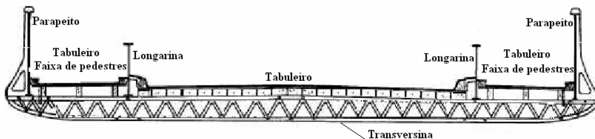
Figura 7. 8 – Seção transversal da CSB.
