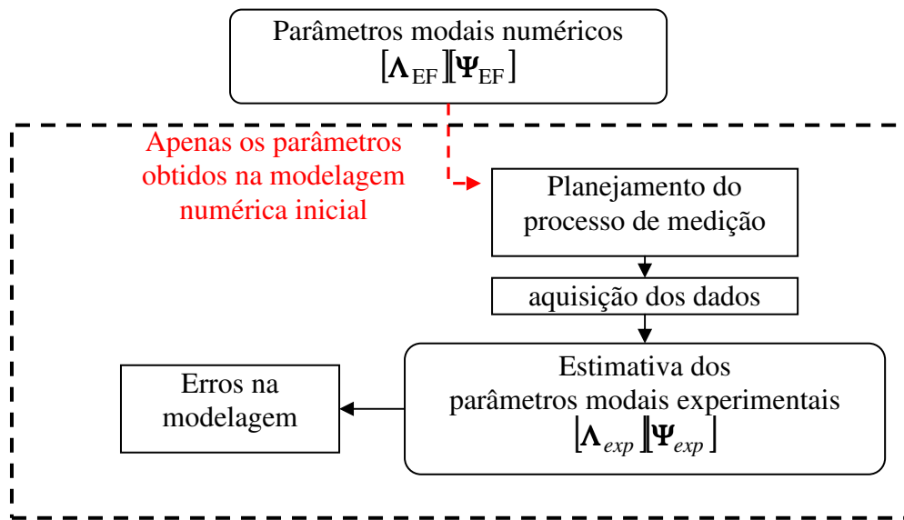
Figura 4. 1 – Fluxograma do processo de modelagem modal experimental.
