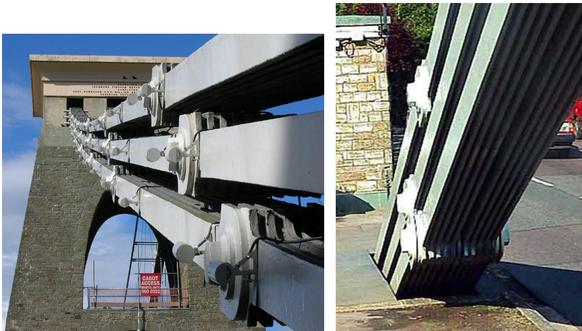
Figura 7.5 – Fotos mostrando os detalhes do cabo.
