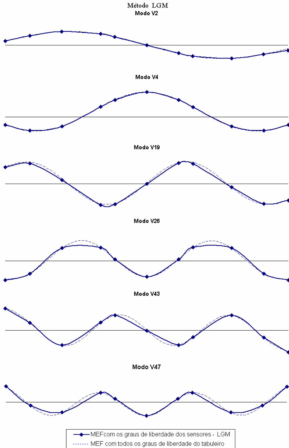
Figura 7.35 – Modos de vibração verticais em elementos finitos – pontos dos sensores obtidos pelo método LGM (1° ao 6° modos verticais obtidos).
