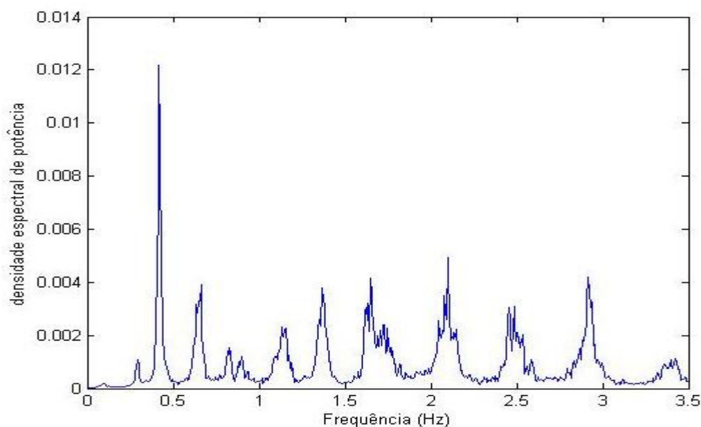
Figura 7. 49 – Densidade espectral para os modos verticais.
