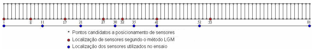
Figura 7. 34 – Localização dos sensores segundo o método LGM e a utilizada no ensaio.
