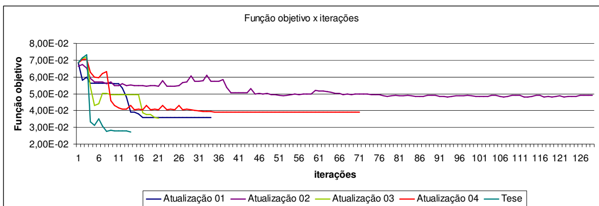
Figura 7. 64 – Função objetivo x iterações para 5 diferentes projetos de atualização automática.
