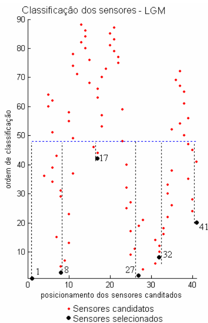
Figura 7. 32 – Classificação dos sensores segundo o método LGM considerando eixo de simetria– Modos verticais – Tabuleiro da ponte pênsil de Bristol.
