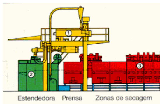
Figura 5.1. Estágio pré-secador (3) da linha contínua de produção de massa longa
