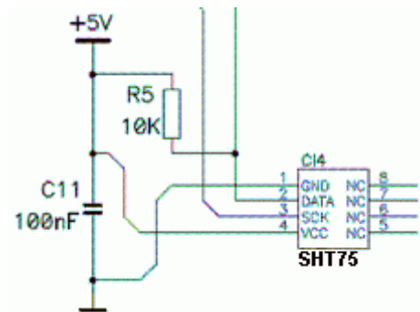
Figura 6.6 – Circuito elétrico de ligação do SHT75.
