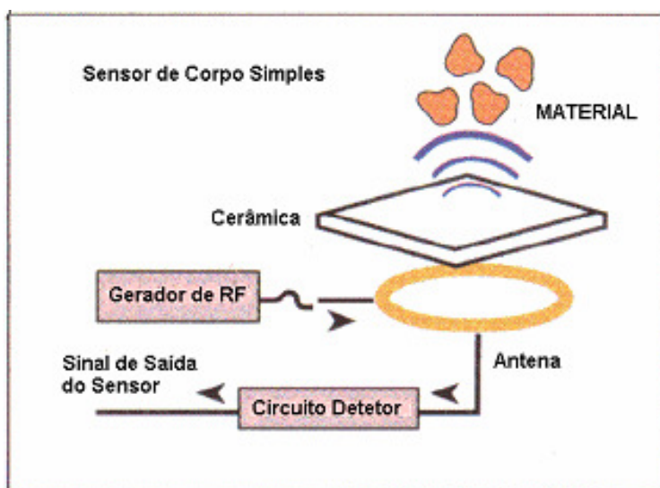
Figura 2.2 Emissão e recepção de microondas
