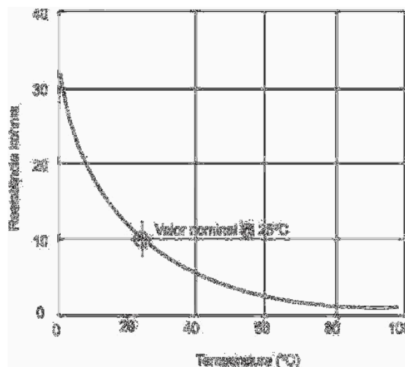
Figura 2.5 – Curva da resistência de um termistor NTC de 10 k \Omega em função da temperatura (modificado de Kester, 2004).
