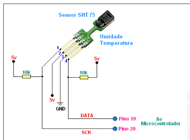
Figura 5.2 Sensor SHT75
