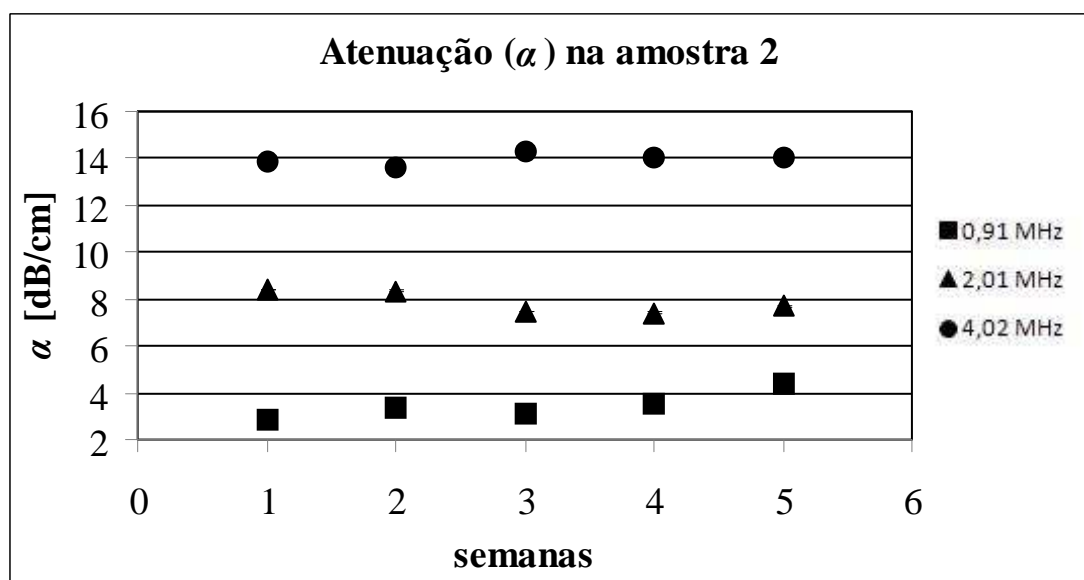
Figura V.3 – Valores de média de atenuação da amostra 2 nas cinco semanas de medições, nas frequências de 0,91, 2,01 e 4,02 MHz.
