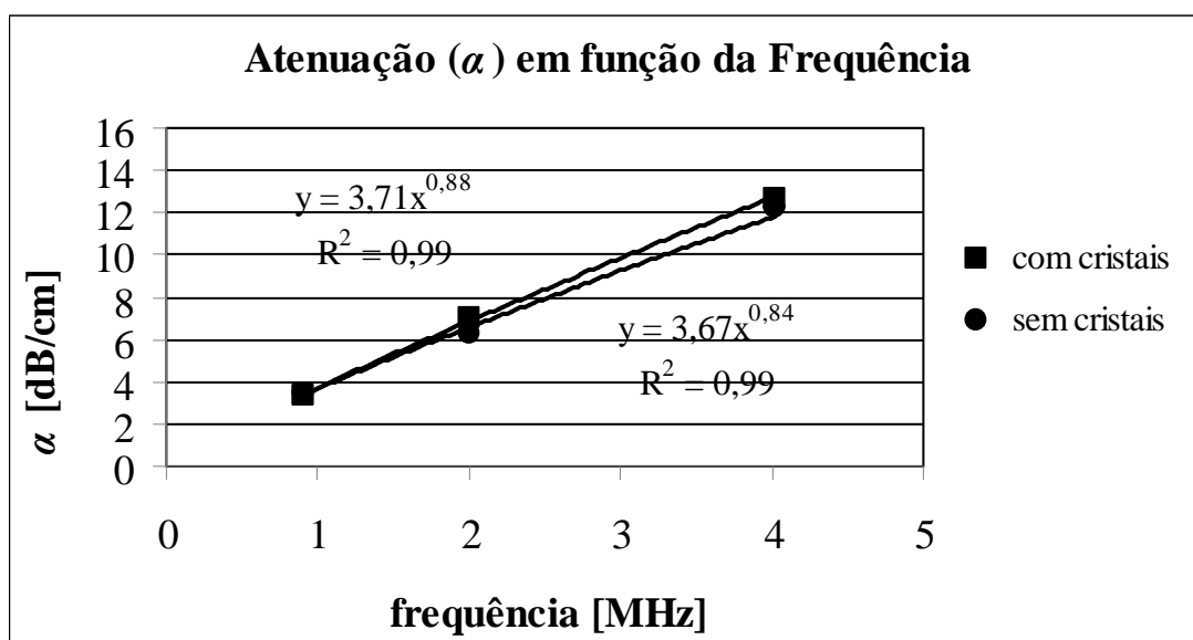
Figura V.10 – Variação da atenuação em função da frequência. Foram traçadas curvas de regressão em potência. As equações e coeficientes para com e sem cristais estão à esquerda e direita, respectivamente.
