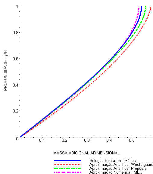
Figura 2.6 - Massa Adicional na face da barragem ao longo da altura M(0,y/H) .
