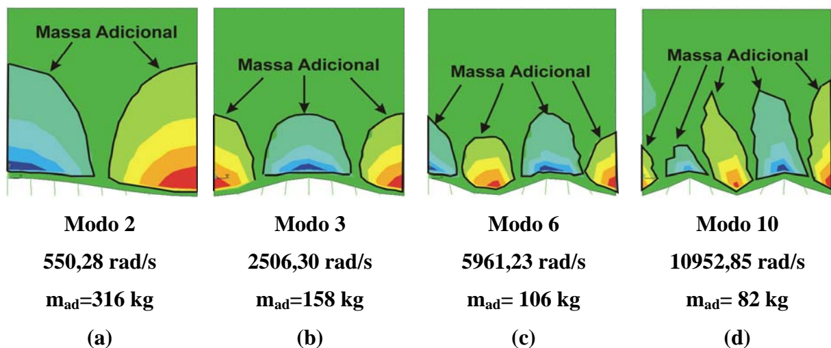
Figura 4.16 – Modos dominados pela estrutura com massa adicional de fluido.
