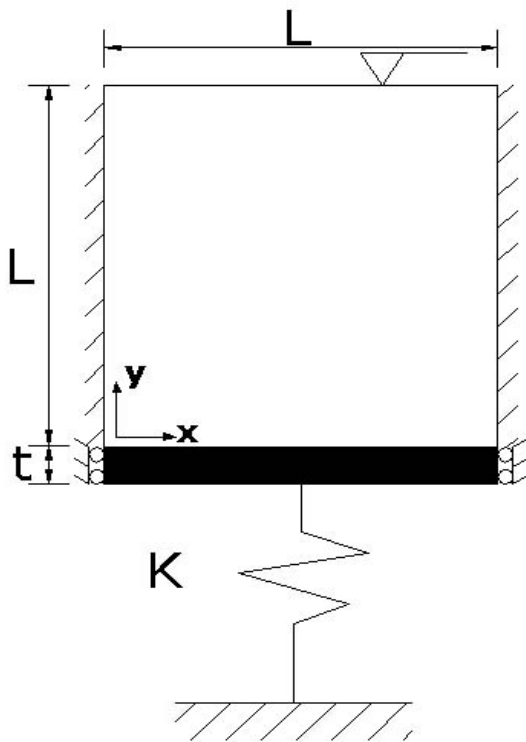
Figura 4.3 – Caso 1- Modelo pistão-cavidade 2D com extremidade superior aberta
