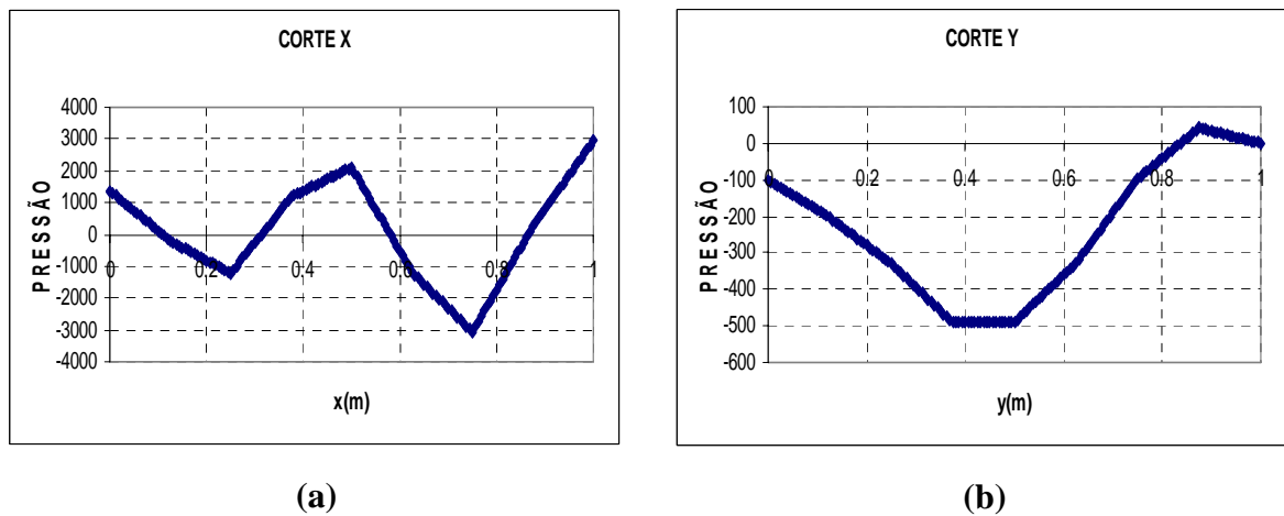
Figura B.17 – Cortes na cavidade do modo 10, Figura 4.14-(j); (a) Corte em x, (b) Corte em y
