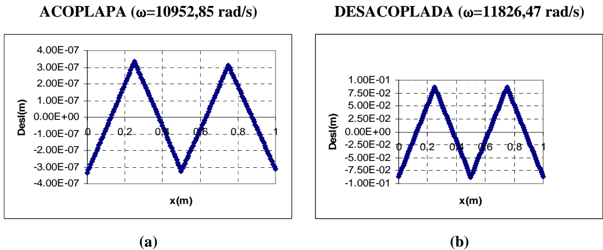
Figura B.16 – Formas modais da estrutura;(a) modo acoplado, Figura 4.14-(j); (b) modo desacoplado, Figura 4.7.
