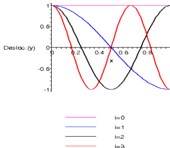
Figura 4.6 – Deformadas analíticas dos modos naturais da viga
