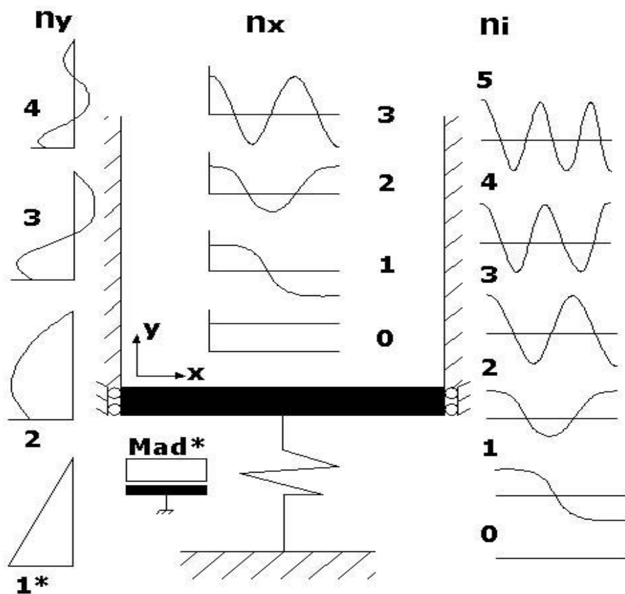
Figura 4.17 – Modos típicos transversais e longitudinais da cavidade e da estrutura (caso 1)
