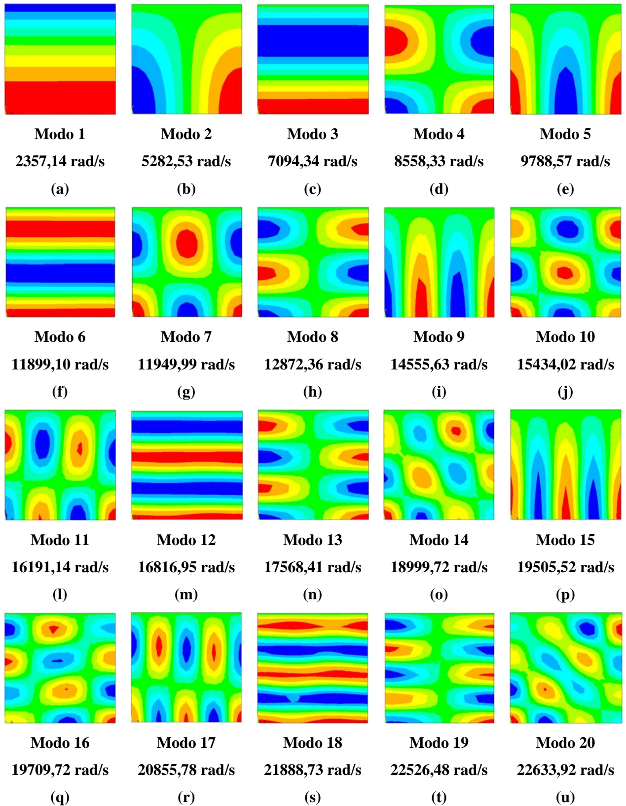
Figura 4.12 – Representação 2D dos modos desacoplados da cavidade aberta obtidos via ANSYS.
