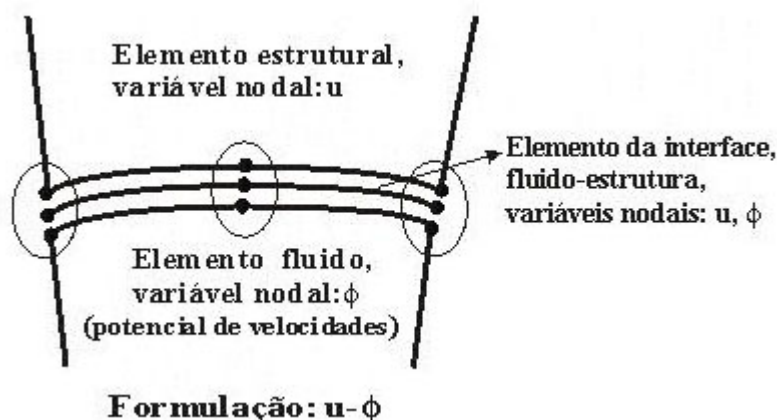
Figura 3.1- Deslocamento no sólido ( u ) e potencial de velocidades no fluido ( \phi ).
