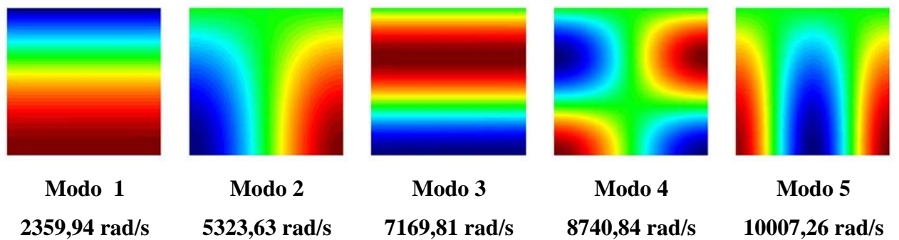
Figura 5.7 – Representação 2D dos cinco primeiros modos desacoplados da cavidade aberta obtidos pelo FEDYFE
