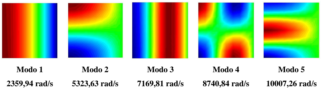
Figura 5.18 – Representação 2D dos modos desacoplados da cavidade aberta com 2 placas móveis obtidos pelo FEDYFE
