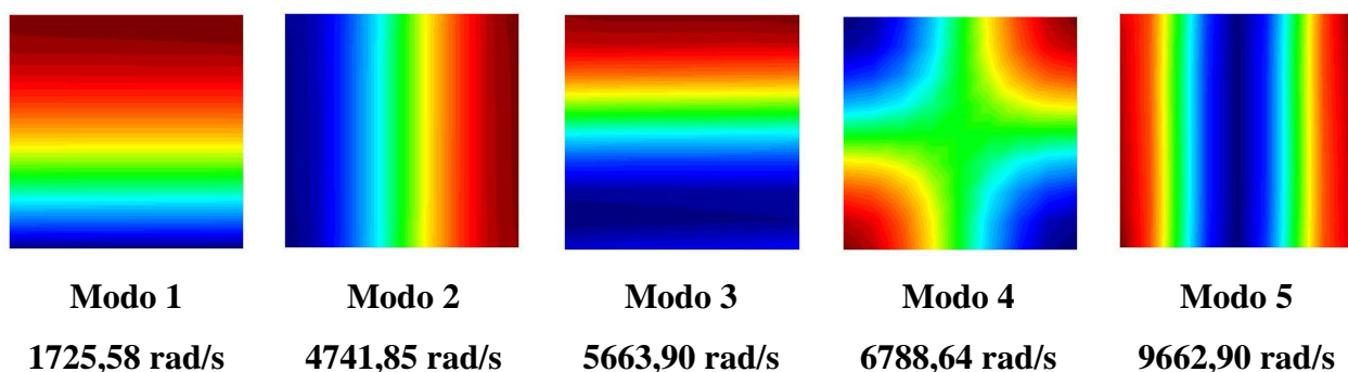
Figura 5.15 – Representação 2D dos cinco primeiros modos acoplados da cavidade fechada fornecidos pelo FEDYFE
