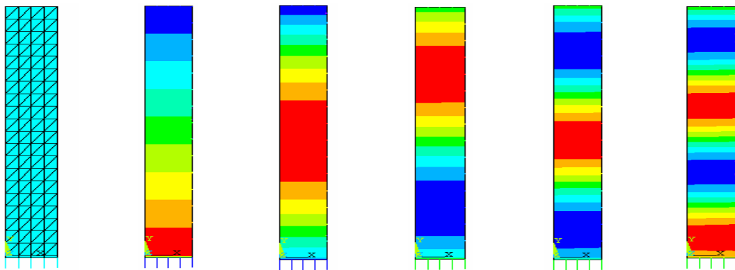
Figura 5.3 – Malha 3 e os cinco primeiros modos acoplados da cavidade aberta obtidos pelo ANSYS.
