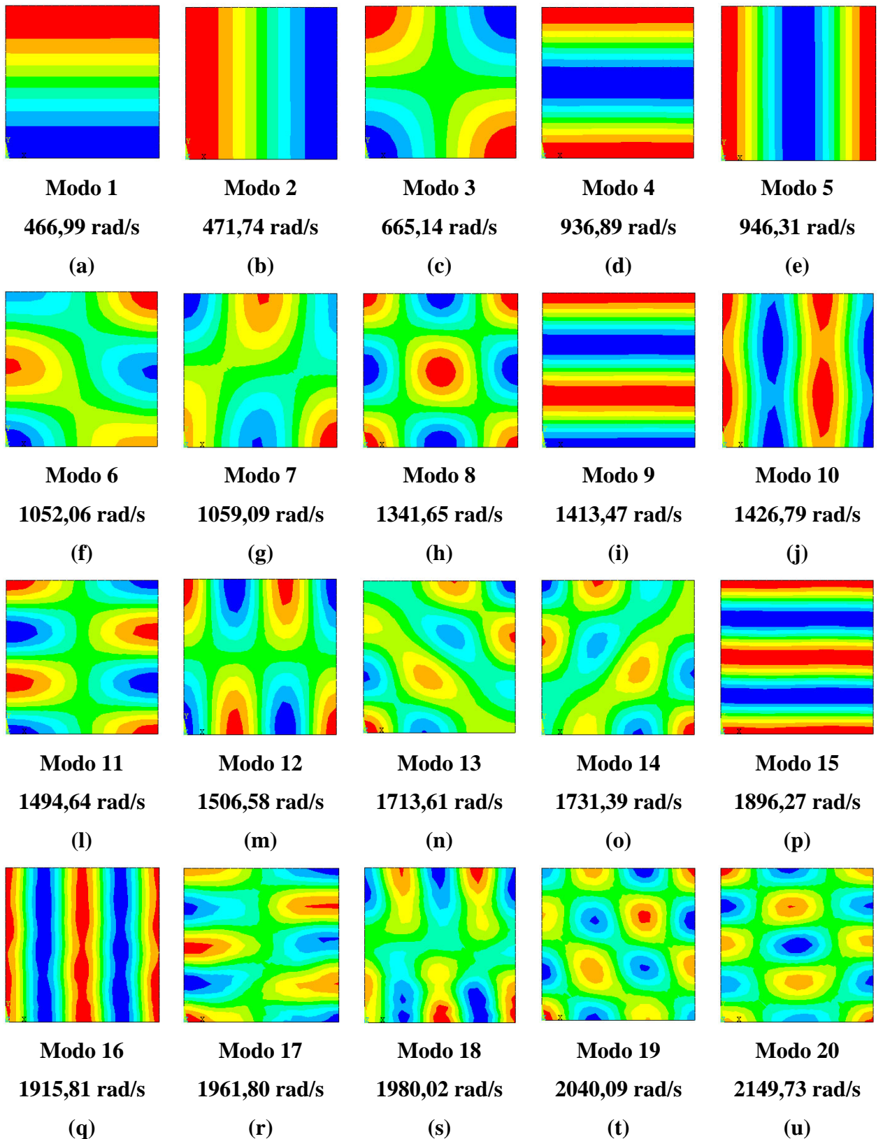
Figura 6.18 – Representação 2D dos modos acoplados da cavidade fechada obtidos via ANSYS com módulo de elasticidade para viga E=2.1 \times 10^{15} \text{N/m}^2 .
