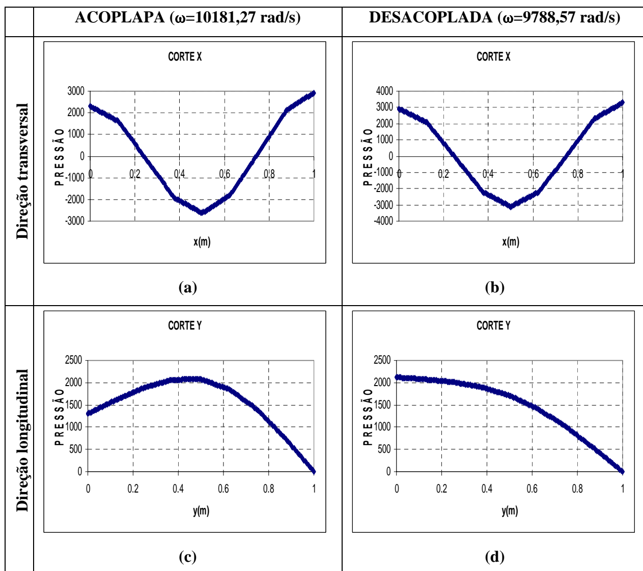
Figura B.15 – Cortes nas direções transversais e longitudinais da cavidade; (a) Corte em x do modo 9, Figura 4.14-(i), (b) Corte em y do modo 9, Figura 4.14-(i), (c) Corte em x do modo 5, Figura 4.12-(e), (d) Corte em y do modo 5, Figura 4.12-(e)
