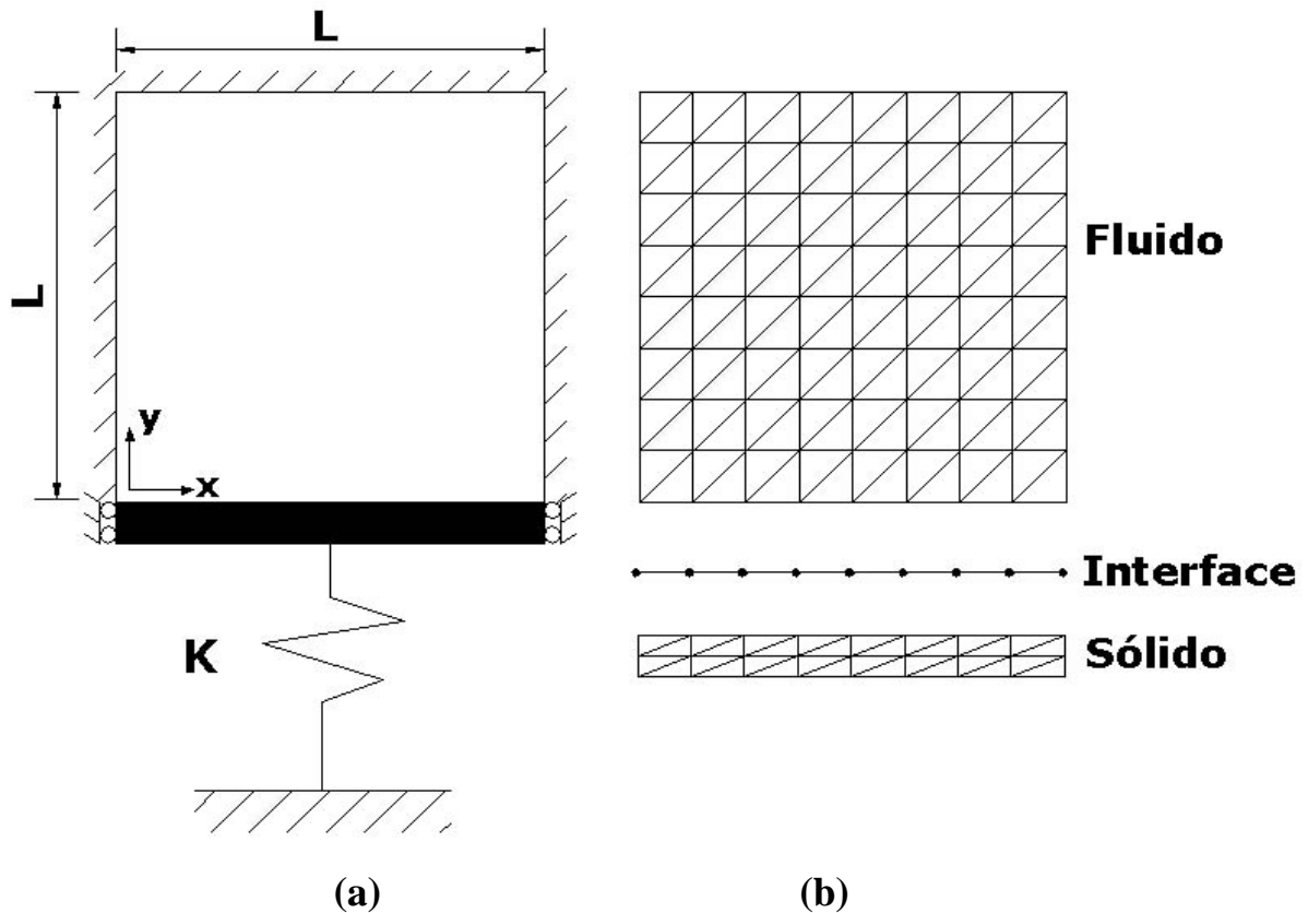
Figura 5.10 – (a) Cavidade rígida curta com extremidade superior fechada. (b) Malha utilizada na discretização.
