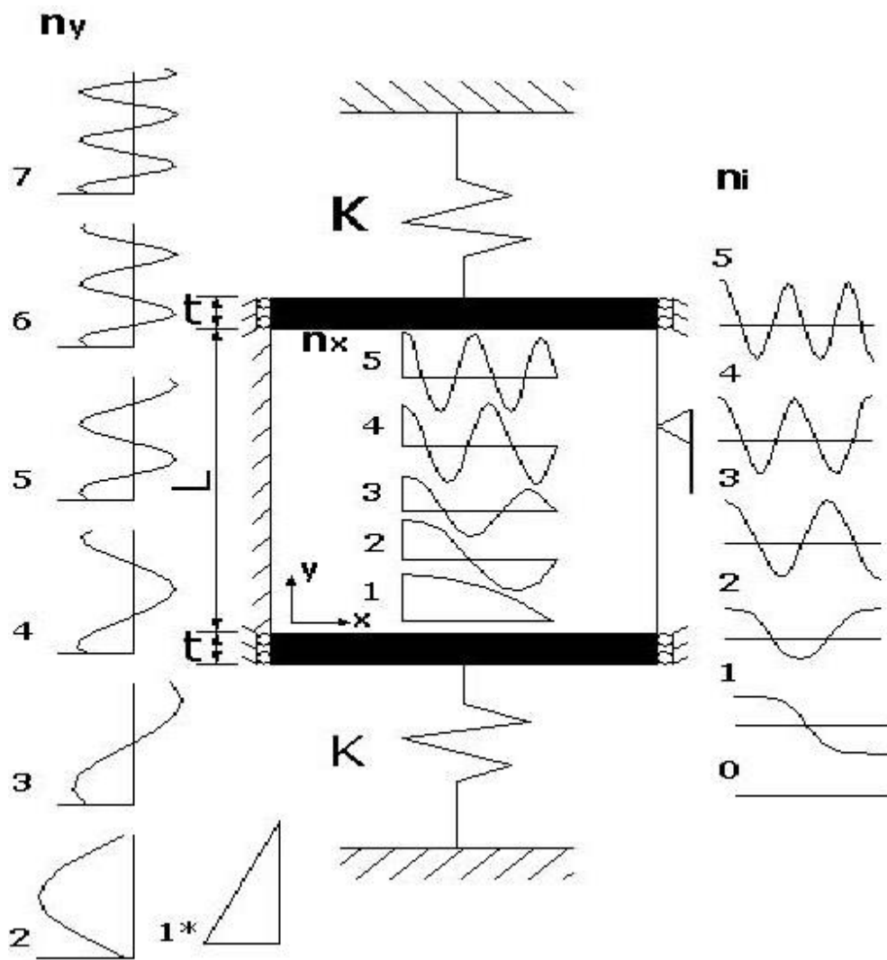
Figura 4.26– Modos típicos transversais e longitudinais da cavidade e da estrutura (caso 2)
