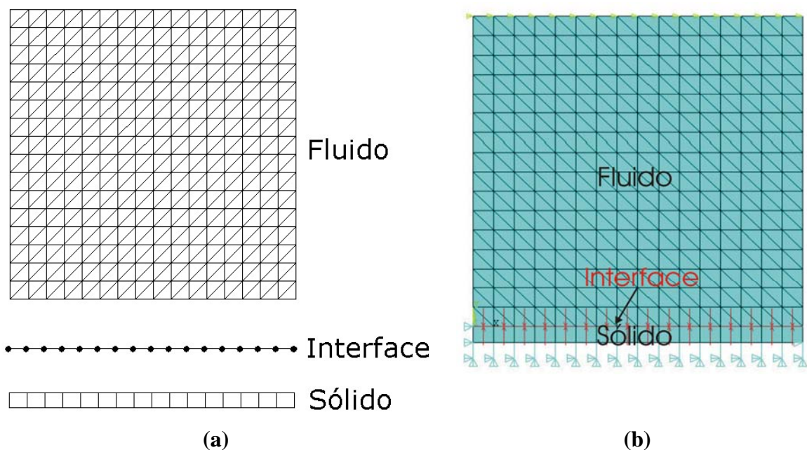
Figura 4.13 – Problema acoplado caso 1; (a) Esquema da malha.(b) Modelo gerado pelo programa ANSYS
