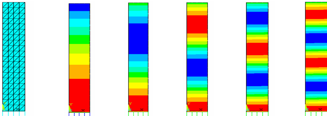
Figura 5.2 – Malha 3 e os cinco primeiros modos desacoplados da cavidade aberta longa obtidos pelo ANSYS.
