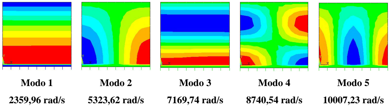
Figura 5.6 – Representação 2D dos cinco primeiros modos desacoplados da cavidade aberta obtidos pelo ANSYS
