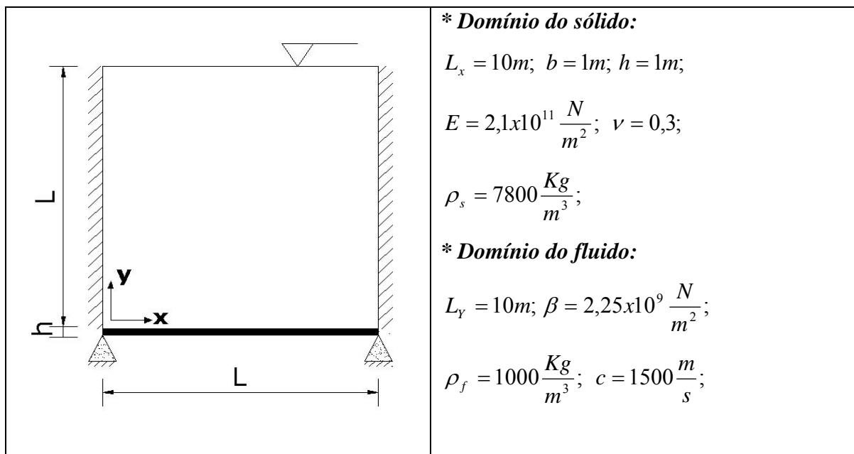
Figura 6.1 – Modelo de uma viga biapoiada com reservatório 2D para condição de contorno aberta
