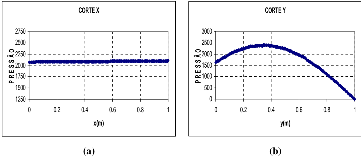
Figura B.6 – Cortes na cavidade para o modo 4, Figura 4.14-(d); (a) Corte x - primeiro modo desacoplado para a cavidade fechada-fechada (b) Corte y - segundo modo acoplado para cavidade aberta.
