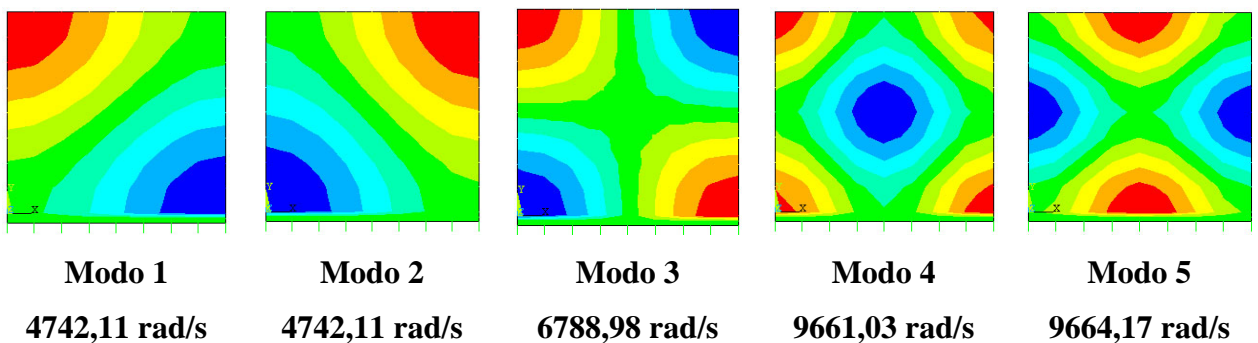
Figura 5.11 – Representação 2D dos modos desacoplados da cavidade fechada obtidos pelo ANSYS (com instabilidade)
