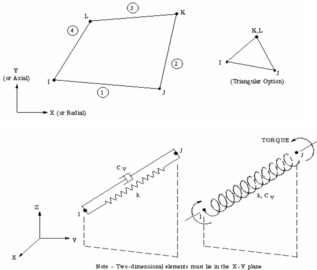
Figura 4.2 – Esquema dos elementos utilizados da biblioteca do ANSYS.
