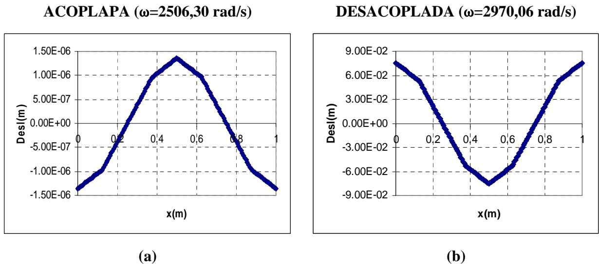
Figura B.4 – Formais modais da estrutura;(a) modo acoplado da Figura 4.14-(c), (b) modo desacoplado da estrutura, ver Figura 4.7.
