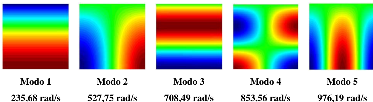
Figura 6.10 – Representação 2D dos modos de vibração da cavidade aberta desacoplada para o caso da viga apoiada obtidos pelo programa FEDYFE
