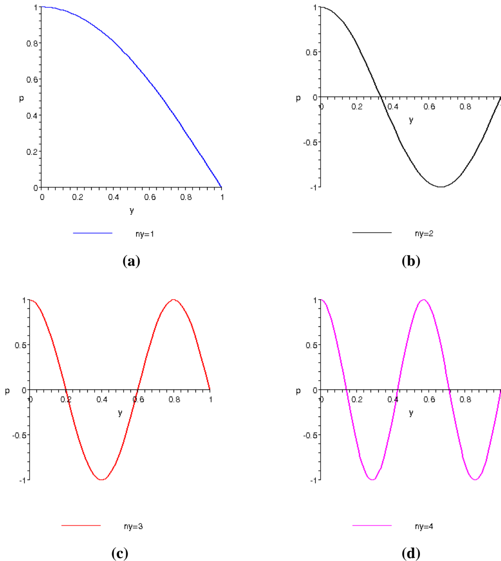
Figura 4.9 – Modos acústicos desacoplados para condição de contorno aberta referentes à solução analítica: (a) 1º, (b) 2º, (c) 3º e (d) 4º Modo.
