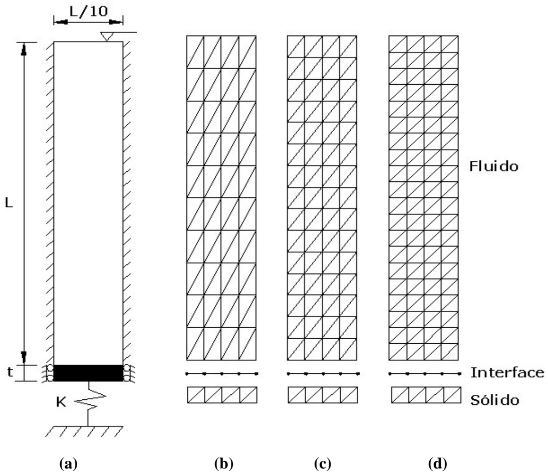
Figura 5.1 – (a) Cavidade rígida longa com extremidade superior aberta. (b), (c) e (d) Diferentes malhas utilizadas na discretização, Barbosa (1998)
