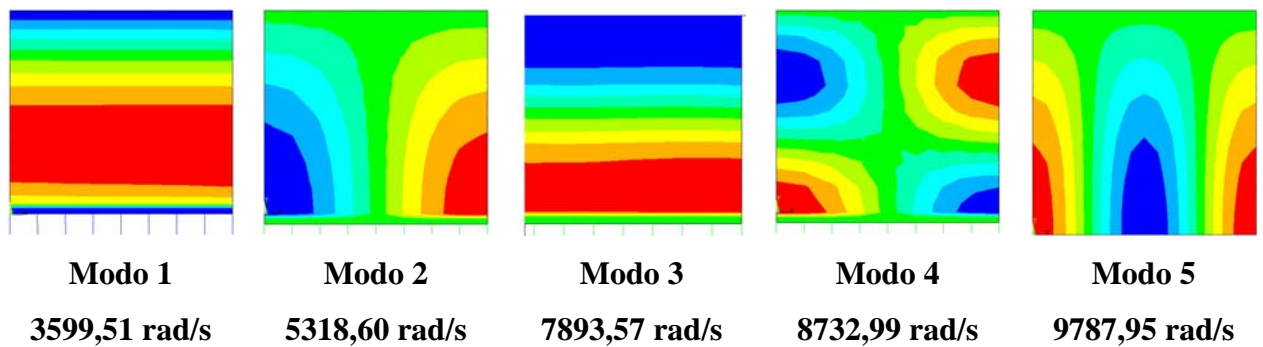
Figura 5.8 – Representação 2D dos cinco primeiros modos acoplados da cavidade aberta obtidos pelo ANSYS
