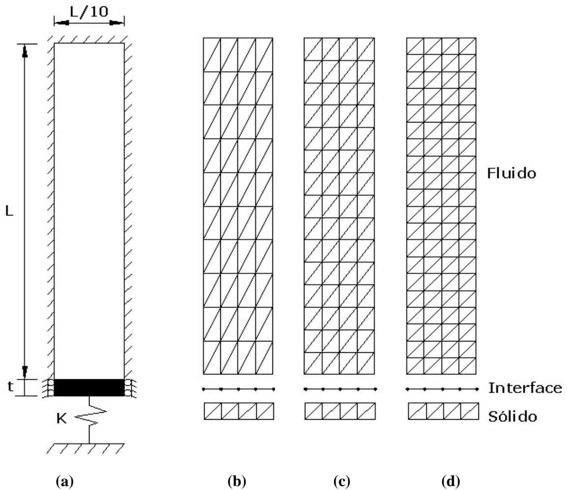
Figura 5.4 – (a) Cavidade rígida longa com extremidade superior fechada. (b)-(d) Malhas utilizadas na discretização.
