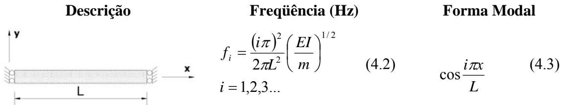
Figura 4.5 – Esquema da estrutura sem apoio elástico
