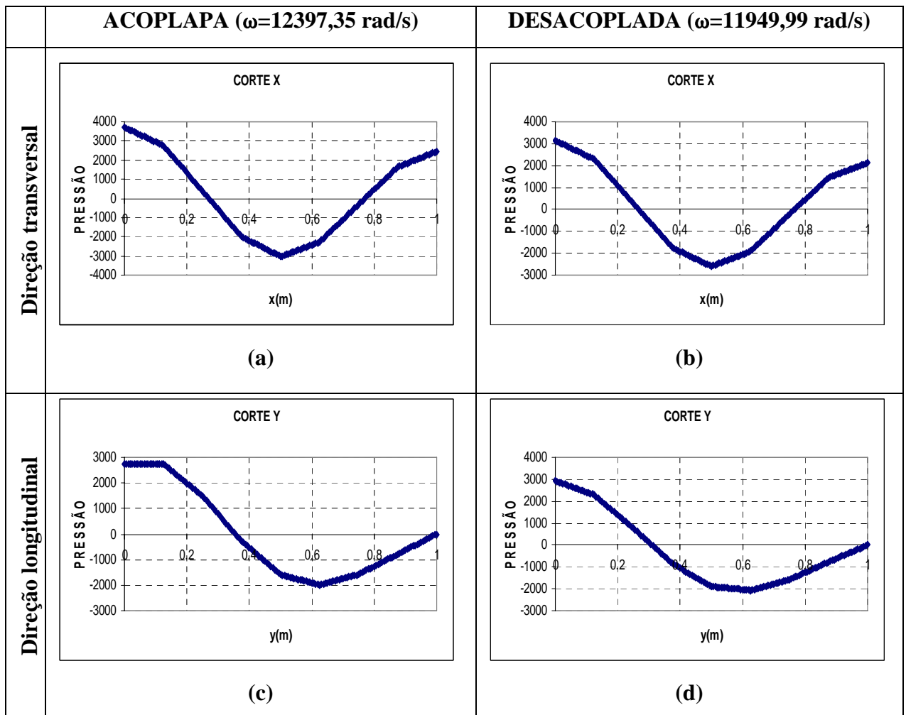
Figura B.20 – Cortes nas direções transversais e longitudinais da cavidade; (a) Corte em x do modo 12, Figura 4.14-(m), (b) Corte em y do modo 12, Figura 4.14-(m), (c) Corte em x do modo 7, Figura 4.12-(g), (b) Corte em y do modo 7, Figura 4.12-(g)
