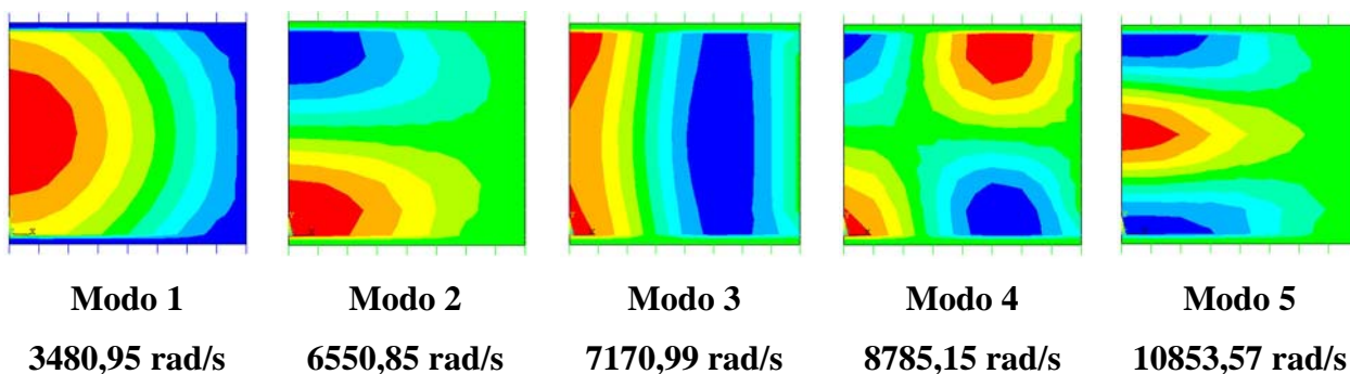
Figura 5.19 – Representação 2D dos modos acoplados da cavidade aberta com 2 placas móveis obtidos pelo ANSYS
