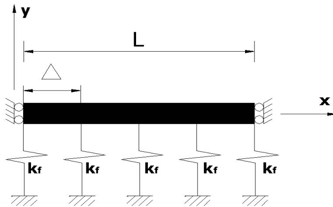
Figura 4.4 – Esquema da estrutura (pistão) sobre base elástica
