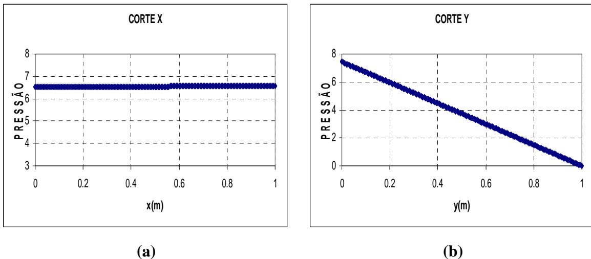
Figura 4.15 – Cortes da cavidade obtidos via ANSYS; (a) Corte x - primeiro modo desacoplado para a cavidade fechada-fechada (b) Corte y - primeiro modo acoplado para cavidade aberta.
