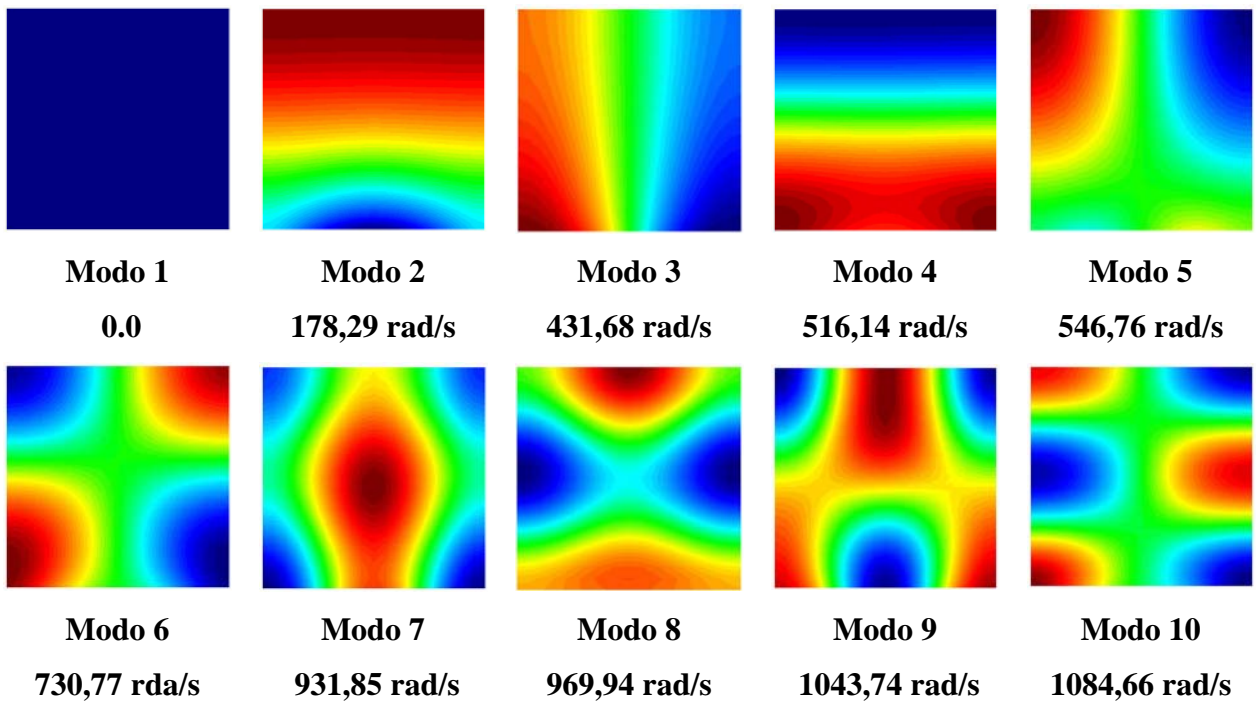
Figura 6.19 – Representação 2D dos modos acoplados da cavidade fechada para o caso da viga apoiada obtidos pelo FEDYFE
