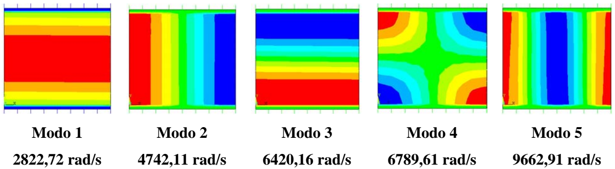
Figura 5.22 – Representação 2D dos modos acoplados da cavidade fechada com 2 placas móveis obtidos via ANSYS
