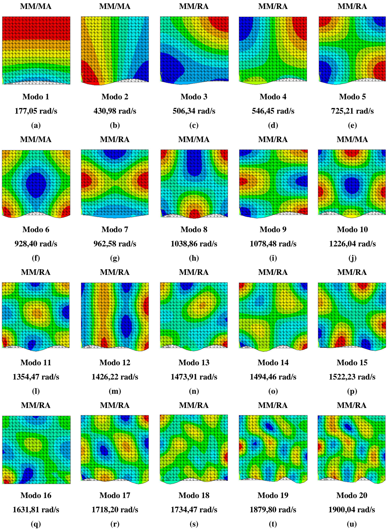
Figura 6.17 – Representação 2D dos modos acoplados da cavidade fechada obtidos via ANSYS com módulo de elasticidade E=2.1 \times 10^{11} \text{N/m}^2 .
