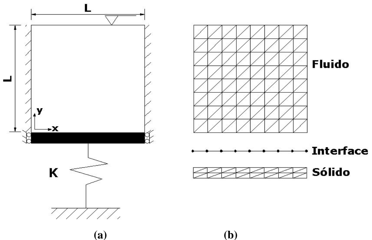
Figura 5.5 – (a) Cavidade rígida curta com extremidade superior aberta. (b) Malha utilizada na discretização.
