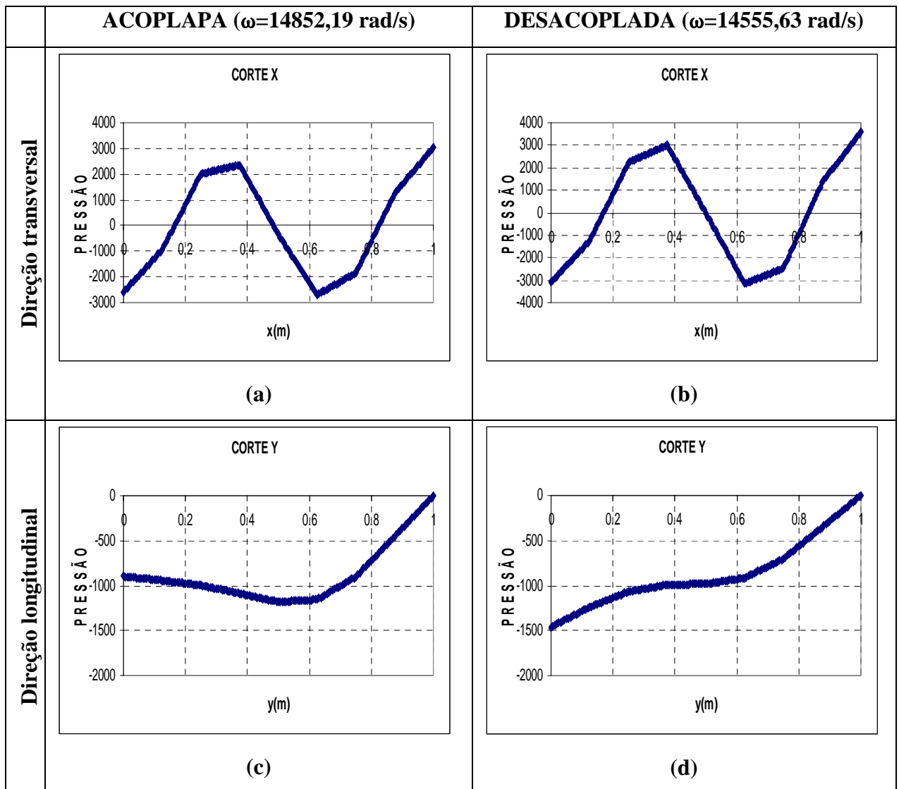
Figura B.24 – Cortes nas direções transversais e longitudinais da cavidade; (a) Corte em x do modo 14, Figura 4.14-(o), (b) Corte em y do modo 9, Figura 4.14-(o), (c) Corte em x para o modo 9, Figura 4.12-(i), (d) Corte em y do modo 9, Figura 4.12-(i)
