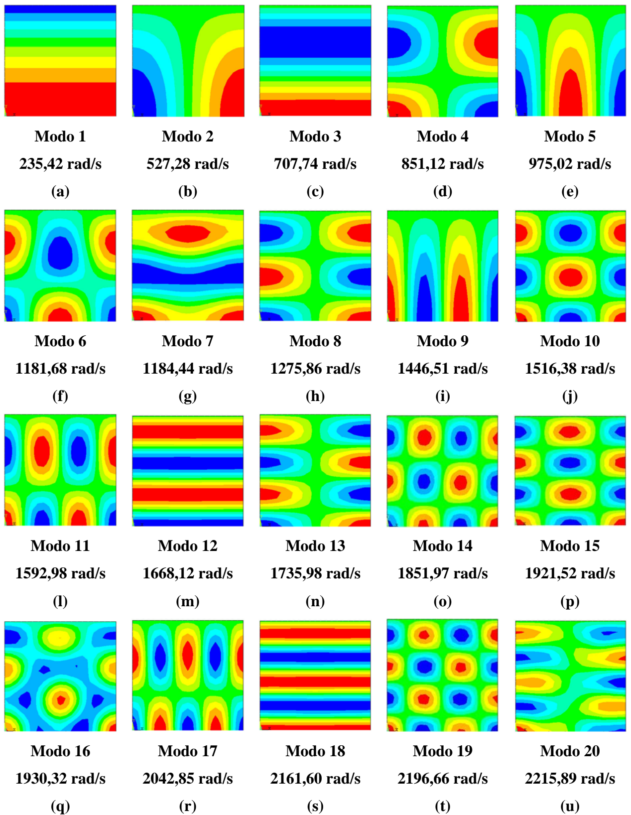
Figura 6.9 – Representação 2D dos modos acoplados da cavidade aberta obtidos via ANSYS com módulo de elasticidade para viga E=2.1 \times 10^{15} \text{N/m}^2 .
