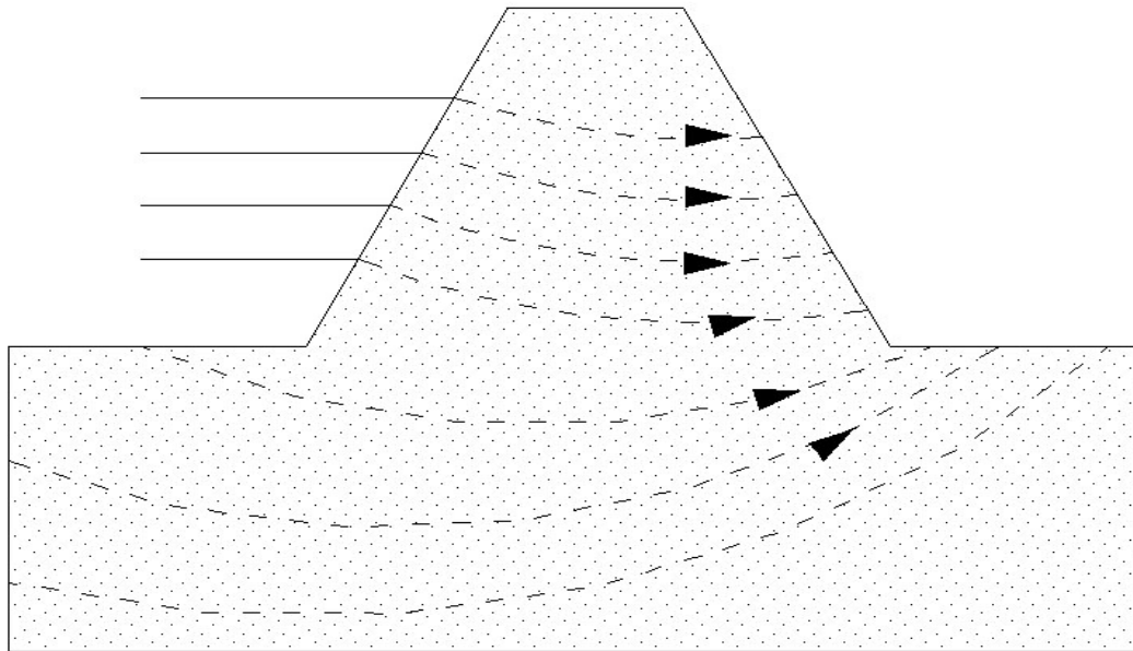
Figura 1.4 – Classe II – Percolação por meios porosos, Zienkiewicz & Taylor (1989)
