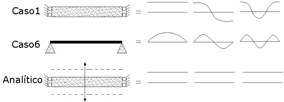
Figura 6.7 – As diferenças entre as deformadas modais do sólido.
