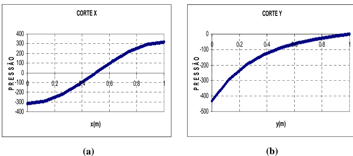
Figura B.3 – Cortes na cavidade do modo 2, Figura 4.14-(b); (a) Corte em x (b) Corte em y
