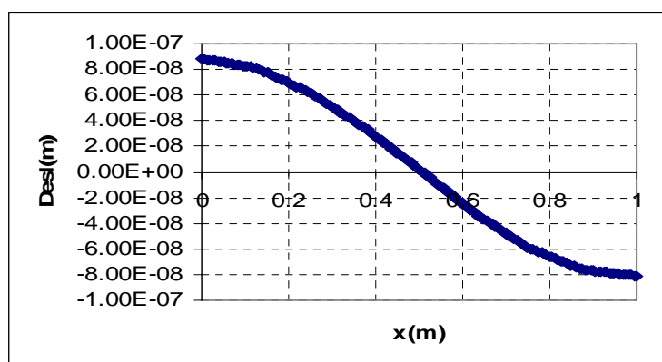
Figura B.12 – Forma modal da estrutura para o caso acoplado da Figura 4.14-(h)
