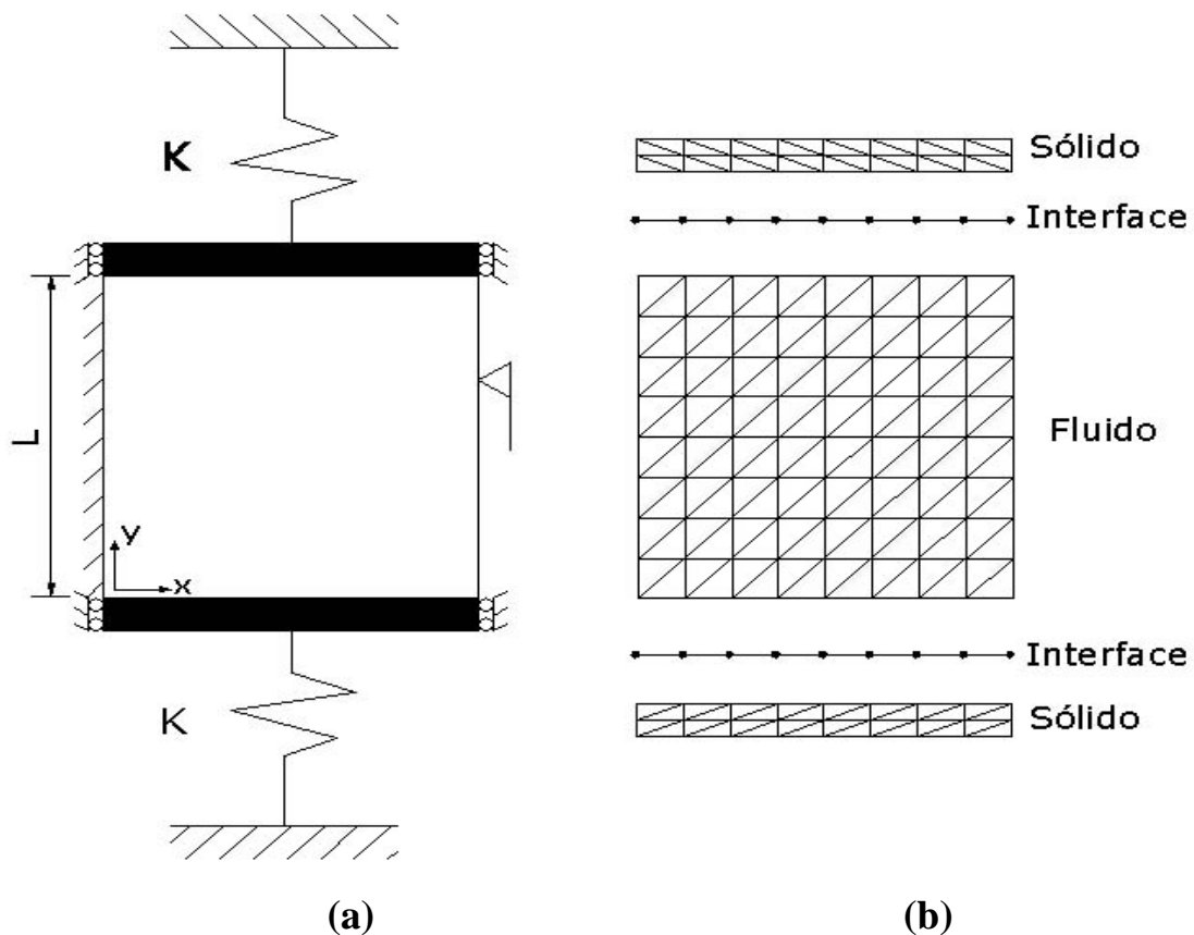
Figura 5.16 – (a) Cavidade rígida curta aberta com duas placas móveis. (b) Malha utilizada na discretização.
