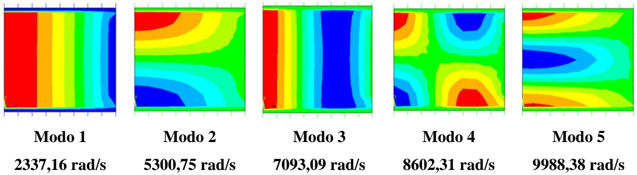
Figura 5.17 – Representação 2D dos modos desacoplados da cavidade aberta com 2 placas móveis obtidos pelo ANSYS
