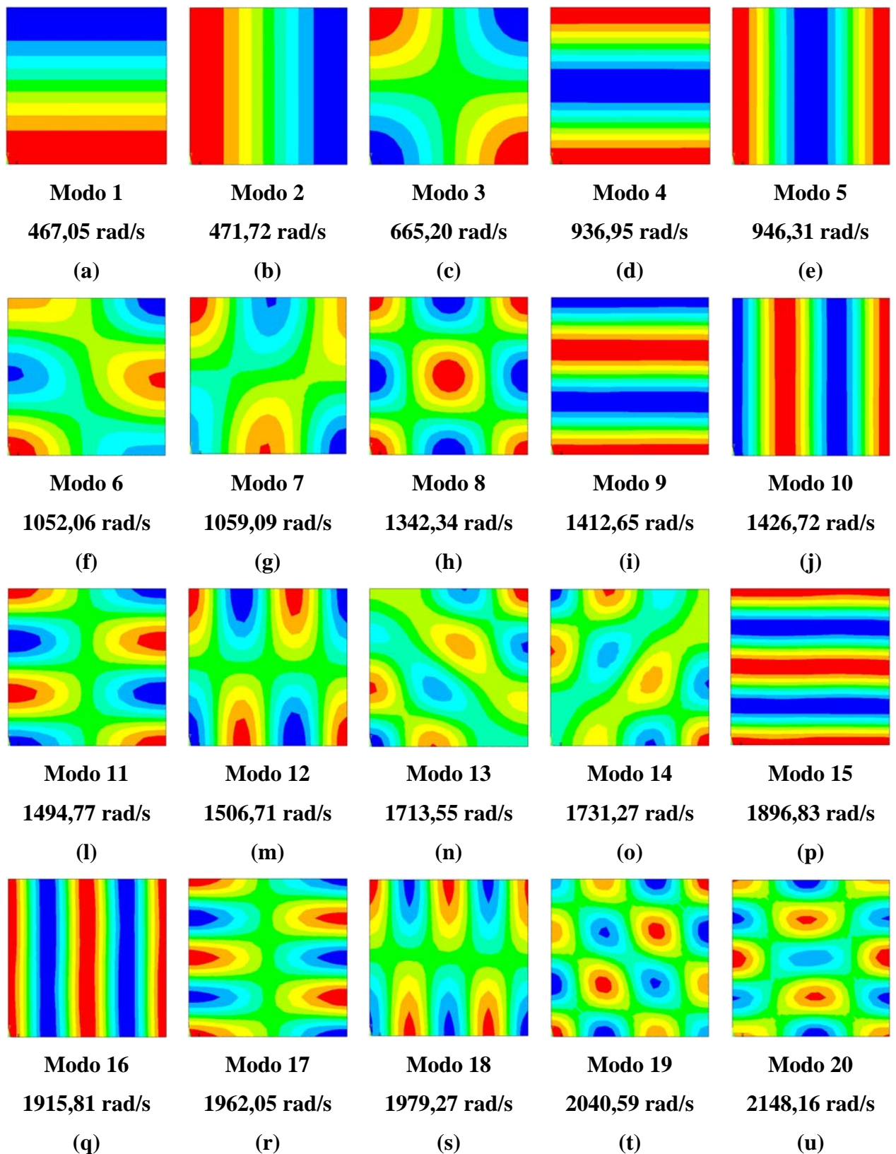
Figura 6.15 – Representação 2D dos modos desacoplados da cavidade fechada obtidos via ANSYS
