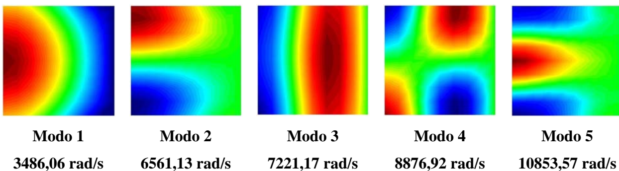
Figura 5.20 – Representação 2D dos modos acoplados da cavidade aberta com 2 placas móveis obtidos pelo FEDYFE
