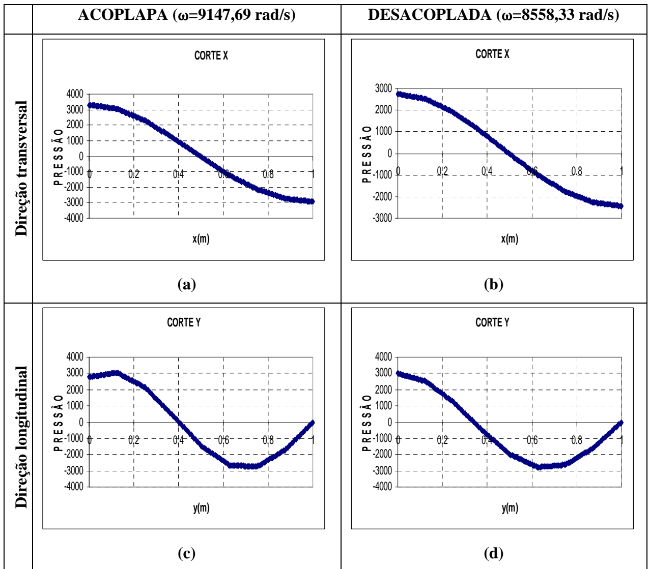
Figura B.13 – Cortes nas direções transversais e longitudinais da cavidade; (a) Corte em x do modo 8, Figura 4.14-(h), (b) Corte em y do modo 8 -Figura 4.14-(h), (c) Corte em x do modo 4, Figura 4.12-(d), (b) Corte em y do modo 4, Figura 4.12-(d).
