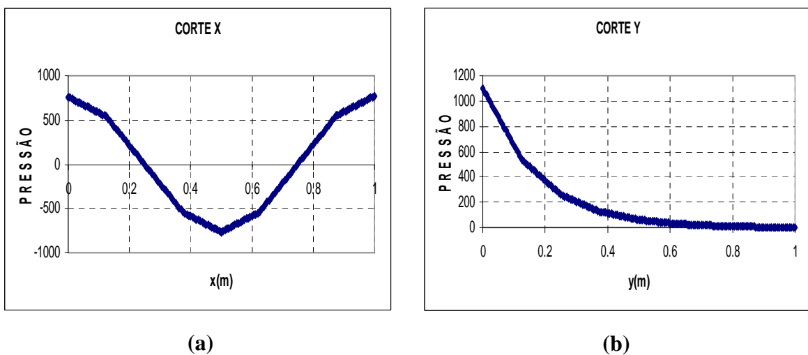
Figura B.5 – Cortes na cavidade para o modo 3, Figura 4.14-(c); (a) Corte na direção (x), (b) Corte na direção (y)
