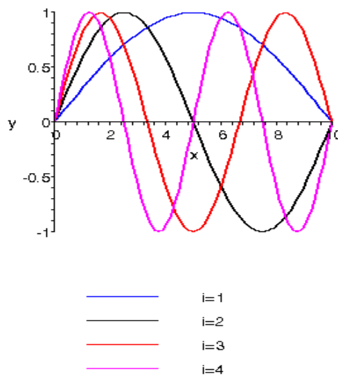
Figura 6.2 – Deformadas analíticas desacopladas dos modos naturais da viga biapoiada
