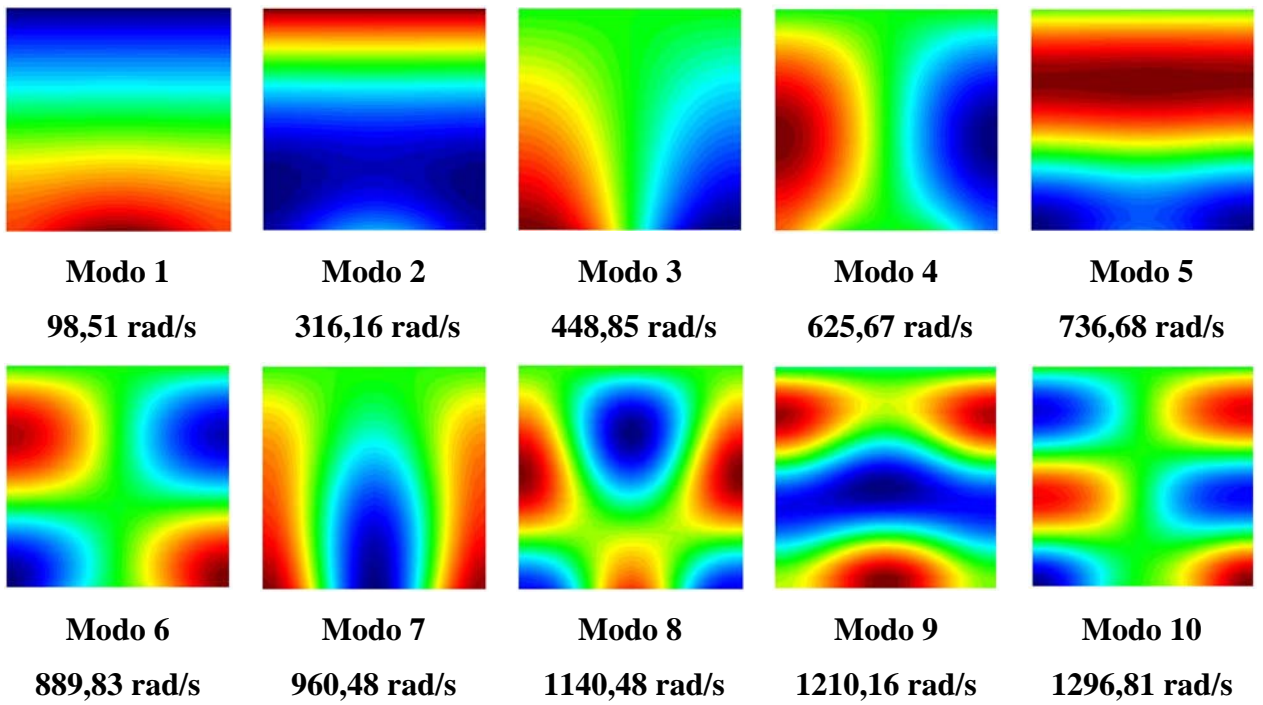
Figura 6.12 – Representação 2D dos modos acoplados da cavidade aberta do caso da viga apoiada obtidos pelo FEDYFE
