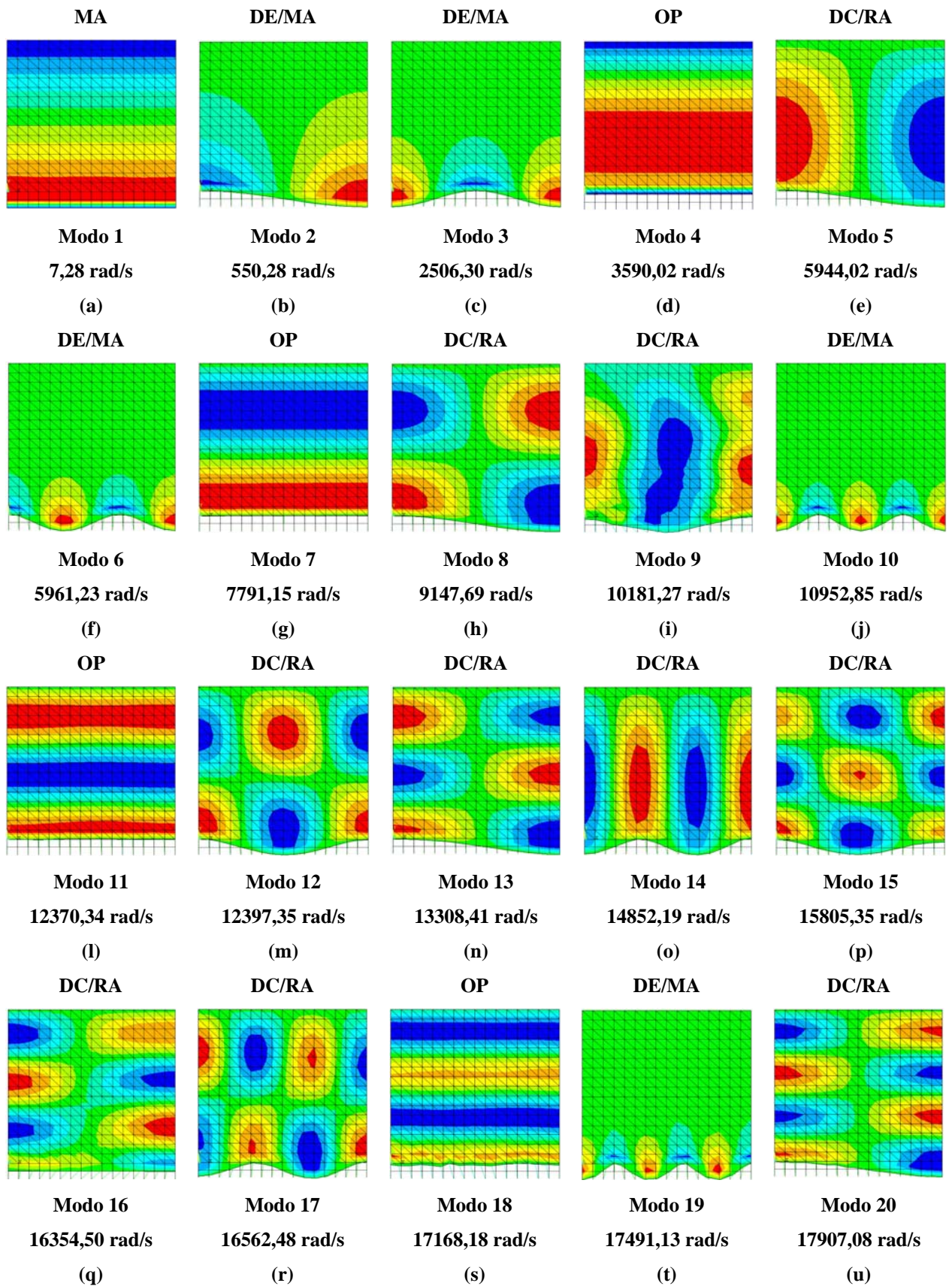
Figura 4.14 – Representação 2D dos modos acoplados da cavidade aberta obtidos via ANSYS com módulo de elasticidade E=2.1 \times 10^{11} \text{N/m}^2 .
