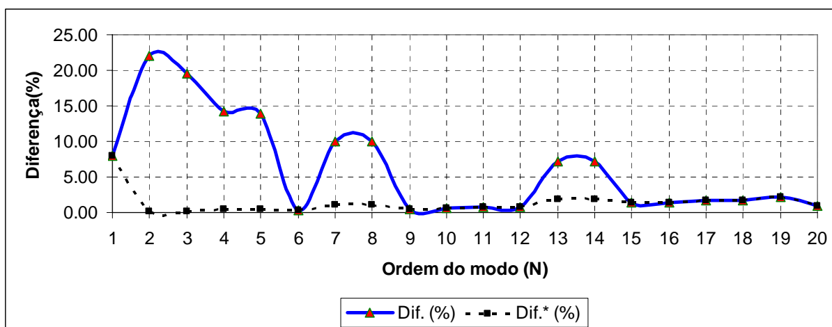
Figura 4.27 – Ordem do modo x Diferença (%)
