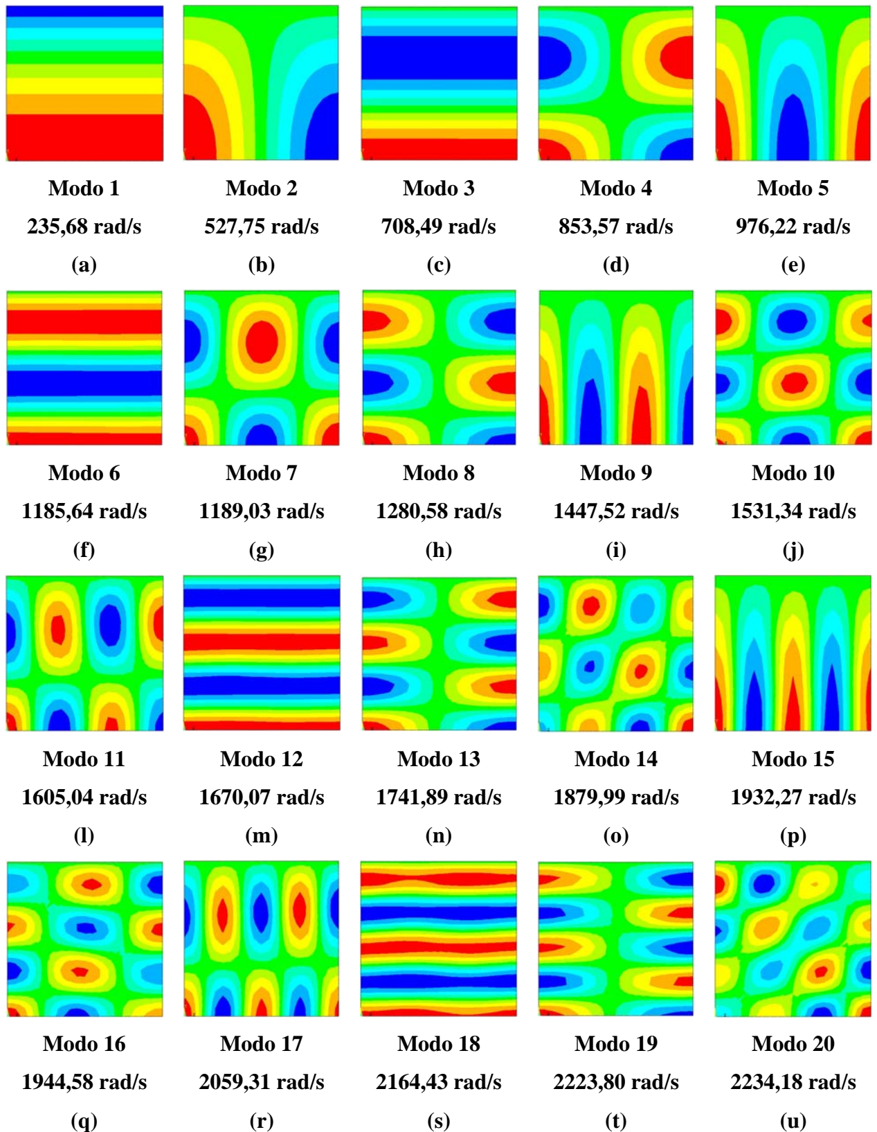
Figura 6.4 – Representação 2D dos modos desacoplados da cavidade aberta obtidos via ANSYS
