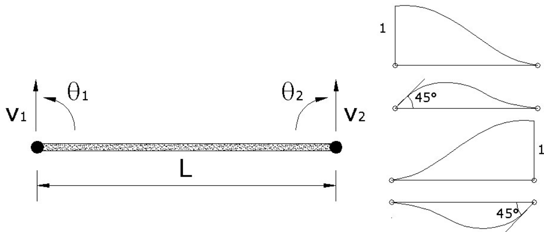
Figura 3.4 – Elemento de viga de Bernoulli e suas funções de forma.
