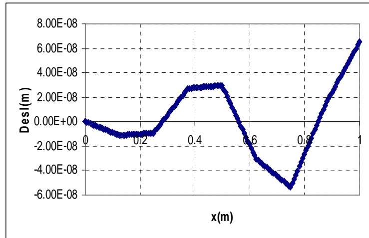
Figura B.23 – Forma modal da estrutura para o modo acoplado da Figura 4.14-(o).
