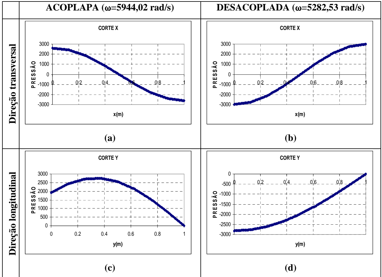
Figura B.8 – Cortes em x e y da cavidade; (a) Corte em x para o modo acoplado 5, Figura 4.14-(e), (b) Corte em y para o modo acoplado 5, Figura 4.14-(e), (c) Corte em x para o modo desacoplado 2, Figura 4.12-(b), (b) Corte em y para o modo desacoplado 2, Figura 4.12-(b)
