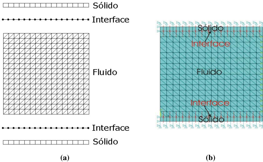
Figura 4.23 –(a) Esquema da malha para o caso 2 (b) Modelo gerado no programa ANSYS
