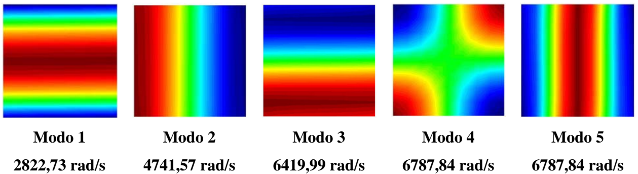
Figura 5.23 – Representação 2D dos modos desacoplados da cavidade fechada com 2 placas móveis obtidos via FEDYFE
