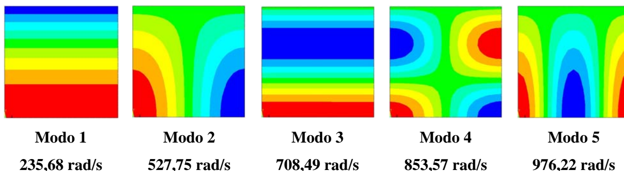
Figura 6.11 – Representação 2D dos modos desacoplados da cavidade aberta do caso da viga apoiada obtidos pelo ANSYS
