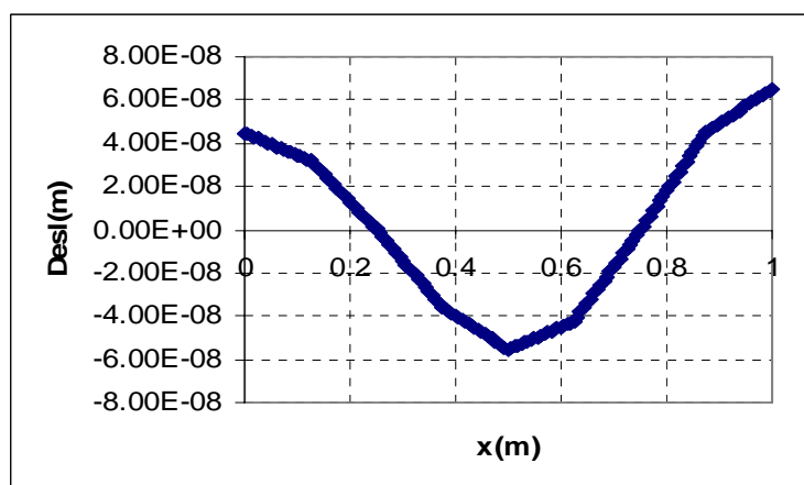
Figura B.14- Forma modal da estrutura para o modo acoplado da Figura 4.14-(i)
