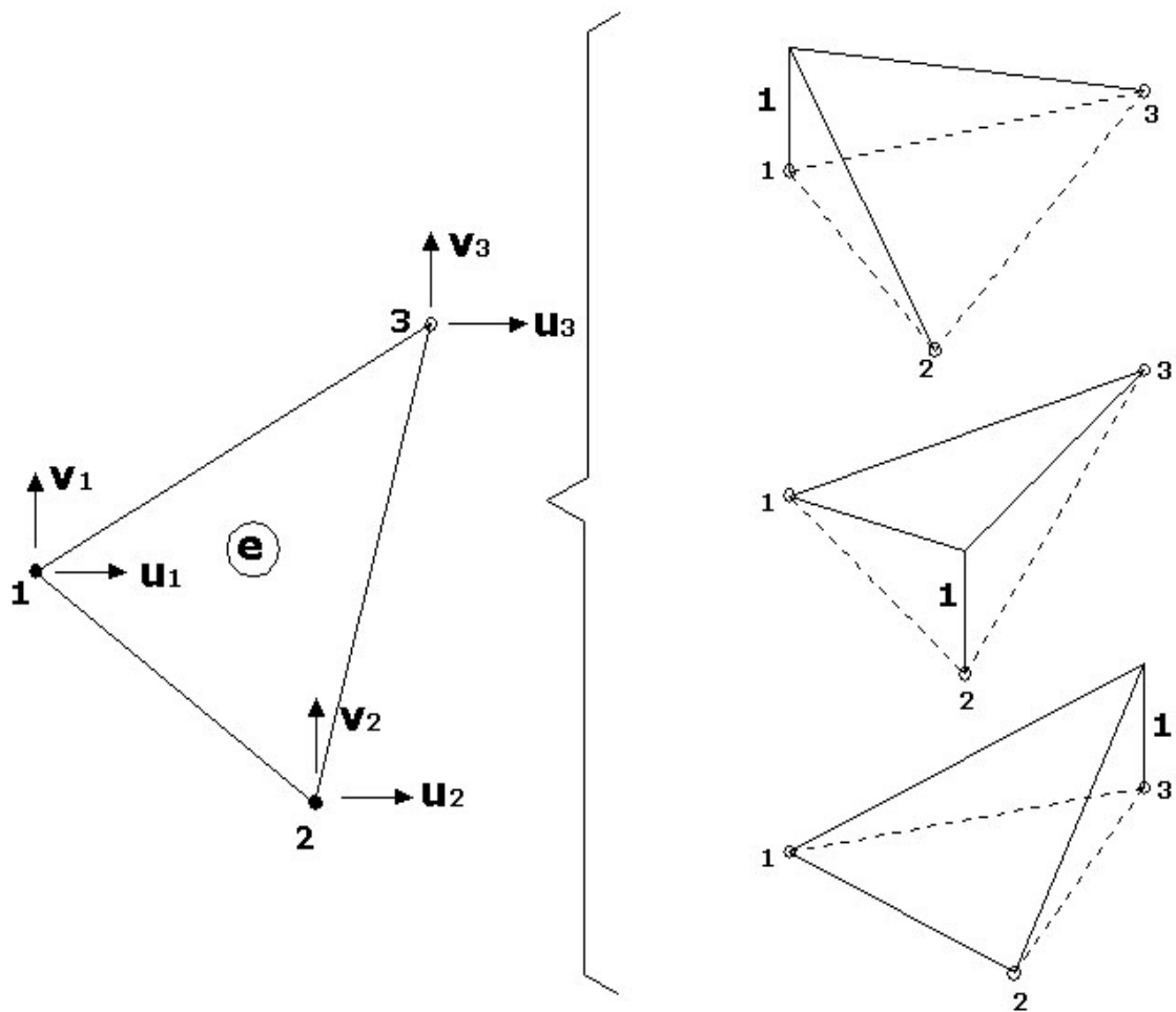
Figura 3.3 –Funções de forma para o elemento triangular de três nós
