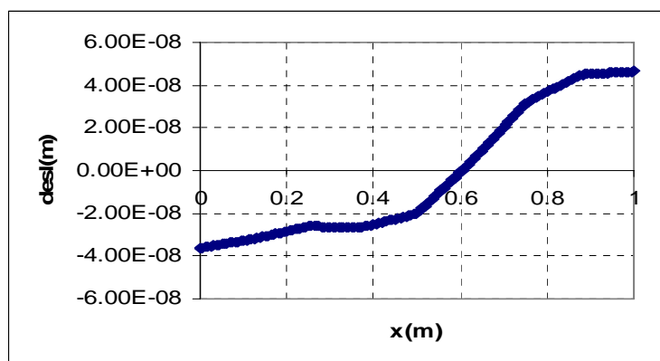
Figura B.21 – Forma modal da estrutura para o modo acoplado da Figura 4.14-(n).
