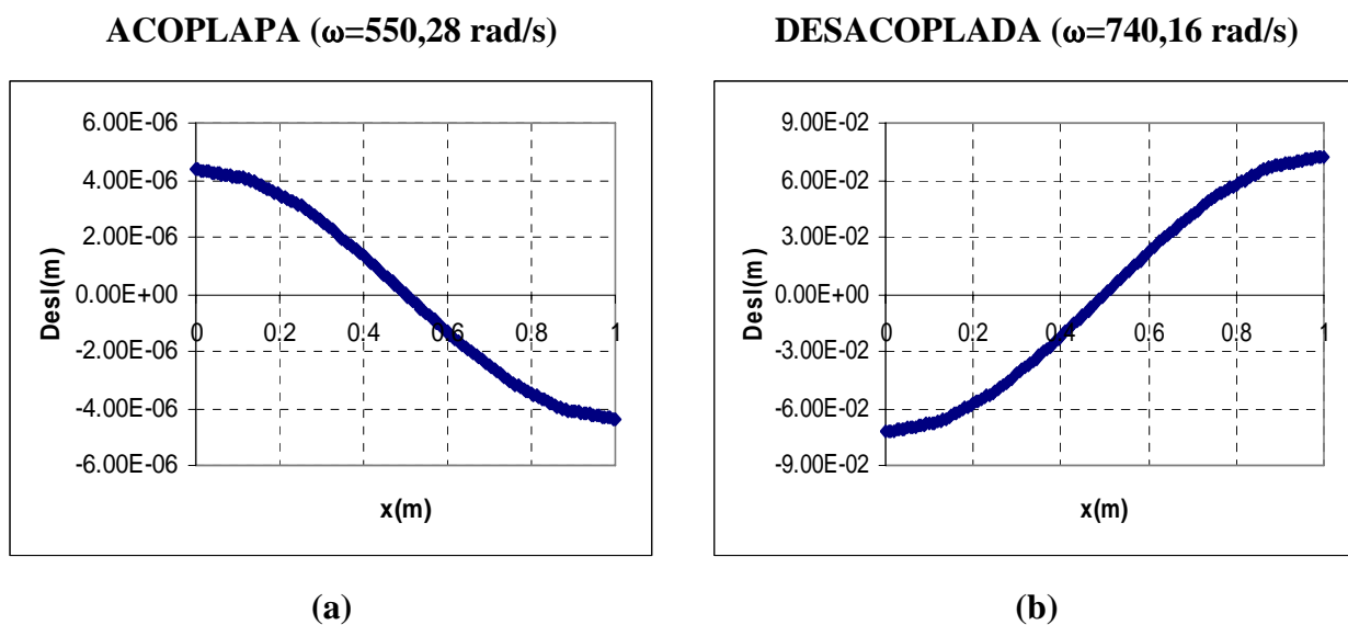
Figura B.2 – Formas modais da estrutura;(a) modo acoplado da Figura 4.14-(b), (b) modo desacoplado da estrutura, ver Figura 4.7.
