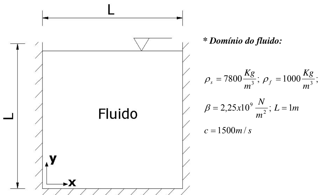
Figura 4.8 – Cavidade rígida curta com extremidade superior aberta
