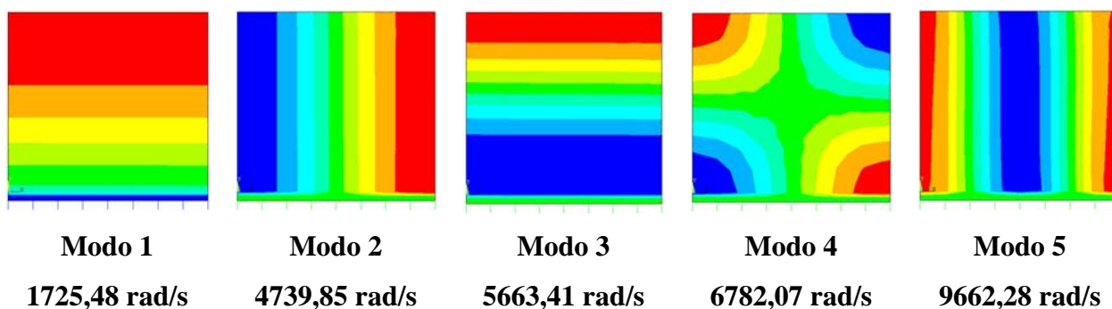
Figura 5.14 – Representação 2D dos cinco primeiros modos acoplados da cavidade fechada fornecidos pelo ANSYS
