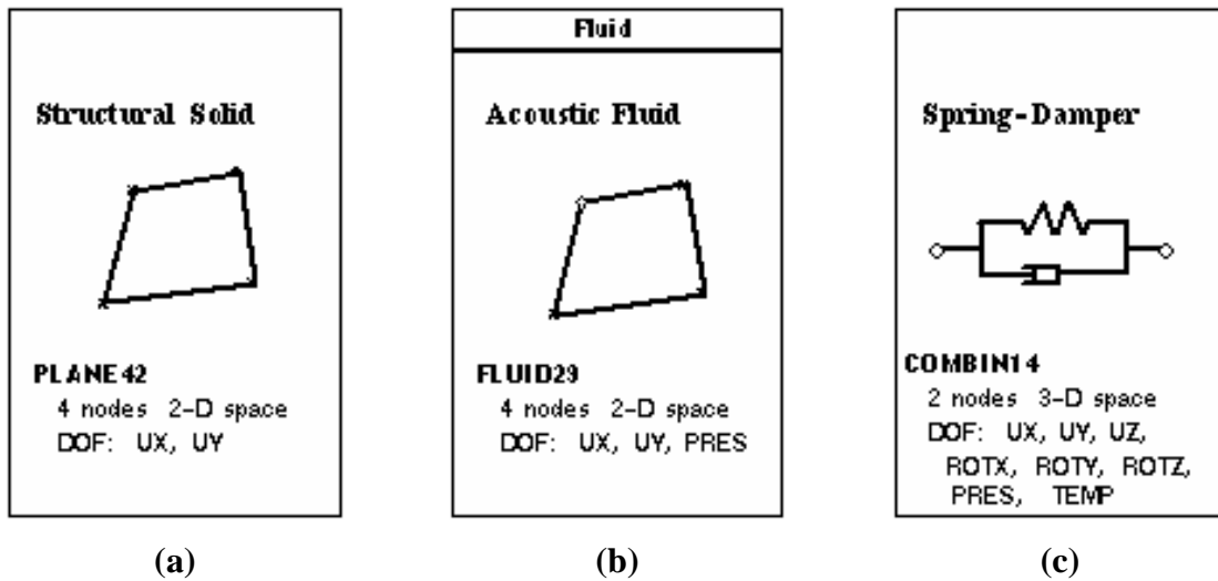
Figura 4.1 – Esquema dos elementos selecionados no ANSYS; (a) Elemento sólido (b) Elemento fluido acústico e (c) Elemento de mola.
