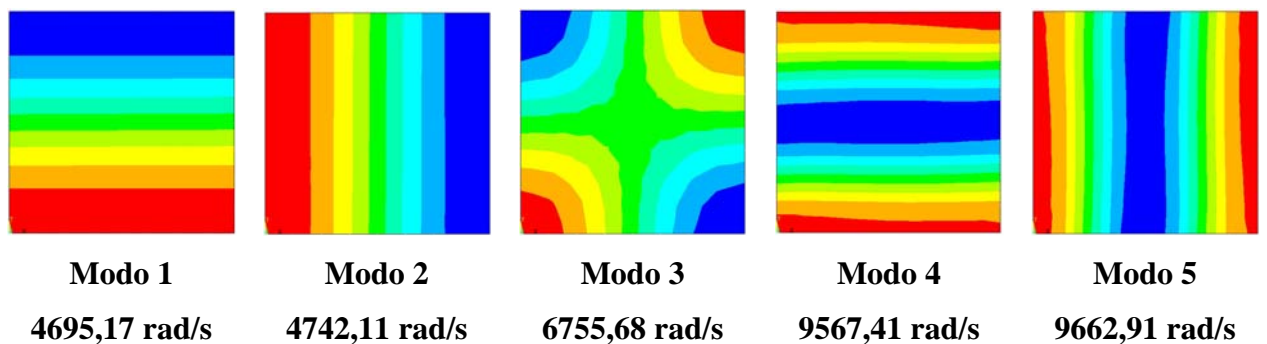
Figura 5.13 – Representação 2D dos modos desacoplados da cavidade fechada obtidos pelo ANSYS (sem instabilidade)
