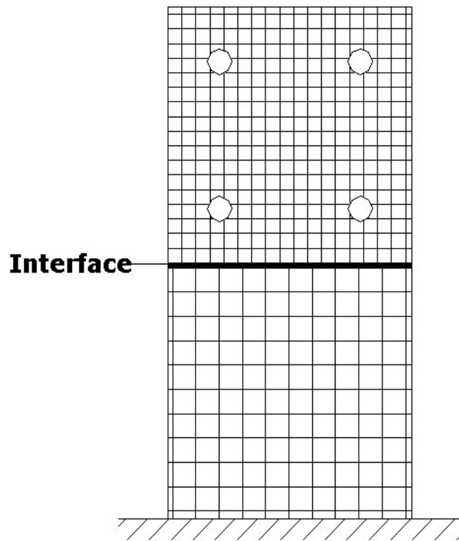
Figura 1.3 – Classe I – Domínios fisicamente idênticos, Zienkiewicz & Taylor (1989)
