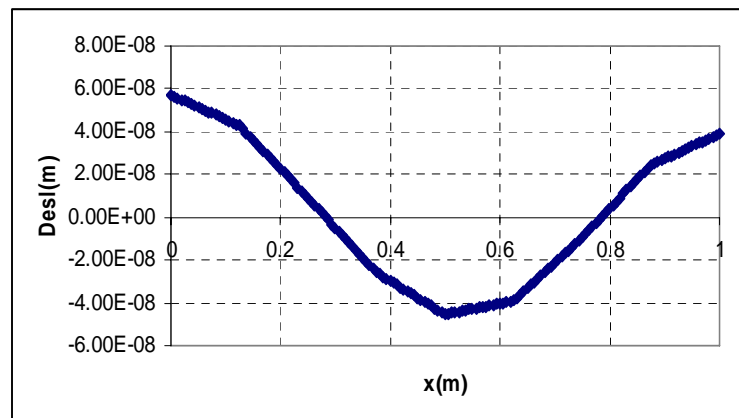
Figura B.19 – Forma modal da estrutura para o modo acoplado da Figura 4.14-(m)
