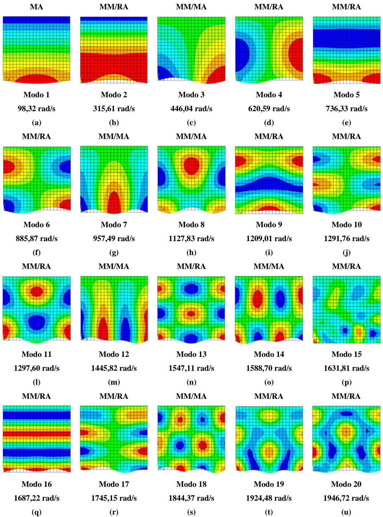
Figura 6.6 – Representação 2D dos modos acoplados da cavidade aberta obtidos via ANSYS com módulo de elasticidade E=2.1 \times 10^{11} \text{N/m}^2 .
