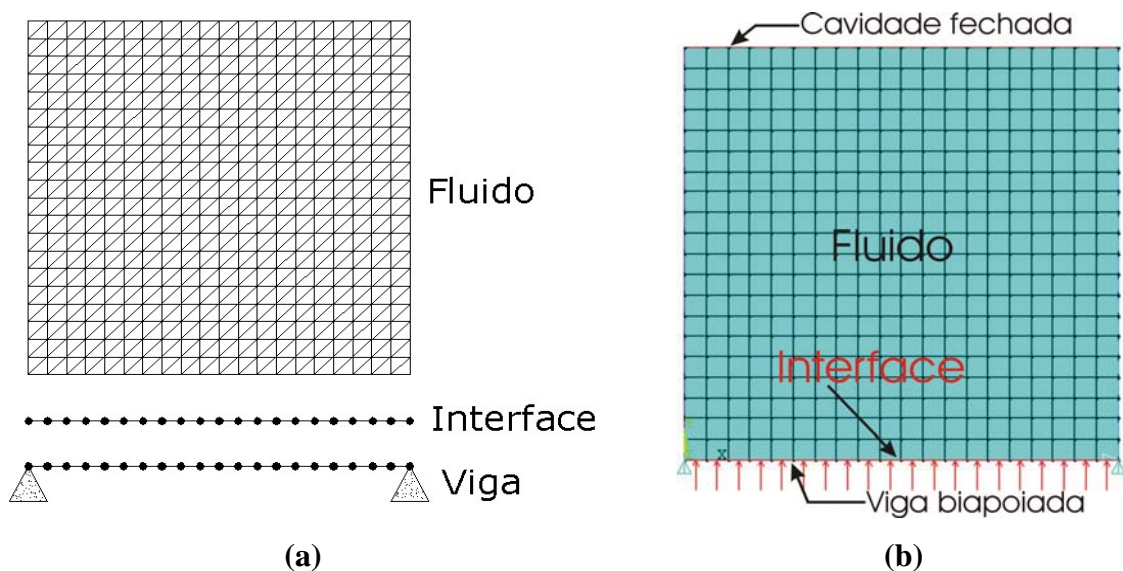
Figura 6.16 – (a) Esquema da malha para o caso da Figura 6.14;(b) Modelo gerado no programa ANSYS
