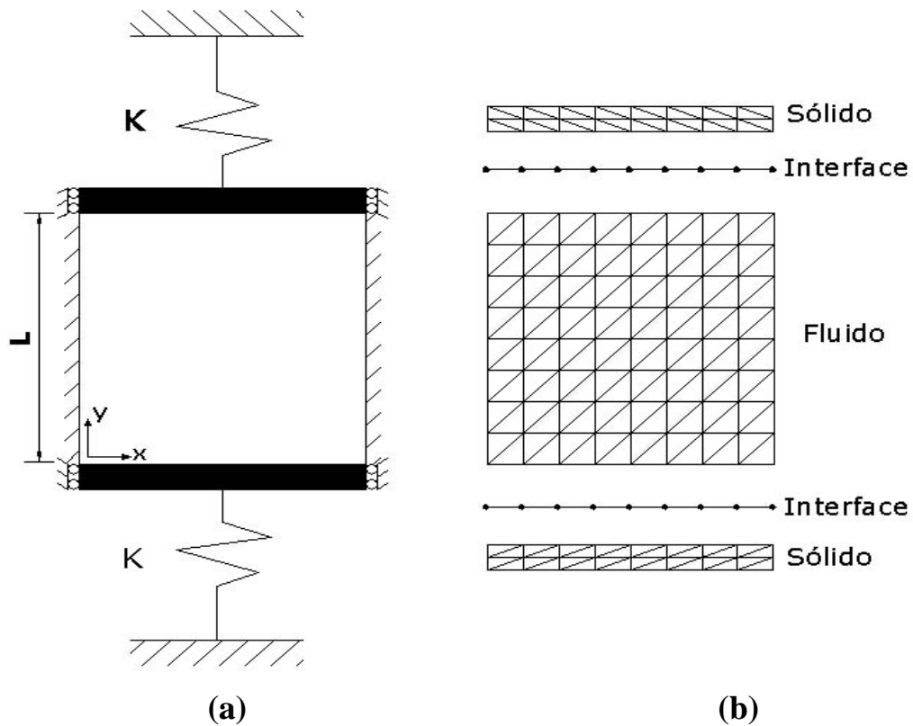
Figura 5.21 – (a) Cavidade rígida curta fechada com duas placas móveis. (b) Malha utilizada na discretização.
