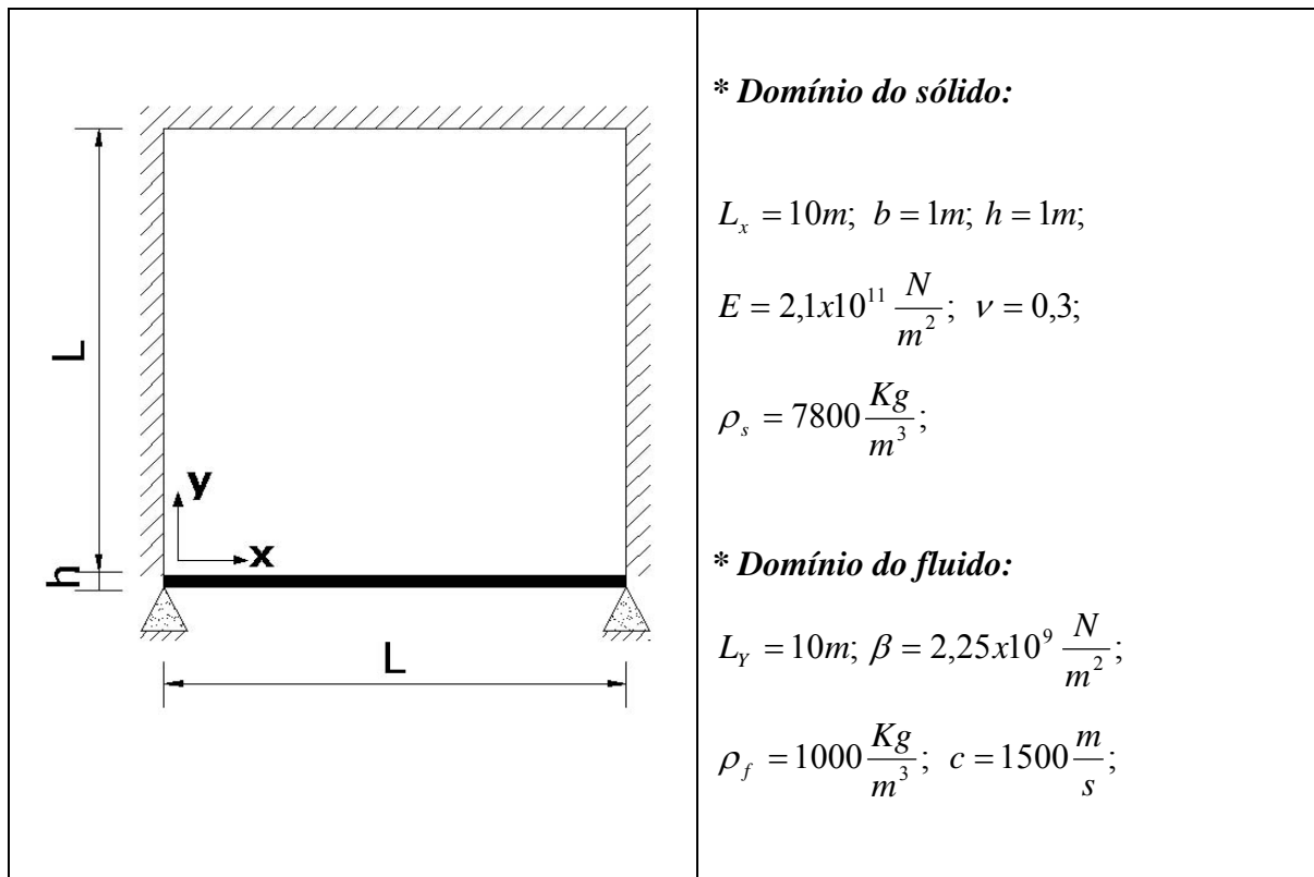
Figura 6.14 – Modelo de uma viga biapoiada com reservatório 2D para condição de contorno da cavidade fechada
