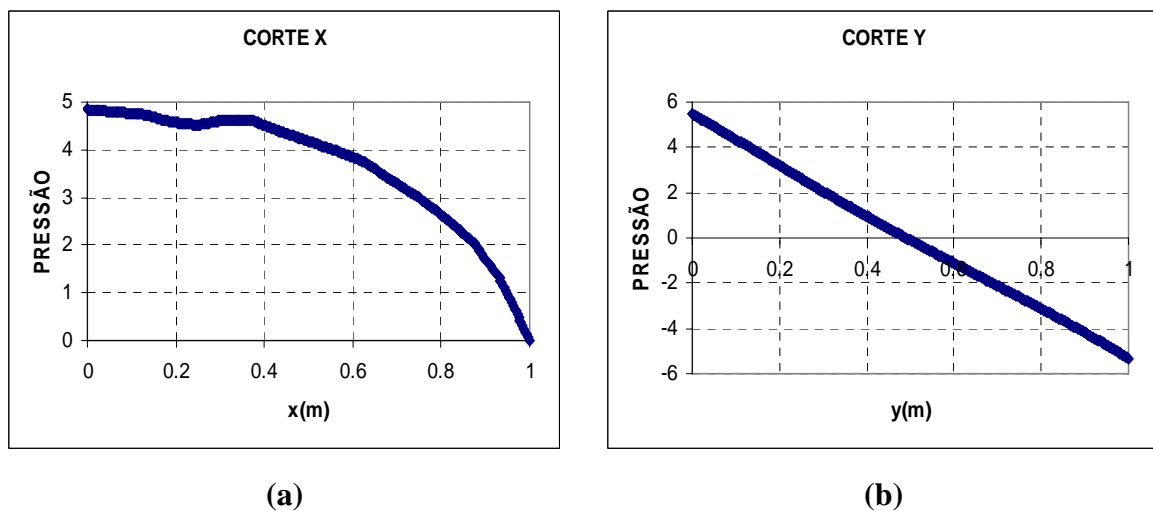
Figura 4.25 – Cortes no modo de massa adicional obtido pelo ANSYS do caso 2; (a) Corte x - primeiro modo desacoplado para a cavidade fechada-aberta (b) Corte y - primeiro modo acoplado
