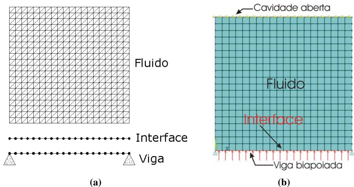
Figura 6.5 – (a) Esquema da malha para o caso da Figura 6.1; (b) Modelo gerado no programa ANSYS
