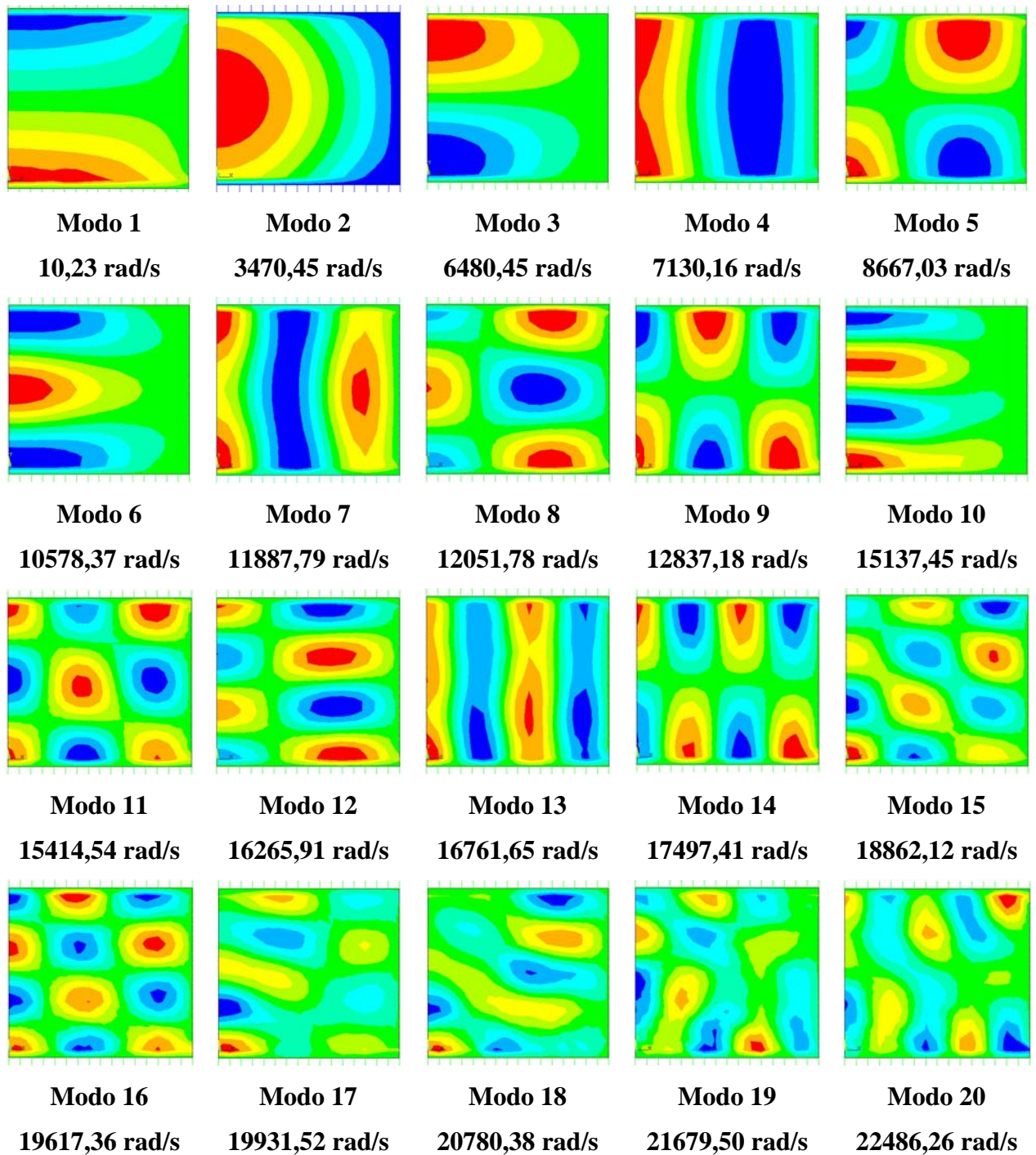
Figura 4.28 – Representação 2D dos modos acoplados da cavidade aberta com pistão duplo obtidos via ANSYS com módulo de elasticidade E=2.1 \times 10^{15} \text{N/m}^2 .
