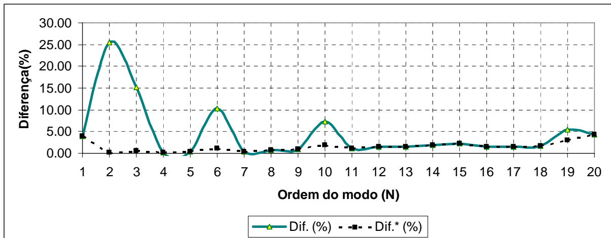
Figura 4.18 – Ordem do modo x Diferença (%) - Caso 1
