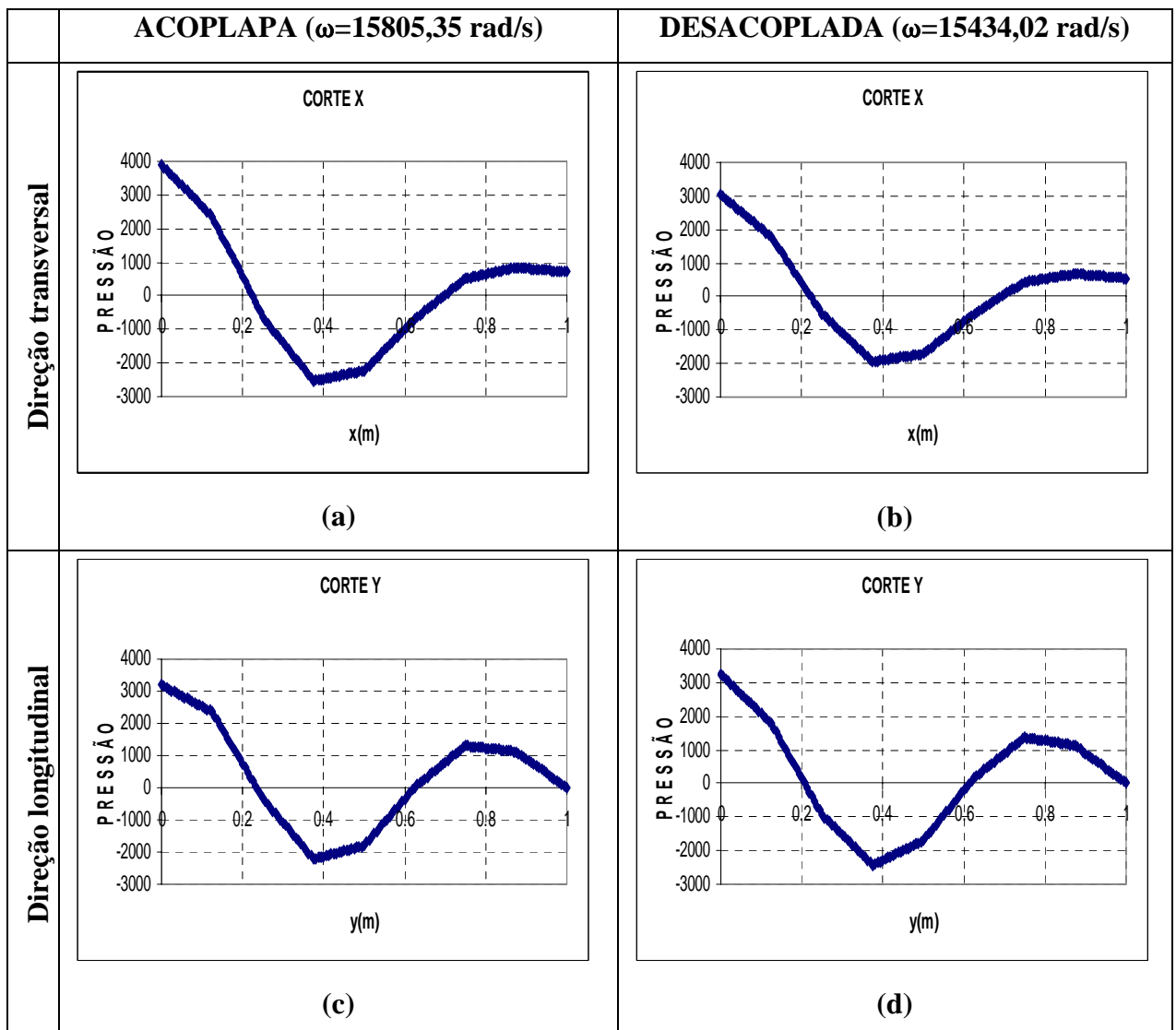
Figura B.26 – Cortes nas direções transversais e longitudinais da cavidade; (a) Corte em x do modo 15, Figura 4.14-(p), (b) Corte em y do modo 15, Figura 4.14-(p), (c) Corte em x do modo 10, Figura 4.12-(j), (d) Corte em y do modo 10, Figura 4.12-(j)
