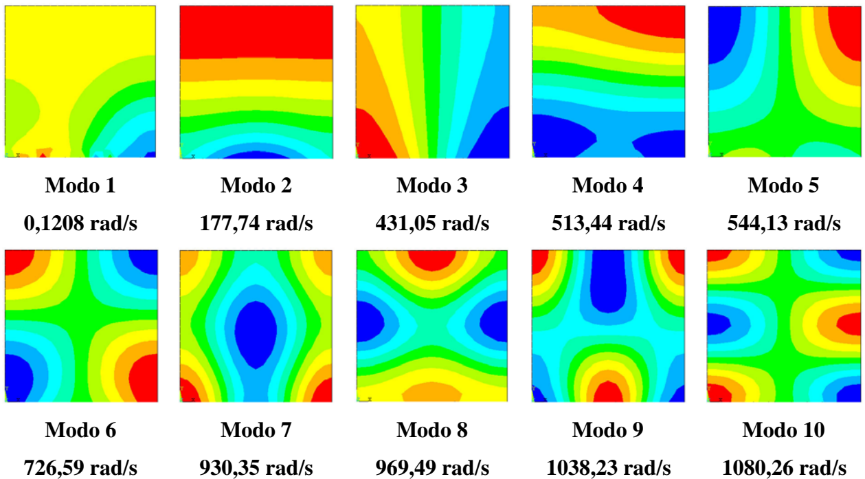
Figura 6.20 – Representação 2D dos modos acoplados da cavidade fechada do caso da viga apoiada obtidos pelo ANSYS
