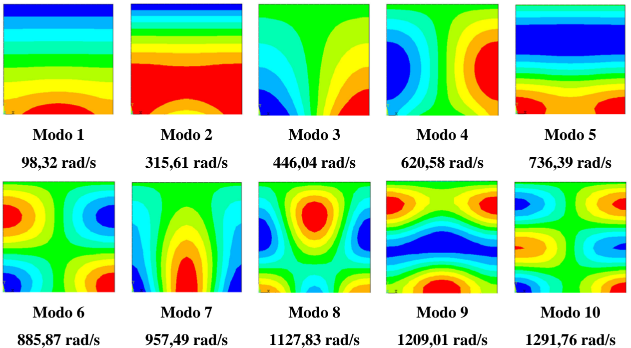
Figura 6.13 – Representação 2D dos modos acoplados da cavidade aberta do caso da viga apoiada obtidos pelo ANSYS
