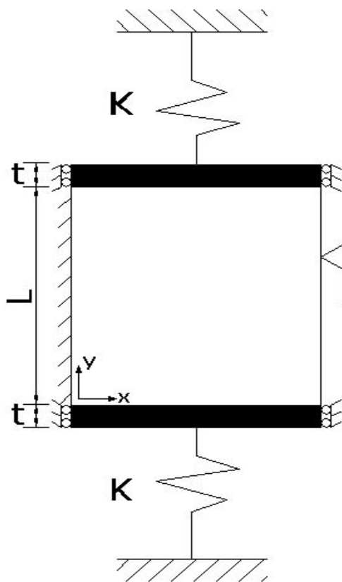
Figura 4.21 – Modelo pistão duplo-cavidade 2D com lateral aberta
