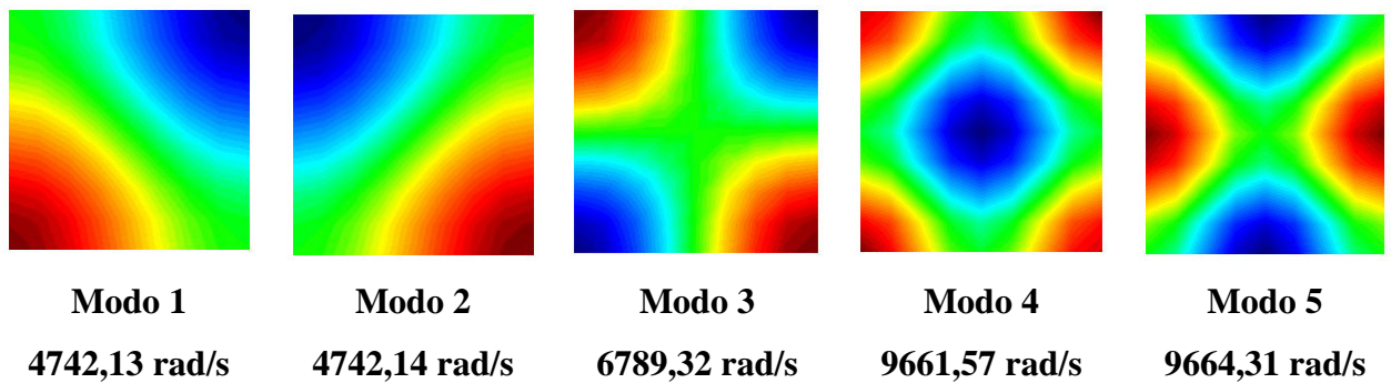
Figura 5.12 – Representação 2D dos modos desacoplados da cavidade fechada obtidos pelo FEDYFE (com instabilidade)
