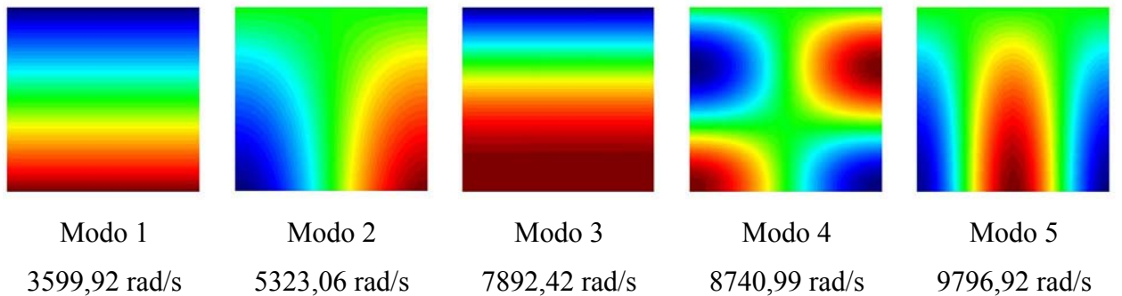
Figura 5.9 – Representação 2D dos cinco primeiros modos acoplados da cavidade aberta obtidos pelo FEDYFE
