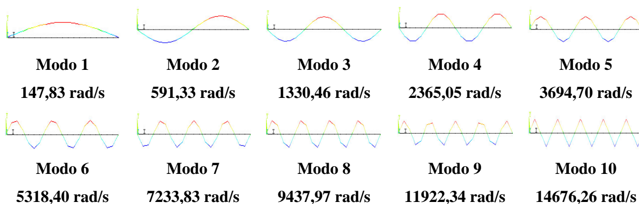
Figura 6.3 – Modos numéricos de vibração da viga biapoiada obtida via ANSYS
