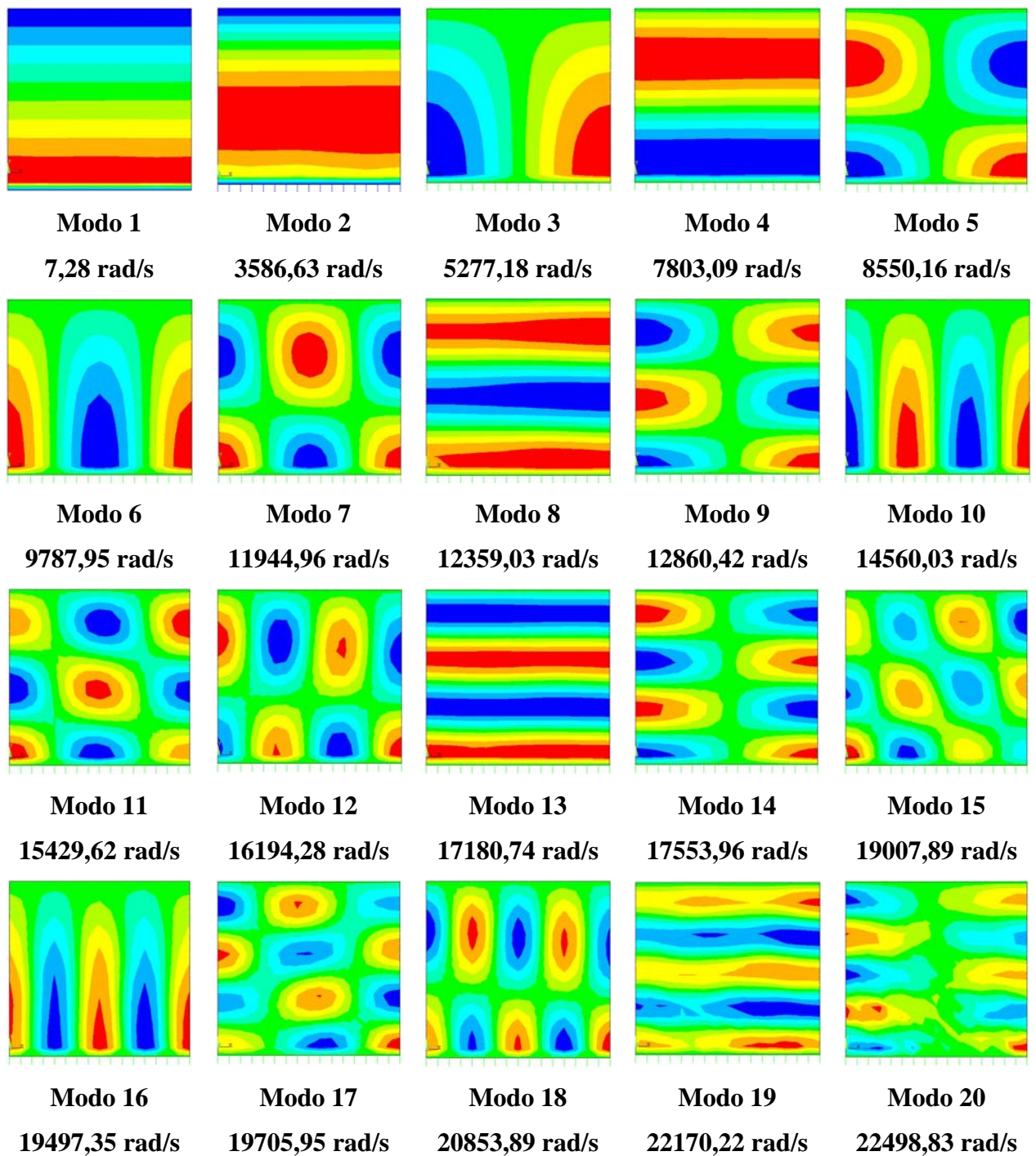
Figura 4.19 – Representação 2D dos modos acoplados da cavidade aberta obtidos via ANSYS com módulo de elasticidade E=2.1 \times 10^{15} \text{N/m}^2 .
