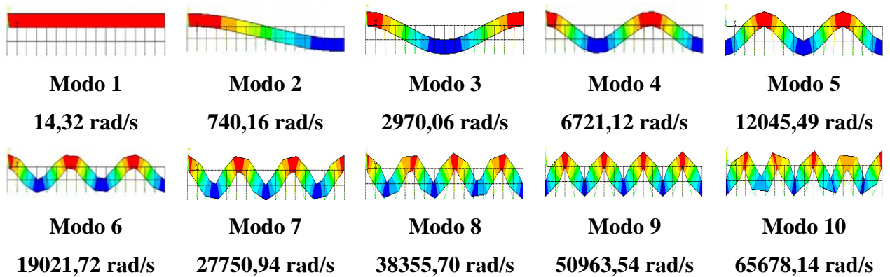
Figura 4.7 – Modos de vibração numéricos da viga sobre base elástica obtidos via ANSYS
