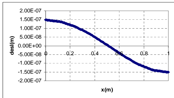
Figura B.7 – Forma modal da estrutura para o problema acoplado da Figura 4.14-(e).
