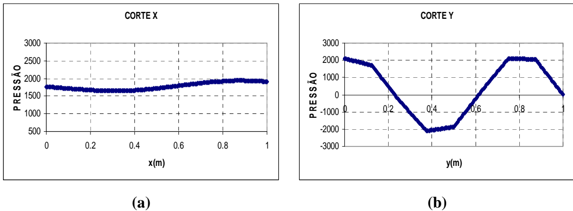
Figura B.18 – Cortes na cavidade do modo 11, Figura 4.14-(l); (a) Corte x - primeiro modo desacoplado para a cavidade fechada-fechada (b) Corte y - quarto modo acoplado para cavidade aberta.
