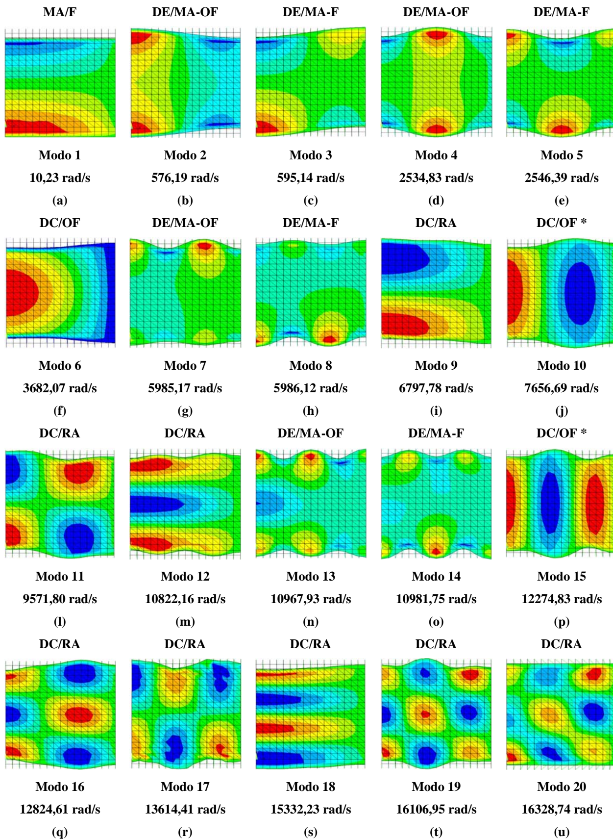
Figura 4.24 – Representação 2D dos modos acoplados da cavidade aberta com pistão duplo obtidos via ANSYS com módulo de elasticidade E=2.1 \times 10^{11} \text{N/m}^2 .
