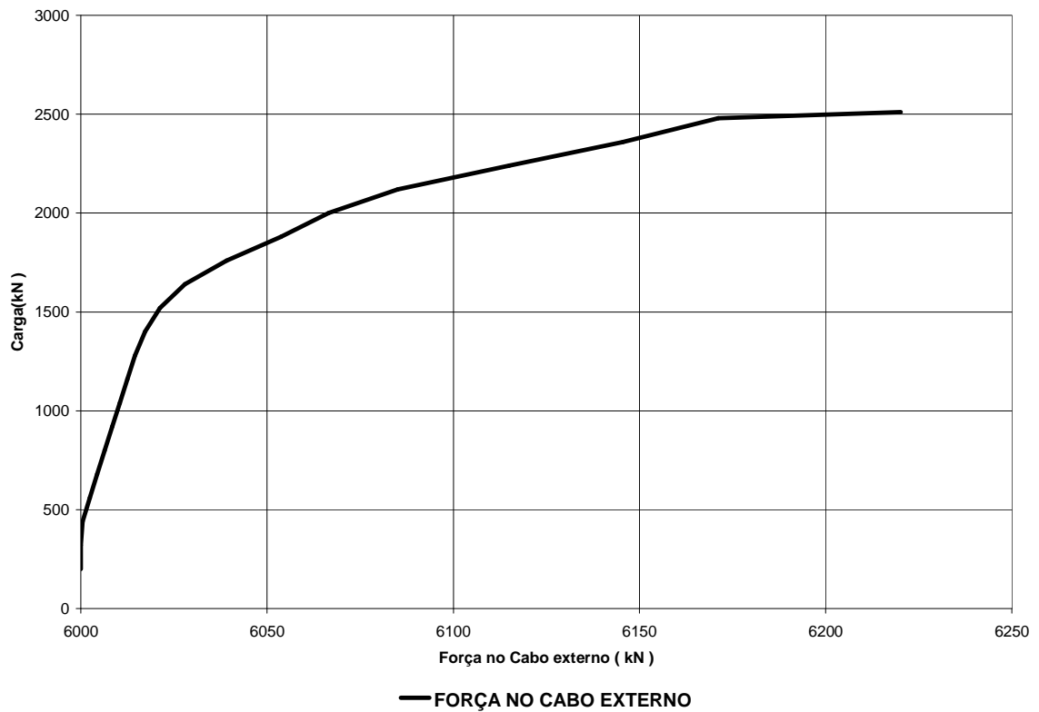
Figura A.9 - Força do cabo externo na seção que foi aplicada a carga – V2
