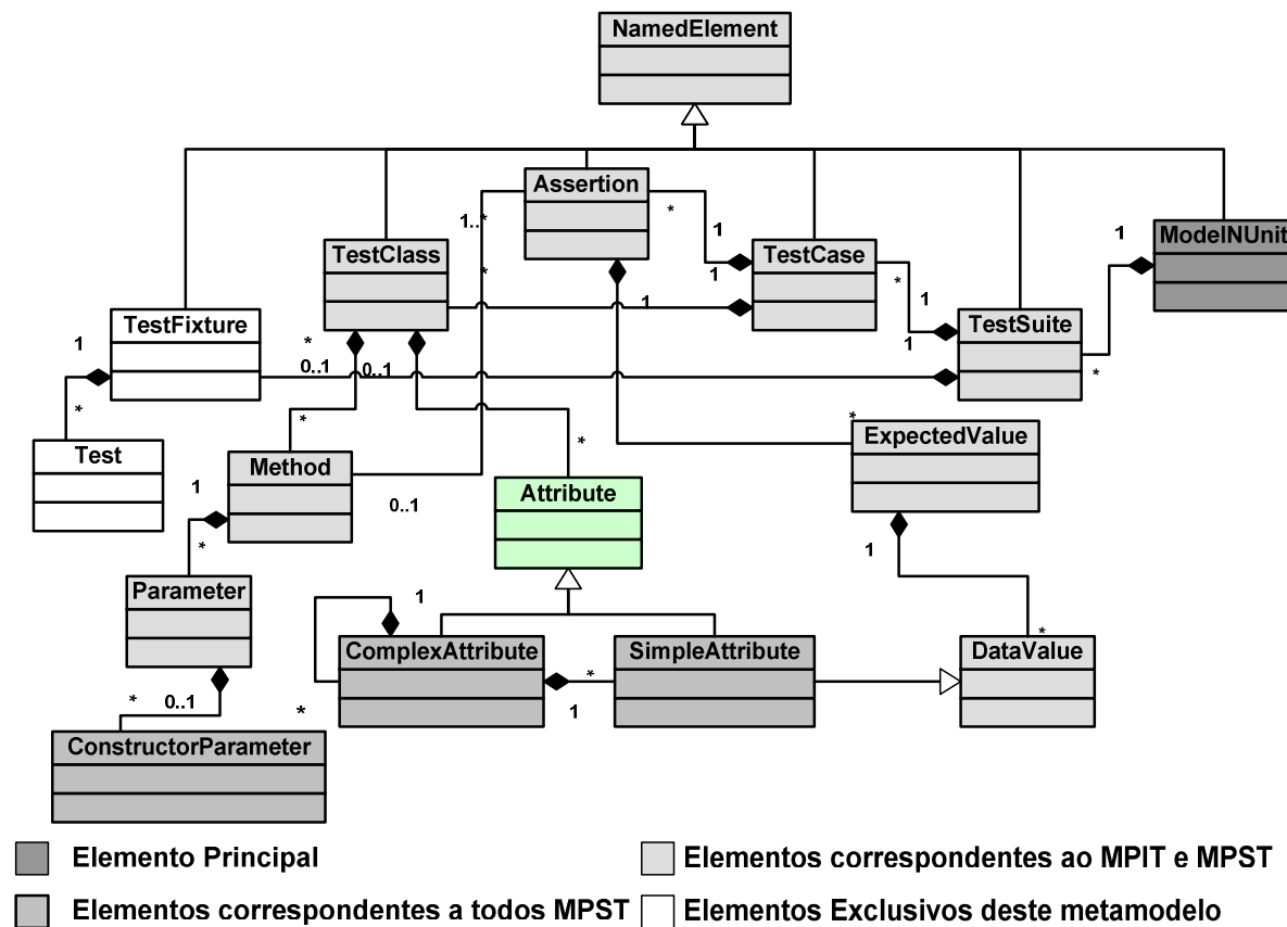
Figura 4.10 - Fragmento do Metamodelo MPST-NUnit
