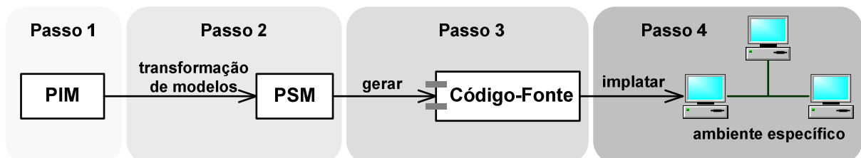
Figura 2.8 - Processo do desenvolvimento MDA (ARLOW & NEUSTADT, 2003)
