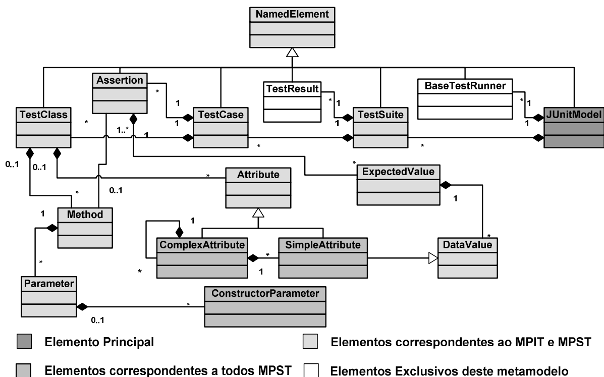
Figura 4.8 - Fragmento do Metamodelo MPST-JUnit
