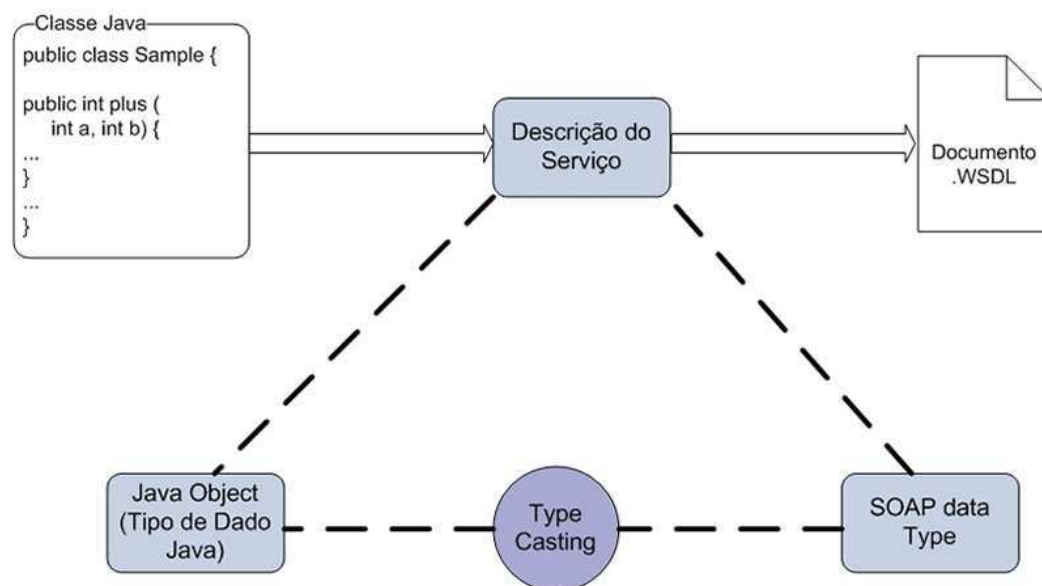
Figura 4.18: Mapeamento classe Java para documento WSDL
