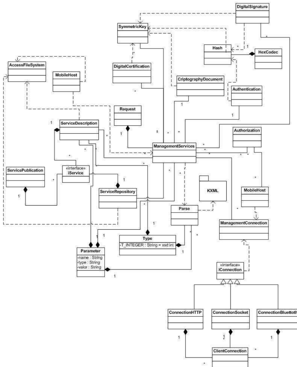
Figura 4.3: Diagrama de Classes do Framework
