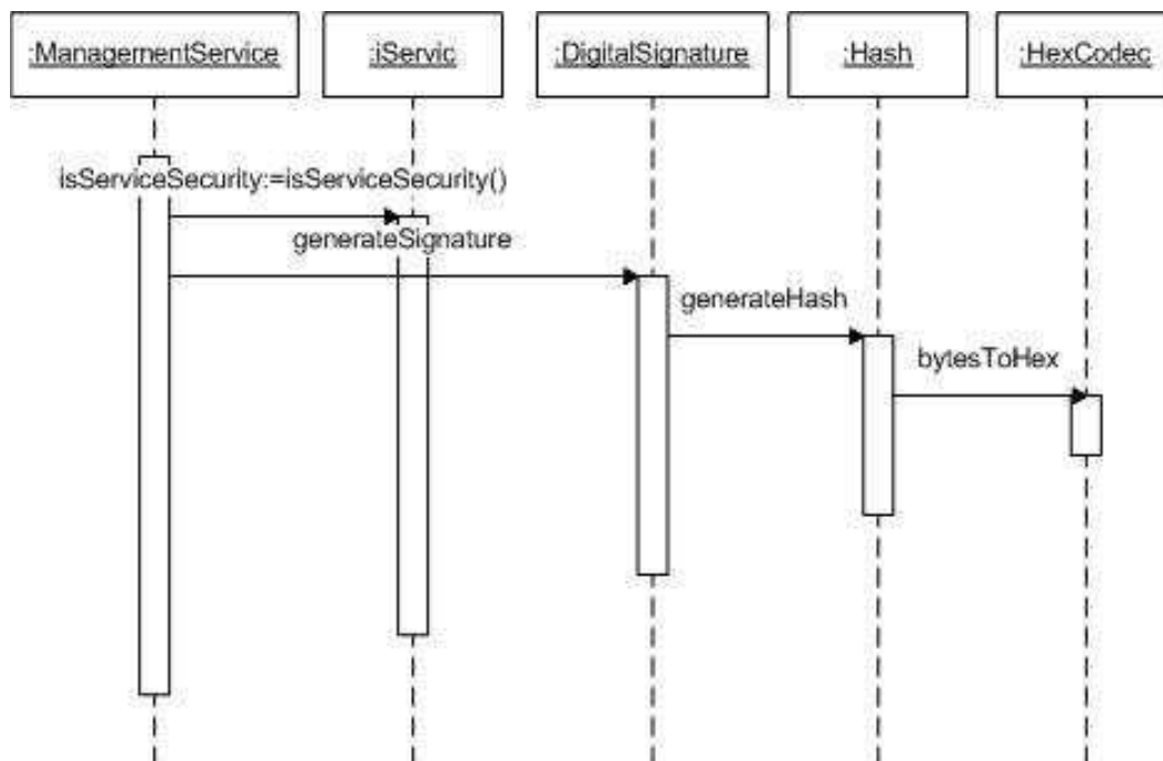
Figura 4.16: Diagrama de Sequência - Geração de Assinatura Digital
