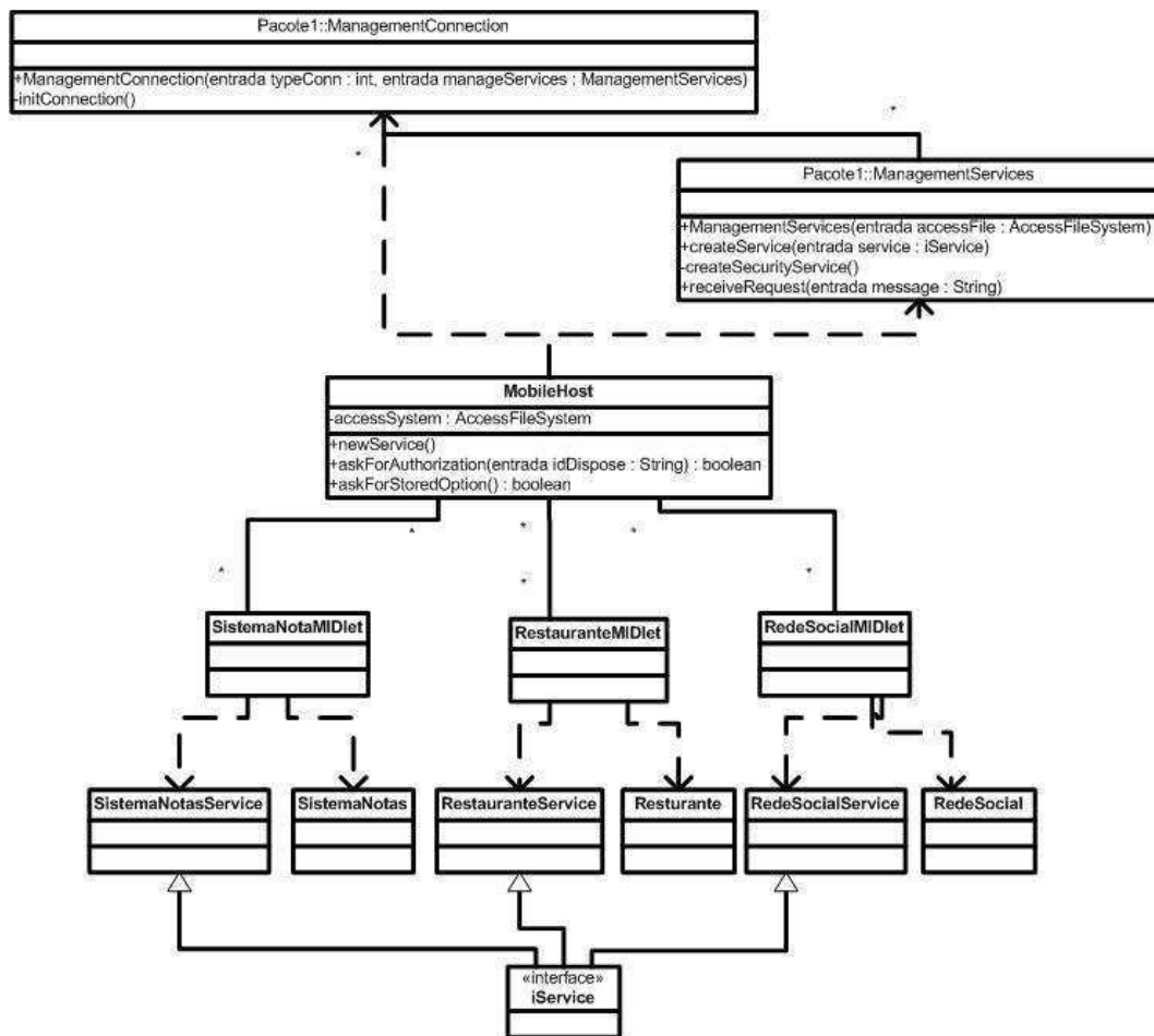
Figura 5.1: Diagrama de Classes dos Estudos de Caso
