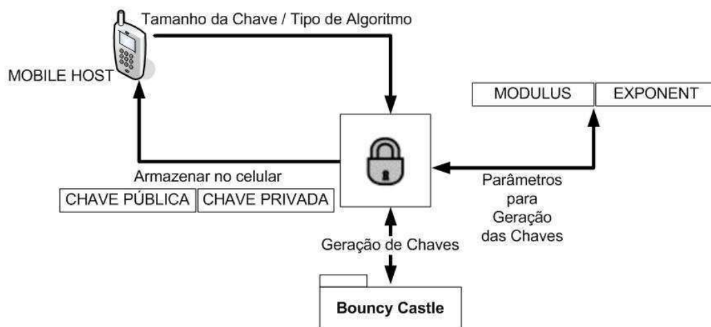
Figura 4.15: Geração de Chaves pelo Framework
