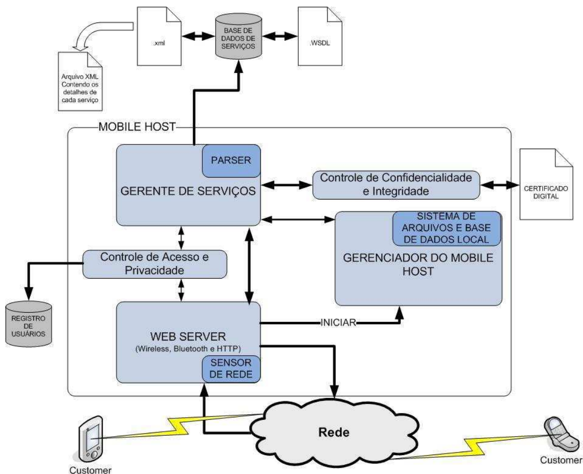
Figura 4.1: Arquitetura Proposta
