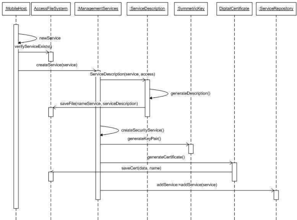
Figura 4.19: Diagrama de Sequência - Processo de Criação de Serviços
