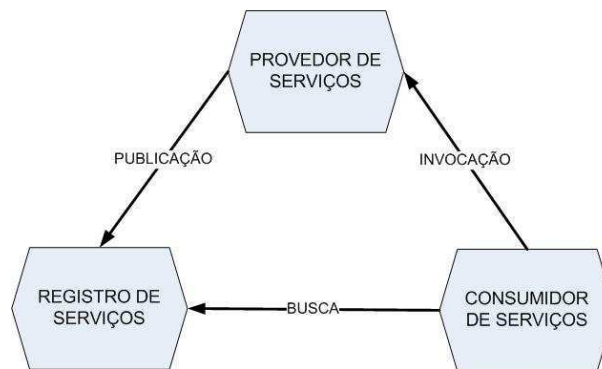
Figura 2.1: Arquitetura Básica de um SOA
