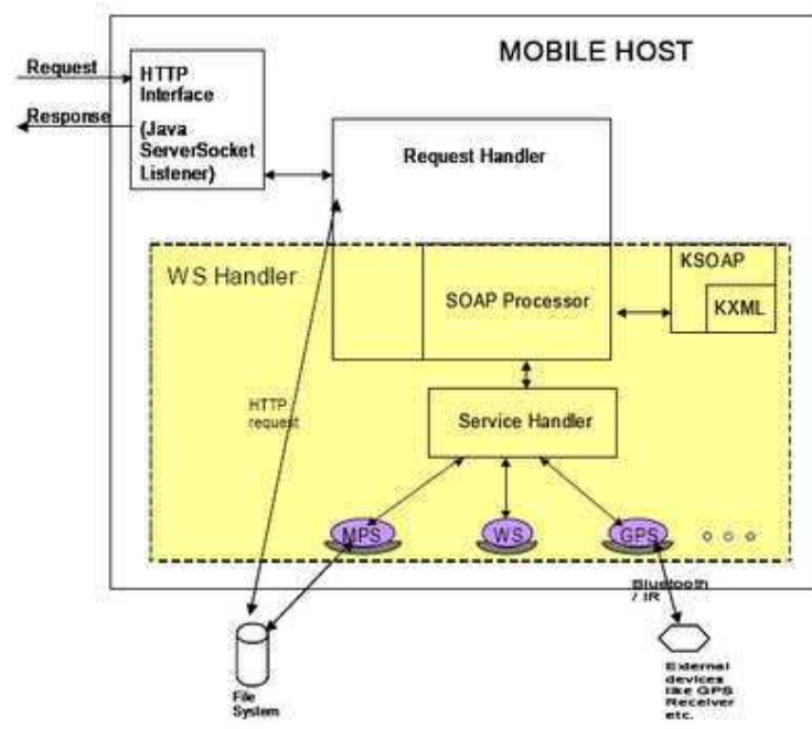
Figura 3.7: Núcleo da Arquitetura Mobile Host, extraído de (Srirama 2006b)
