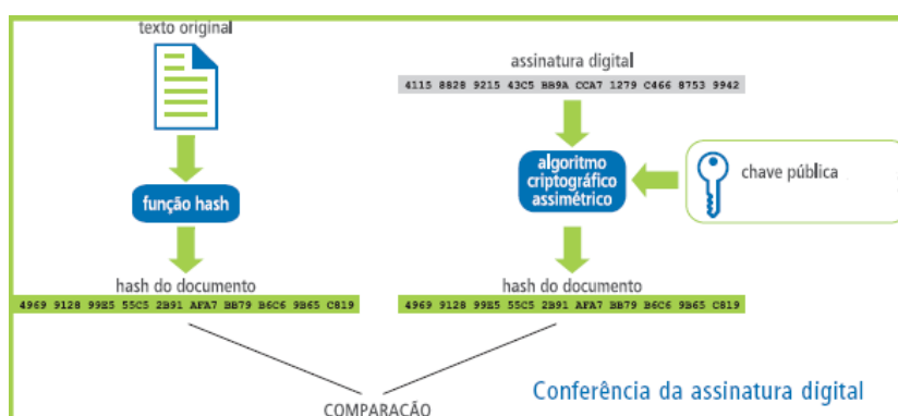
Figura 2.9: Processo de validação das mensagens assinadas digitalmente
