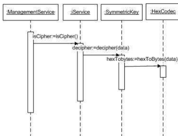
Figura 4.17: Diagrama de Sequência - Decifrar Mensagem Recebida
