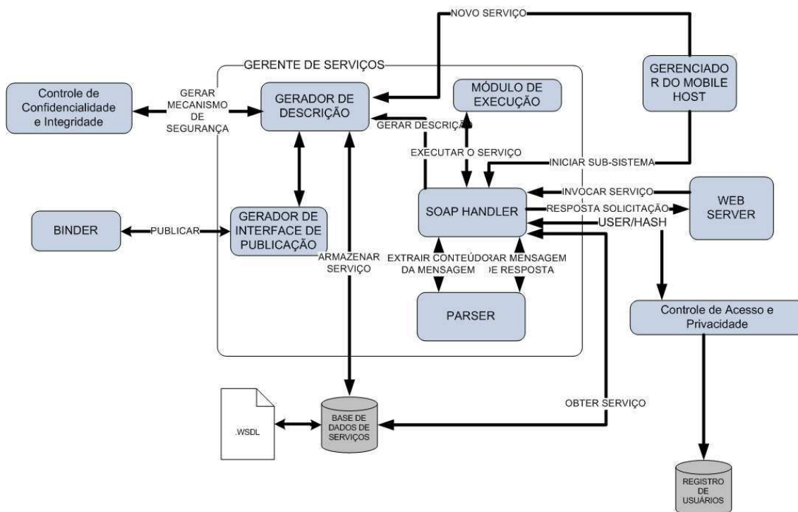
Figura 4.8: Gerente de Serviços
