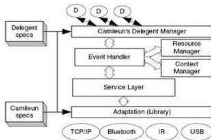
Figura 3.4: Pilha do middleware PICO, extraído de (Kalasapur 2005)
