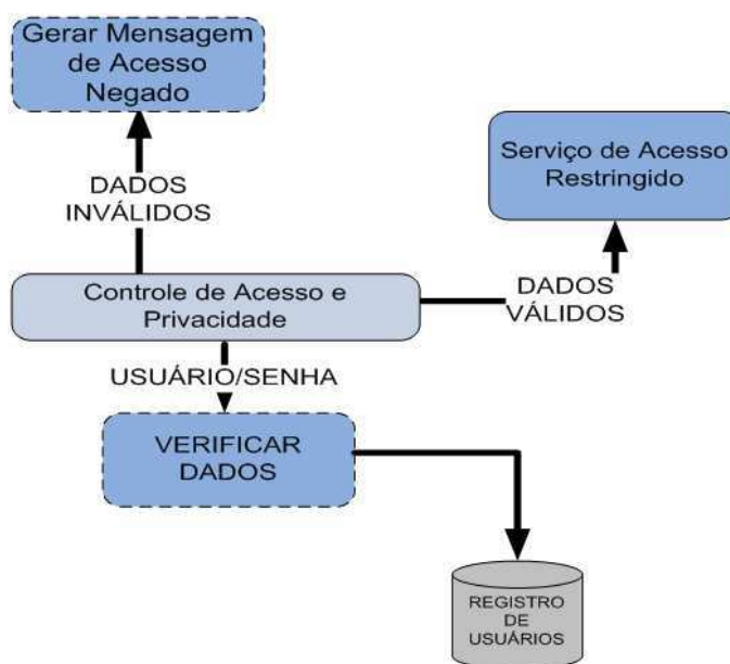
Figura 4.11: Processo de Validação de Mensagem Recebida
