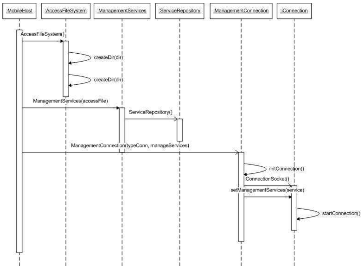
Figura 4.5: Diagrama de Sequência - Inicialização do Mobile Host
