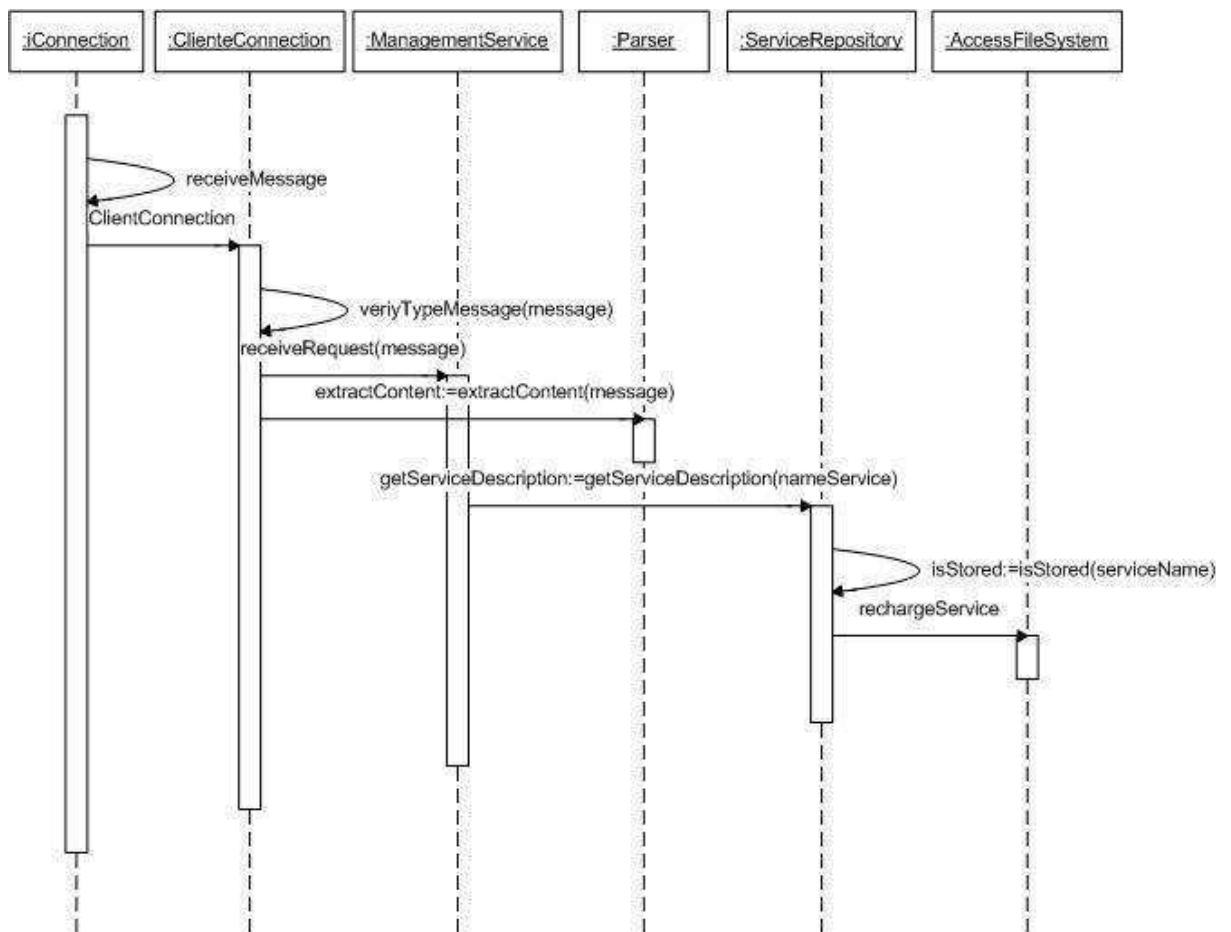
Figura 4.7: Diagrama de Sequência - Processamento de Requisição Recebida
