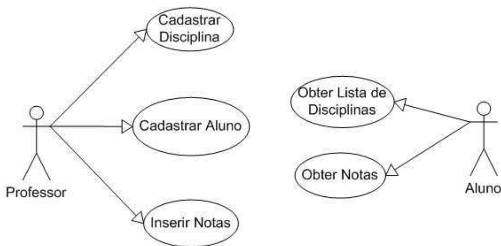
Figura 5.2: Diagrama de Caso de Usos - Sistema de Notas
