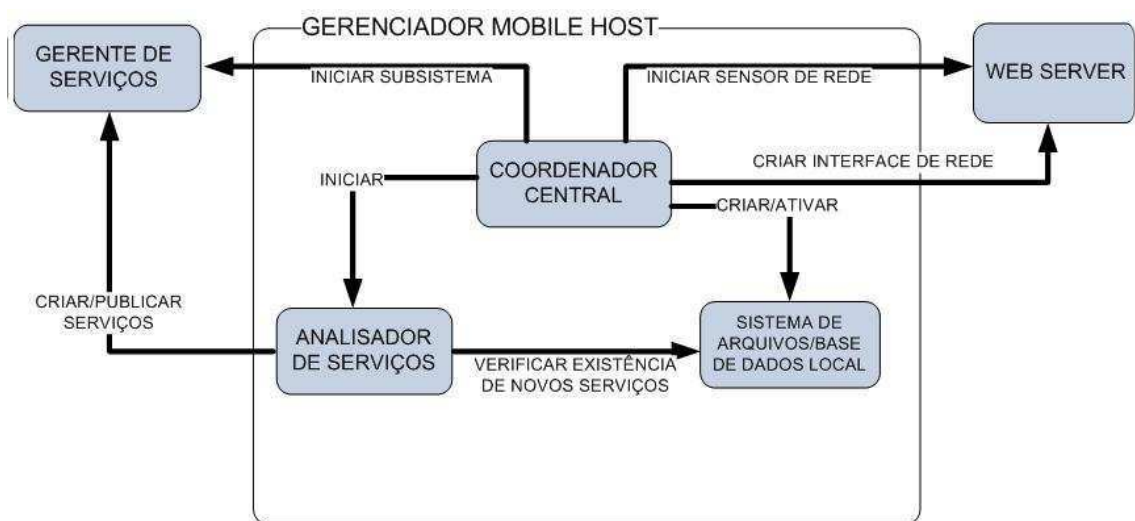
Figura 4.4: Gerenciador do Mobile Host
