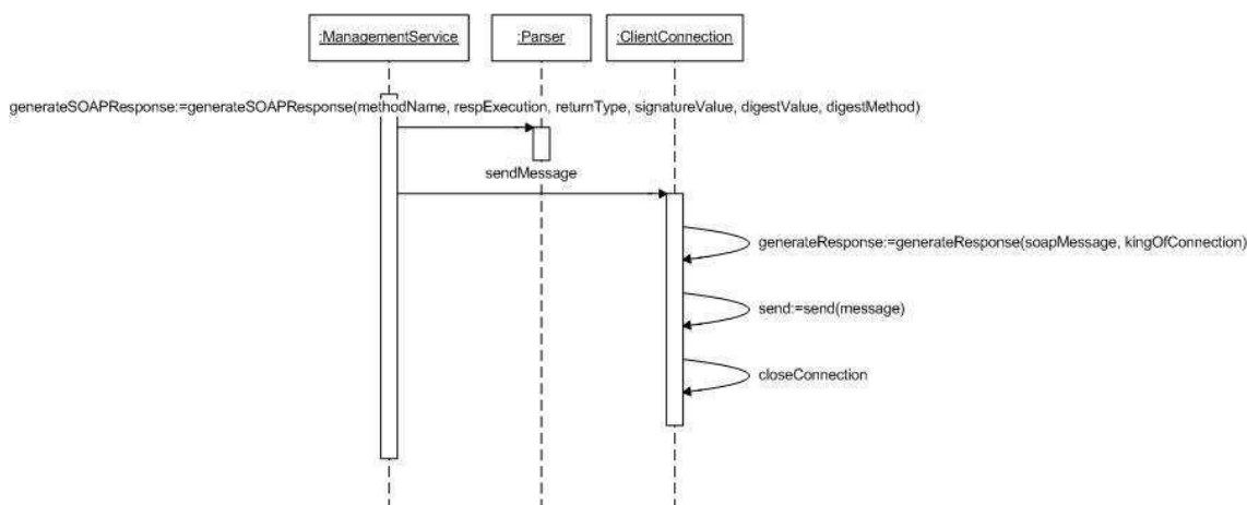
Figura 4.9: Diagrama de Sequência - Geração de Mensagem de Resposta
