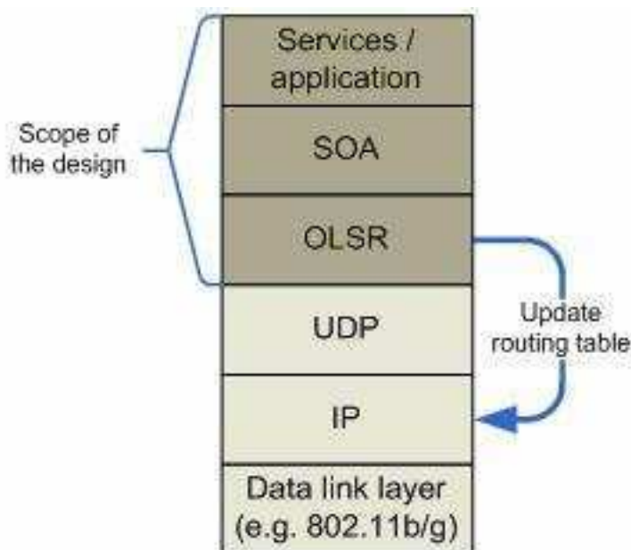
Figura 3.2: Pilha de protocolos da Implementação do protótipo, extraído de (Halonen 2006)
