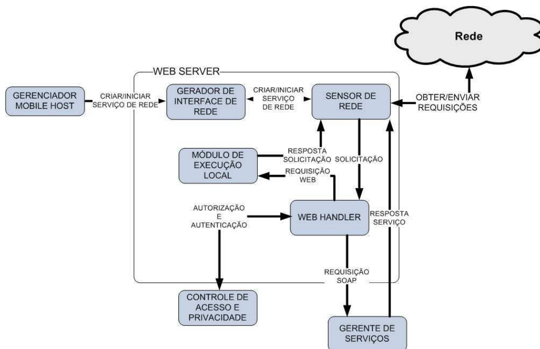
Figura 4.6: Componentes do Web Server Utilizado pela Arquitetura
