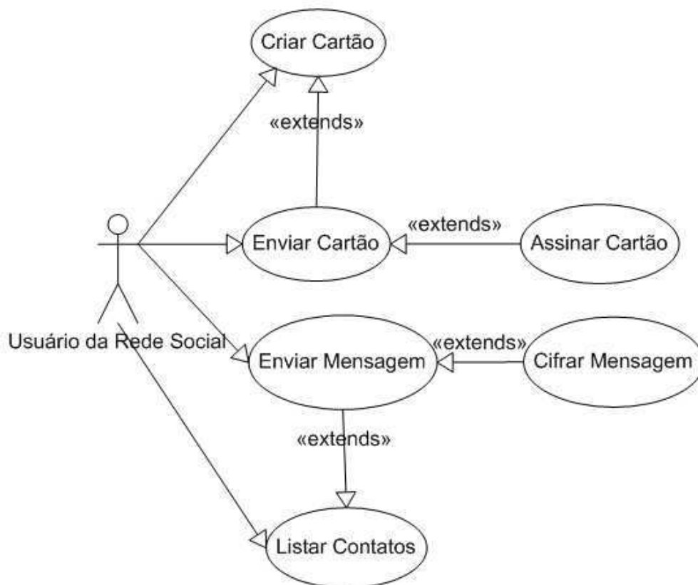
Figura 5.12: Diagrama de Caso de Usos - Rede Social
