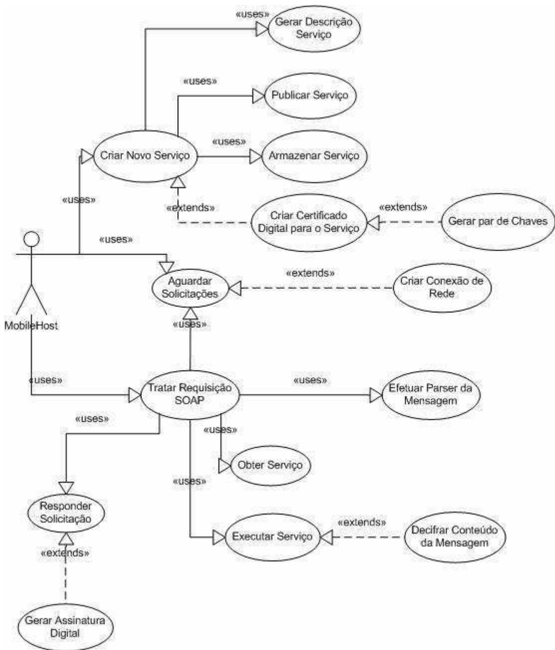
Figura 4.2: Diagrama de Casos de Uso
