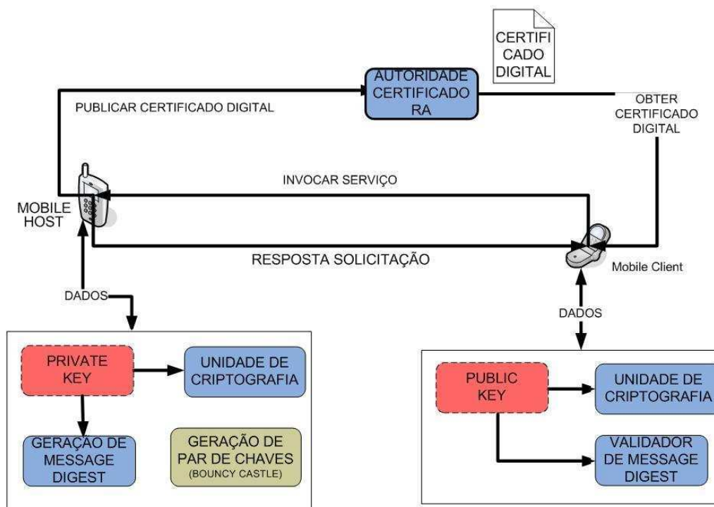
Figura 4.14: Serviço de Segurança: Confidencialidade e Integridade
