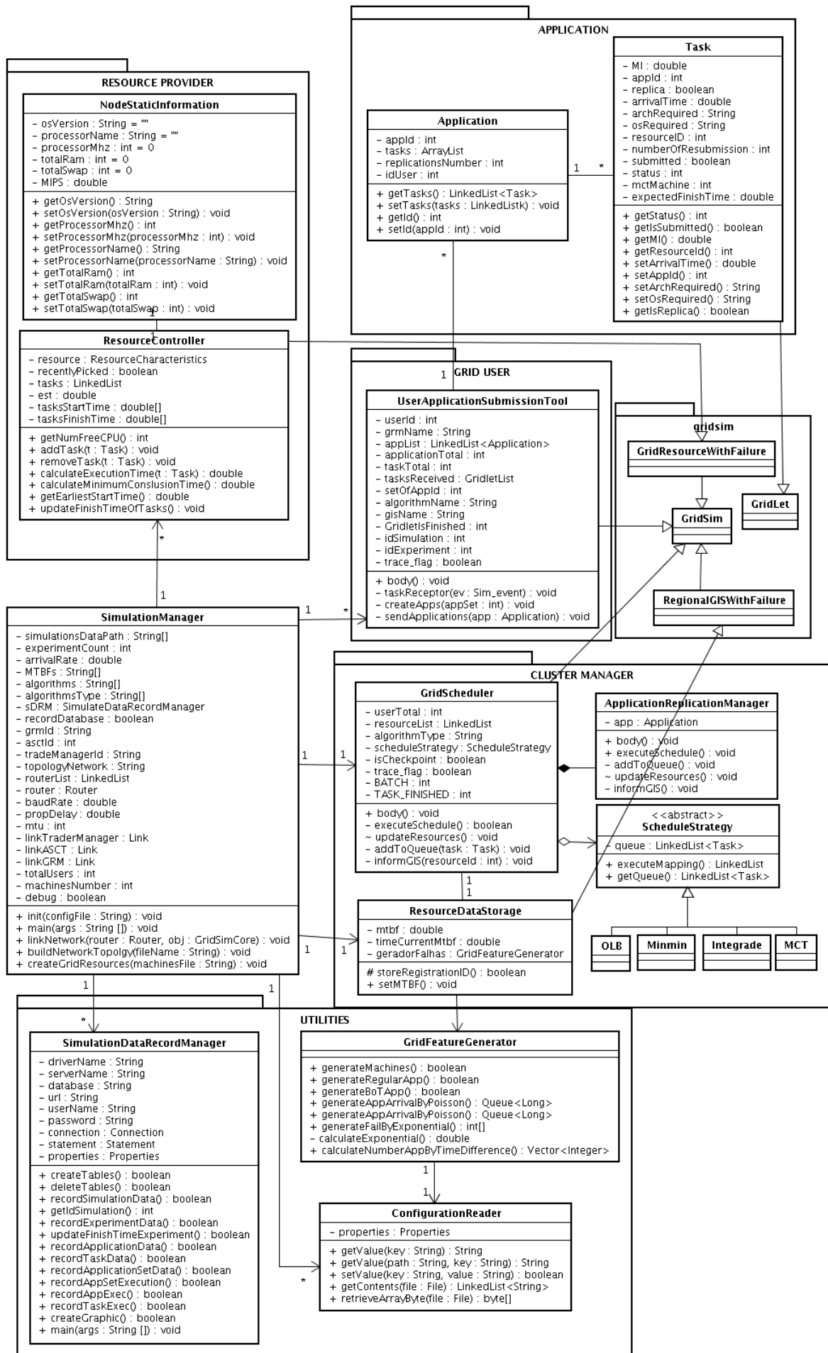
Figura 3.2: Diagrama de classe do OGST
