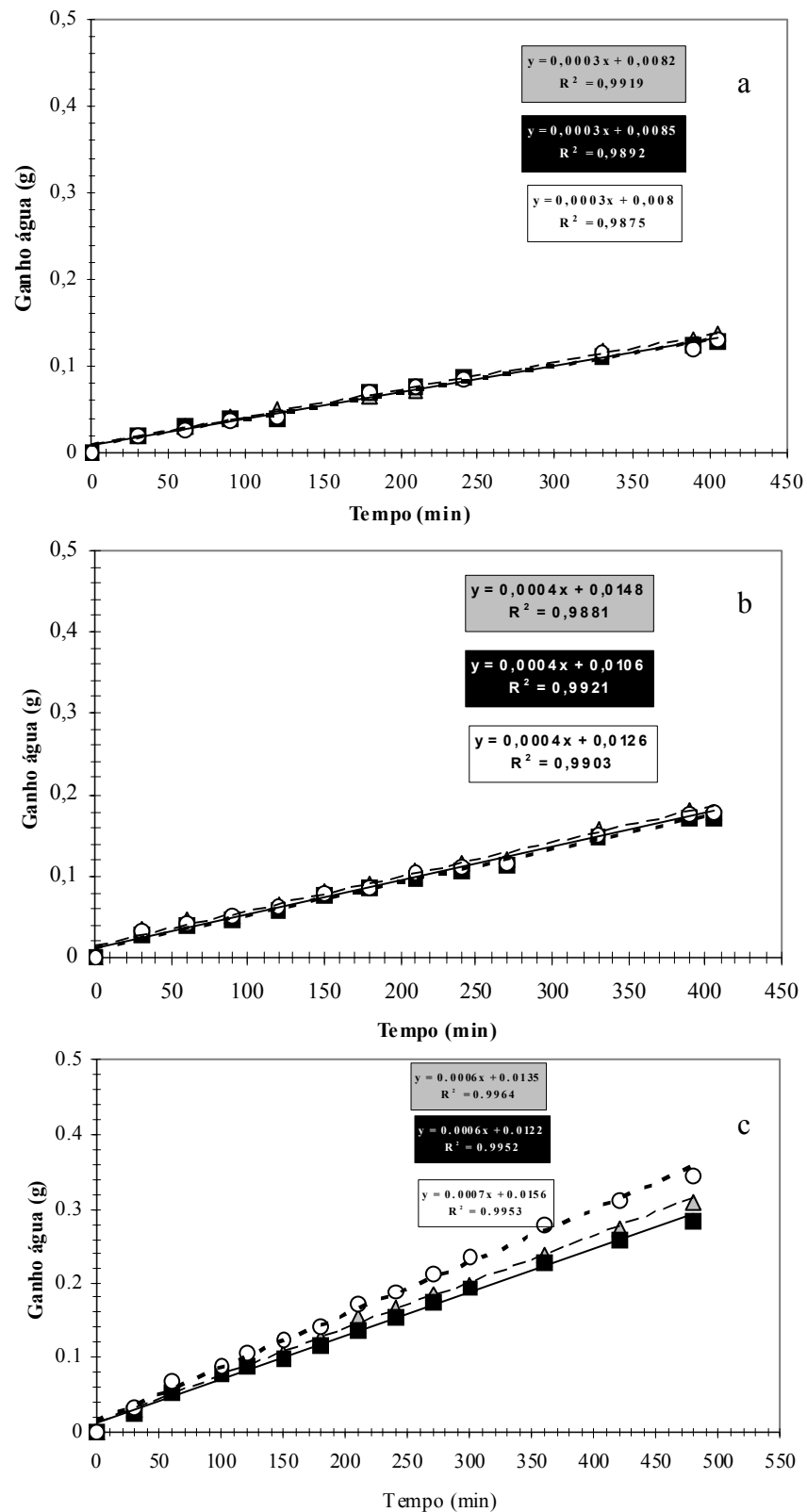
Figura 5.1 – Triplicatas da evolução do peso das células de medida de PVA em função do tempo. Primeira ( \blacktriangle ), segunda ( \blacksquare ) e terceira medida (o) para filmes plastificados com 0,02(a), 0,05(b) e 0,10(c)g PEG 400/g queratina utilizadas, para o cálculo da permeabilidade ao vapor d'água.
