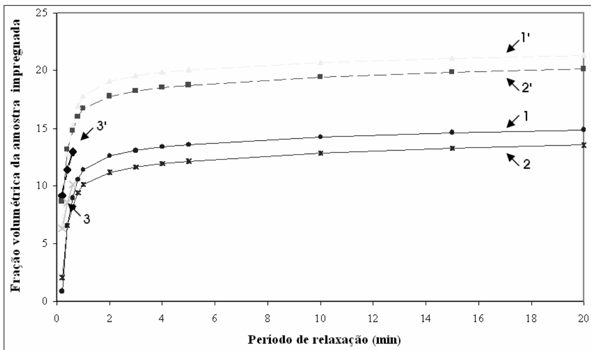
Figura 3.18 - Comparação entre os valores da fração volumétrica efetiva da amostra impregnada (curvas 1, 2 e 3) calculada pela Equação 2.5 \left( X = \frac{w - w_0}{\rho V_0} \right) , com os valores da fração real da amostra preenchida pela solução pela ação do HDM (curvas 1', 2' e 3').
