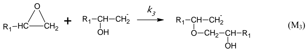
Figura 2. 4. Reações envolvidas na cura de uma resina epoxídica.
