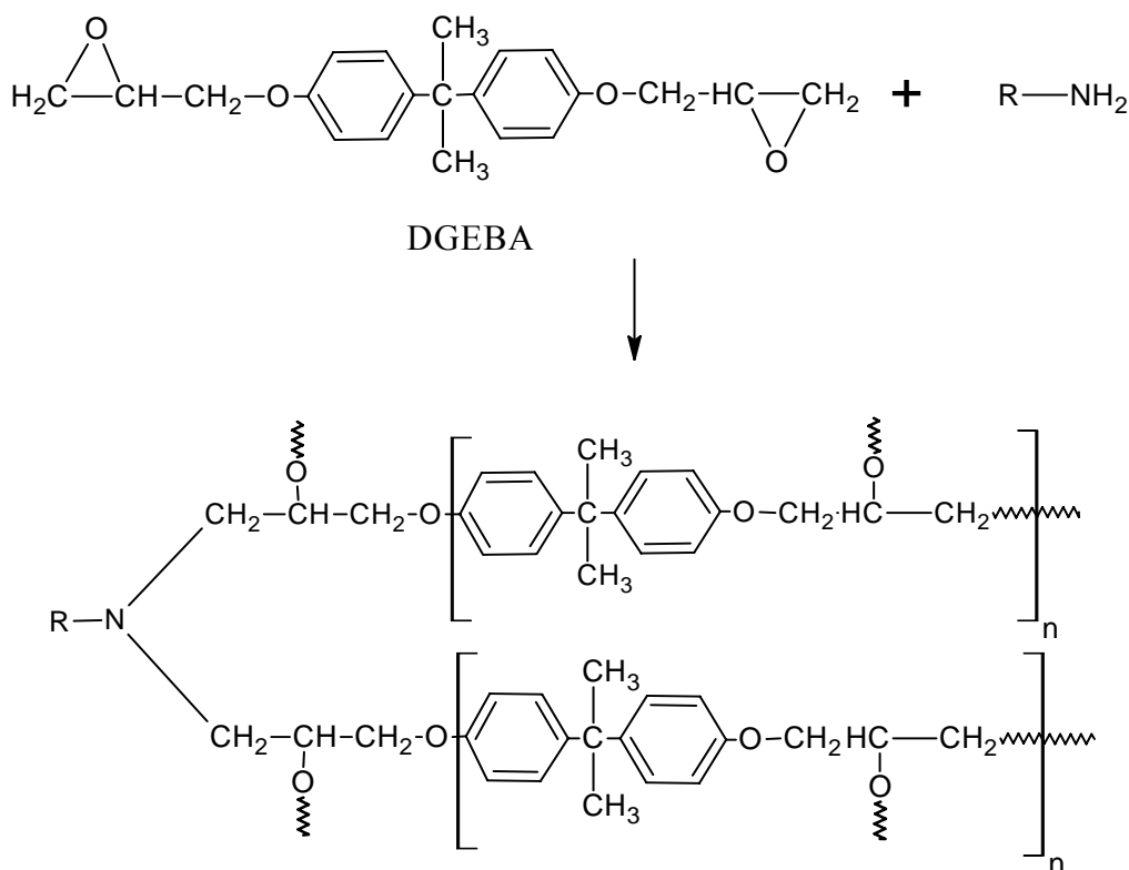
Figura 2. 3. Esquema reacional da polimerização da resina DGEBA.
