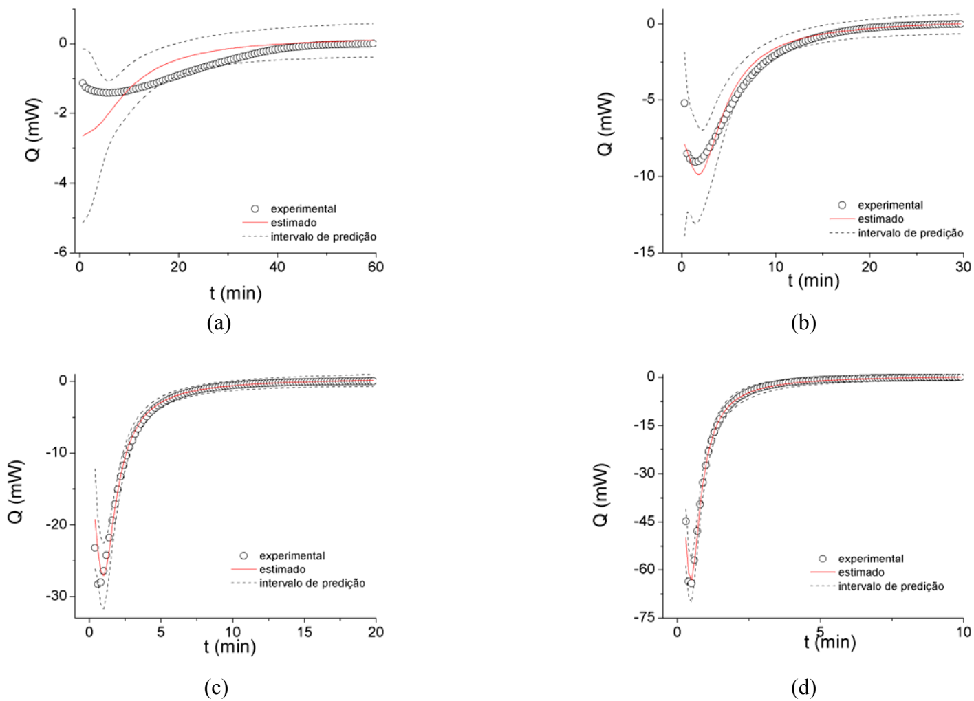
Figura 5. 39. Resultados teóricos e experimentais da taxa de calor para o caso isotérmico: (a) 333 K, (b) 353 K, (c) 373 K e (d) 393 K.
