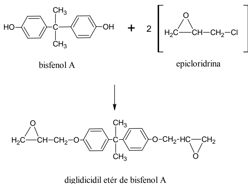
Figura 2. 2. Esquema de produção do DGEBA.
