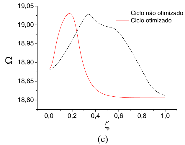
Figura 5. 26. (a) Grau de cura, (b) temperatura e (c) função objetivo do processo de enrolamento filamental com ciclo de cura otimizado.
