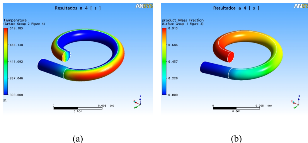
Figura 5. 24. Perfis de (a) temperatura e (b) grau de cura no compósito para o processo de enrolamento filamental.
