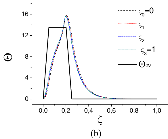
Figura 5. 26. (a) Grau de cura, (b) temperatura e (c) função objetivo do processo de enrolamento filamental com ciclo de cura otimizado.
