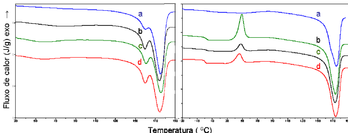
Figura 5.2: Curvas de DSC (1° e 2° aquecimento) para os filmes de P(3HB) extraídos pelo método mecânico purificado em função do tempo de biodegradação em solo compostado: a) 0 dias; b) 7 dias; c) 14 dias; d) 21 dias.
