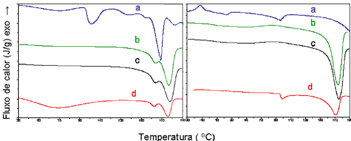
Figura 5.3: Curvas de DSC (1° e 2° aquecimento) para os filmes de P(3HB) extraídos pelo método mecânico não purificado em função do tempo de biodegradação em solo compostado: a) 0 dias; b) 7 dias; c) 14 dias; d) 21 dias.
