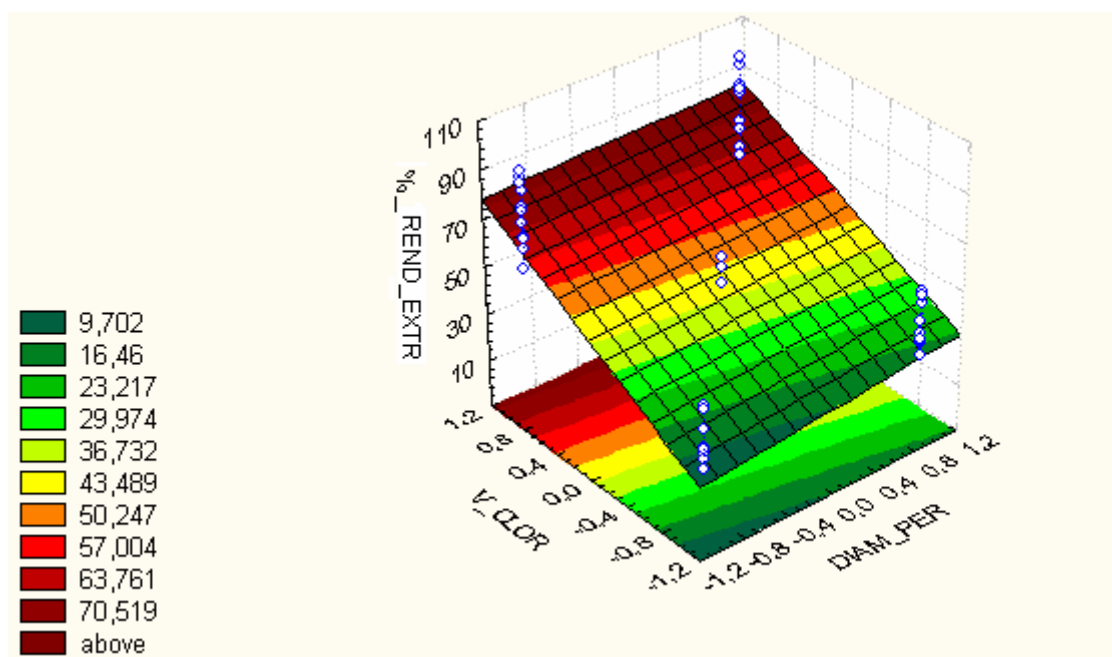
Figura 3.6: Gráfico de superfície demonstrando a interação entre o volume de clorofórmio e o diâmetro das pérolas sobre o rendimento de extração de P(3HB).
