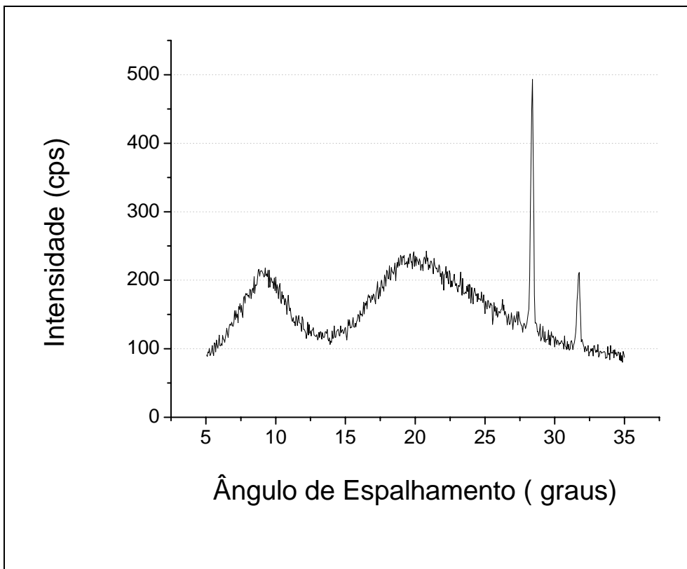
Figura 4. 3 – Perfil característico das amostras de plasma (PL).
