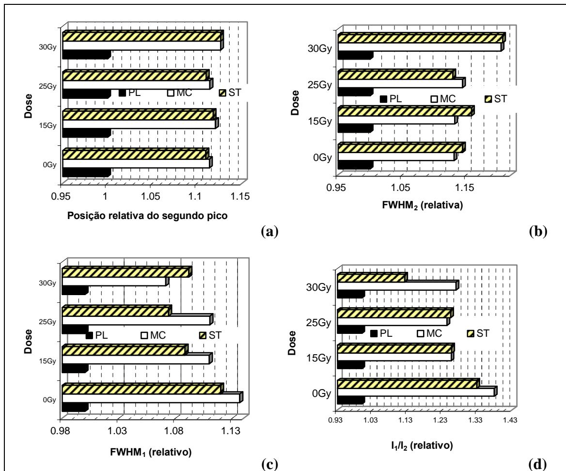
Figura 4. 6 – Comparação dos valores médios encontrados para parâmetros de caracterização: (a) \theta_2 , (b) FWHM 2 , (c) FWHM 1 e (d) I 1 /I 2 .
