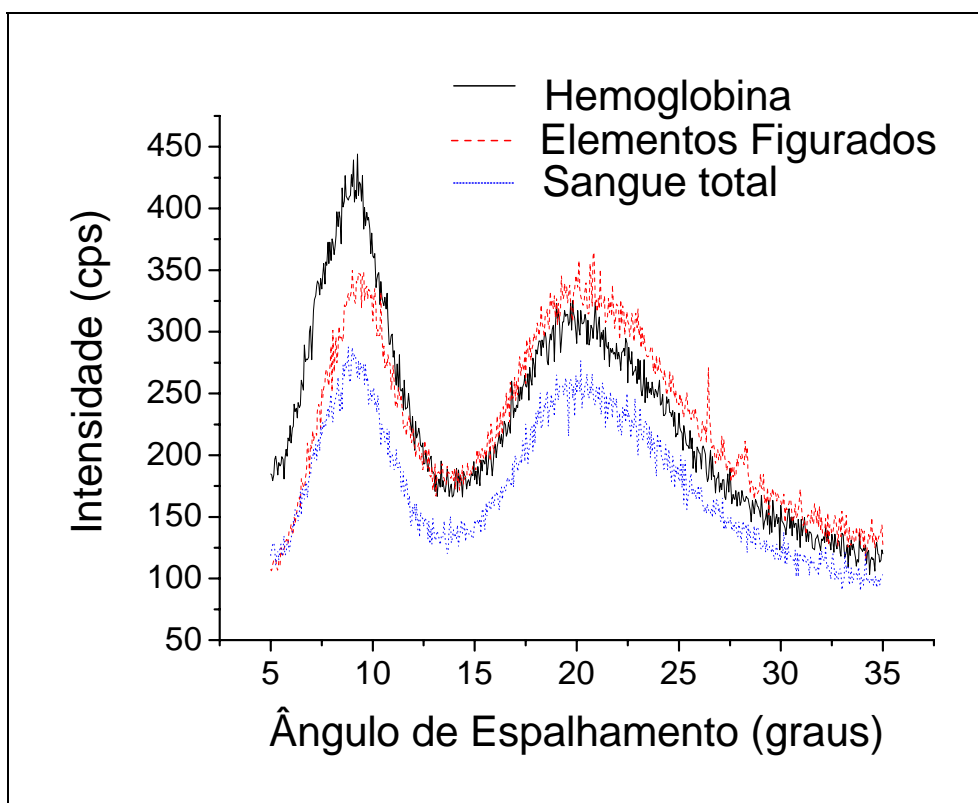
Figura 4. 4 - Comparação entre os perfis de espalhamento de ST, MC e HB.
