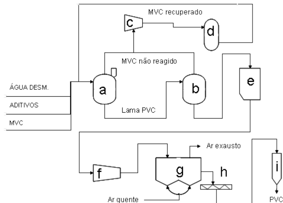
Figura 8. Fluxograma do processo de produção do PVC via suspensão.
