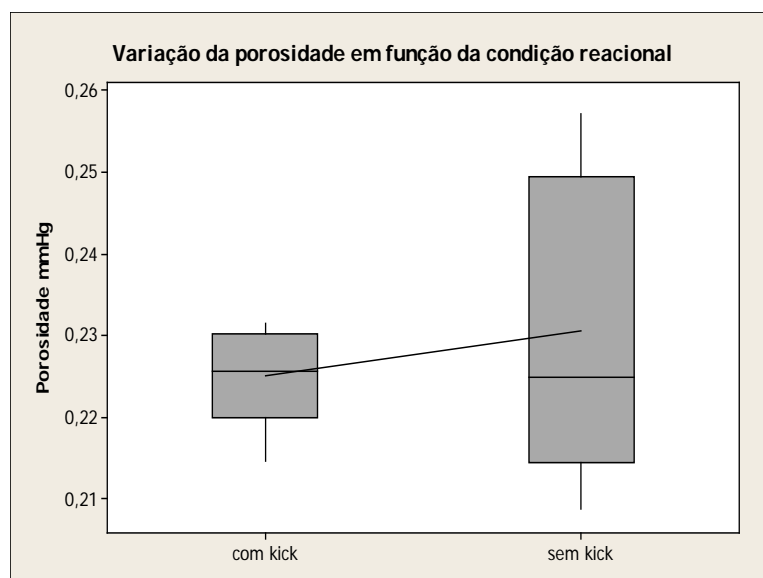
Figura 14 – Resultados de porosidade em função da condição reacional.
