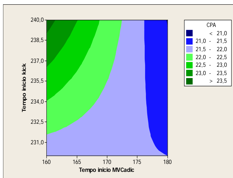
Figura 32. Superfície de contorno para a porosidade versus o tempo do início de adição de MVC.
