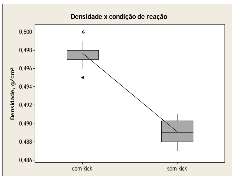
Figura 15 – Resultados de densidade aparente em função da condição reacional.
