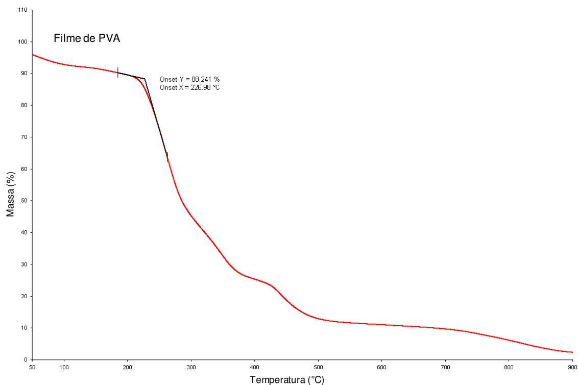
Figura 4.17. Curva de análise termogravimétrica da membrana de PVA 99% hidrolisado.
