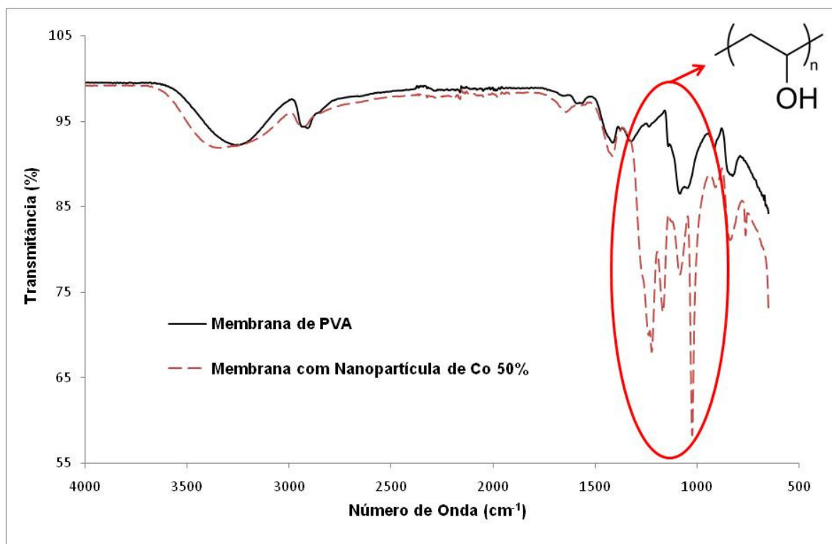
Figura A.4.3. Espectros de infravermelho (FTIR) das membranas de PVA 99% hidrolisado e PVA + Nanopartícula de Co 50%.
