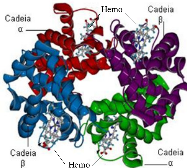
Figura 2.15. Representação da estrutura da hemoglobina destacando as cadeias \alpha e \beta da parte globina e os quatro grupos hemo. Fonte: www.commonswiki.org .
