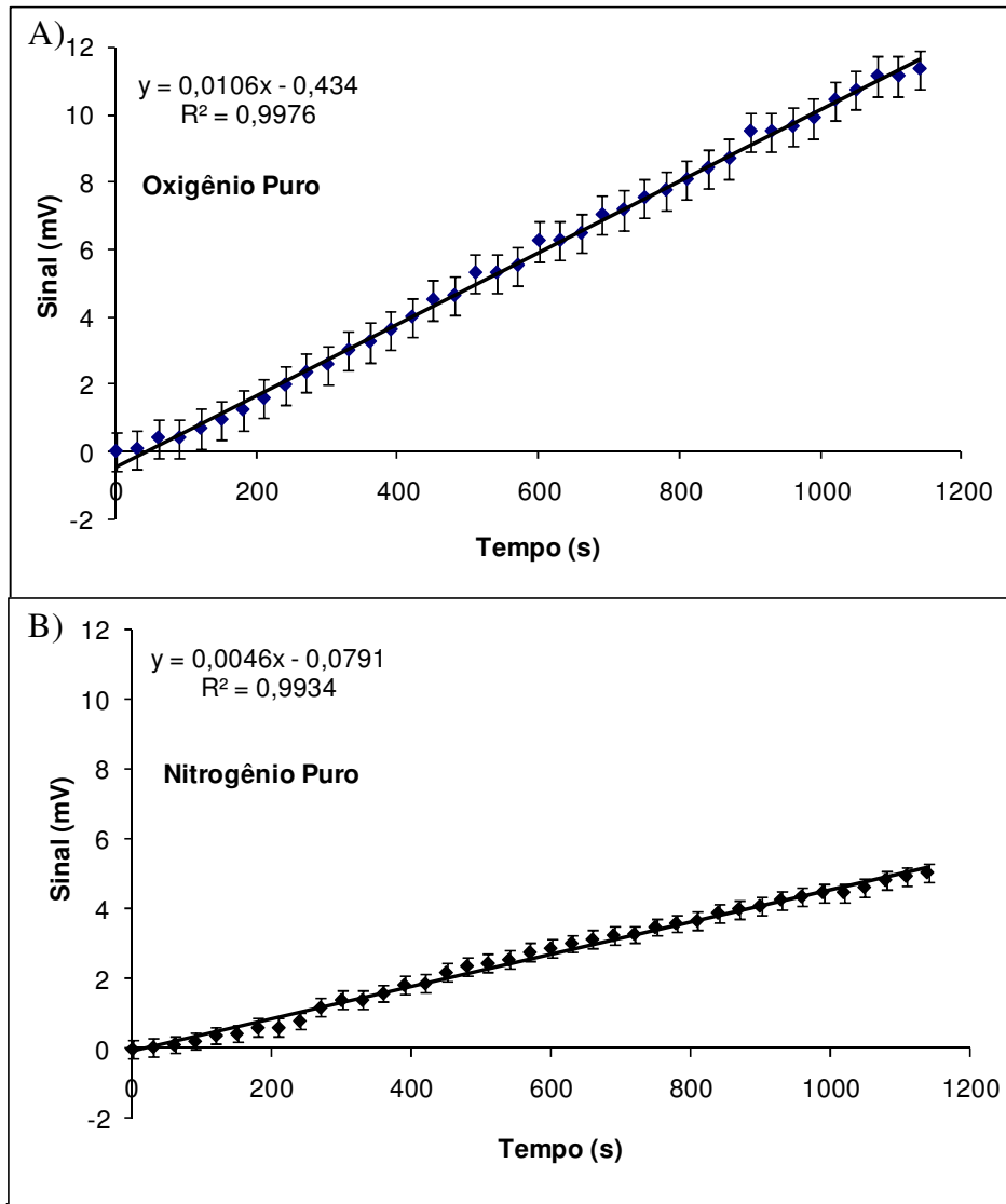
Figura 4.1. Variação do sinal (mV) do transdutor de pressão com o tempo, utilizado para determinar a permeabilidade nas membranas de PDMS. (A) O 2 ; (B) N 2 .
