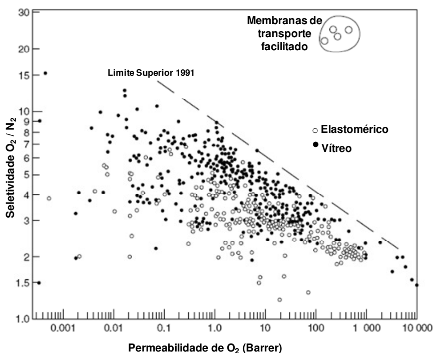
Figura 2.5. Diagrama de Robeson para a separação O_2/N_2 e as propriedades de algumas membranas de transporte facilitado (BAKER, 2002).
