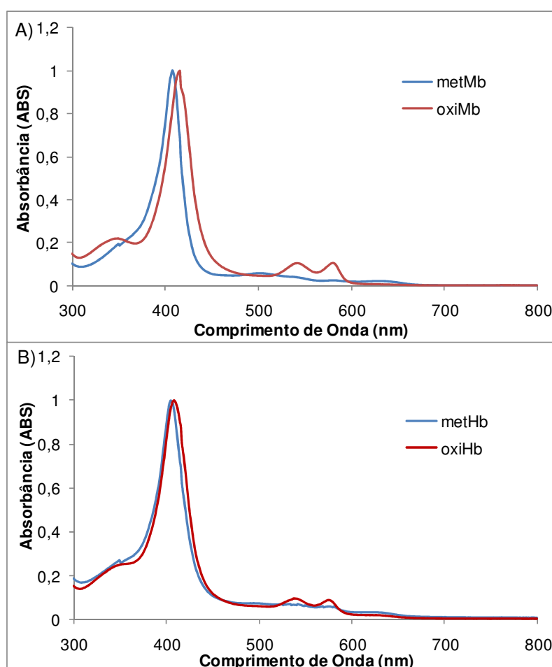
Figura 4.3. Espectros de absorção UV/Vis das soluções tampão (pH = 7,0 e T = 25°C) dos biotransportadores. A) Espectros de metMb e oxiMb; B) Espectros de metHb e oxiHb.
