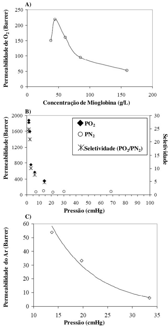
Figura 2.20. Permeabilidade e seletividade em membranas com biotransportadores. A) Efeito da concentração do transportador na permeabilidade da membrana. B) Permeabilidade de uma membrana líquida contendo mioglobina como uma função da diferença de pressão através da membrana. C) Permeabilidade de oxigênio em PVA contendo mioglobina (FERRAZ, 2007).
