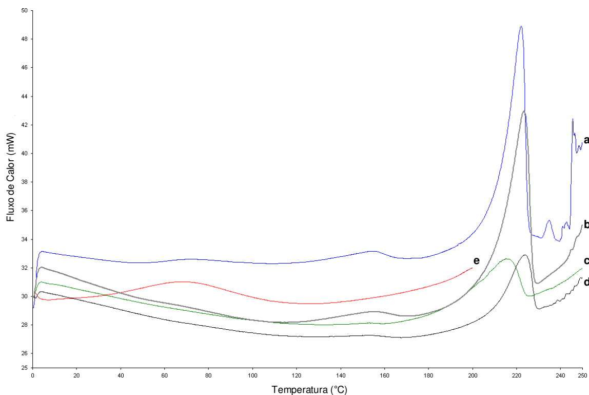
Figura 4.21. Curvas de DSC. a) PVA; b) PVA/metMb reduzida com ditionito de sódio; c) PVA/oxiMb; d) PVA/metMb; e) Mb em pó.
