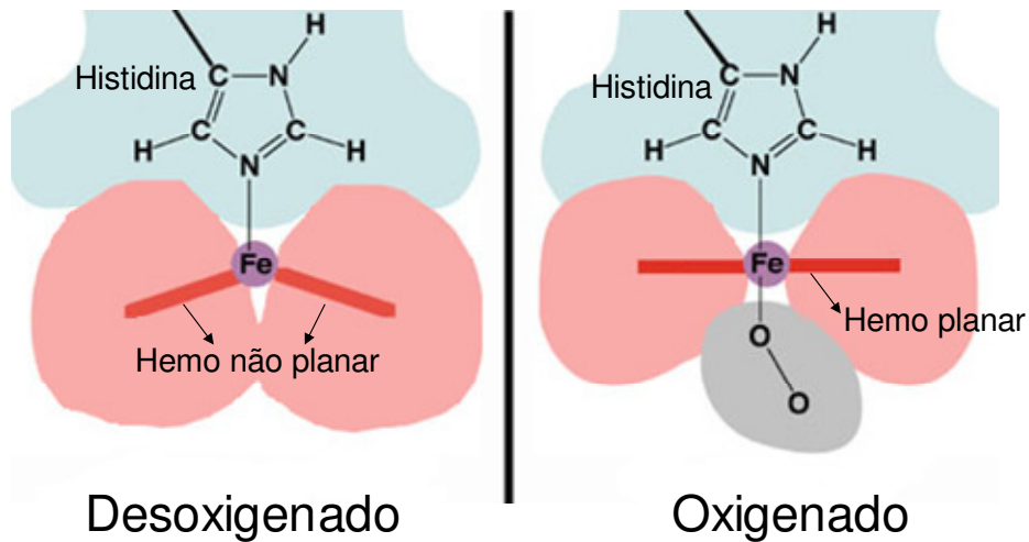
Figura 2.17. Representação da oxigenação da hemoglobina. Do lado esquerdo a forma desoxi – antes da ligação do O_2 e do lado direito a forma oxi – após a ligação com O_2 . O ferro move-se 0,6 \text{ \AA} em direção ao plano do hemo. Fonte: www.chemistry.wustl.edu .
