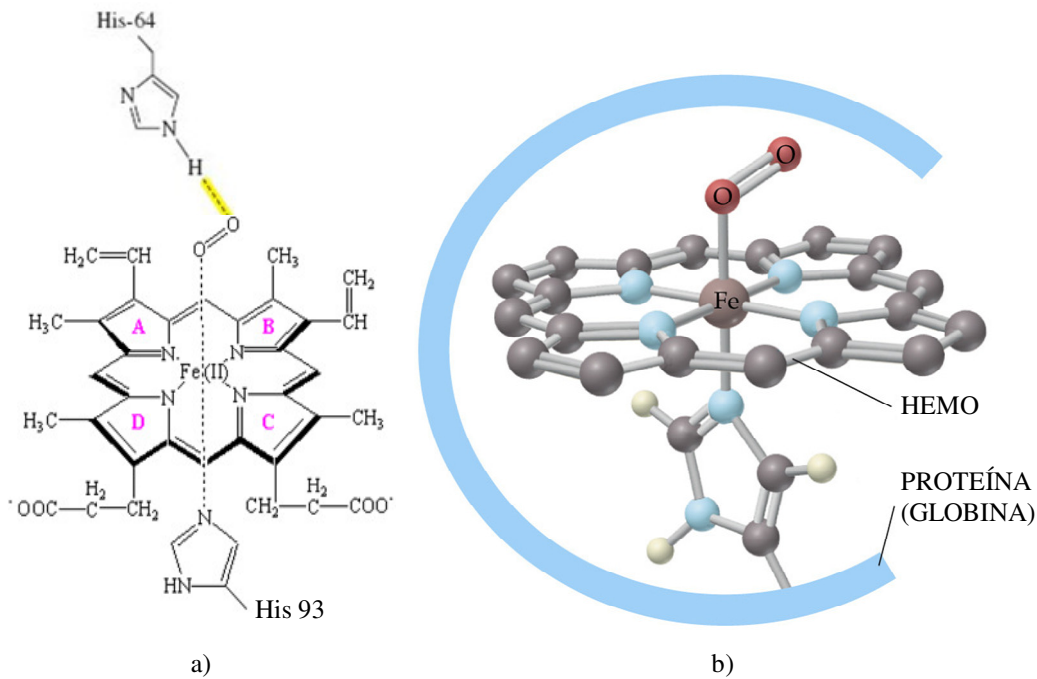
Figura 2.13. a) Representação planar do grupo prostético hemo, onde A, B, C e D são os anéis pirrólicos. b) Representação tridimensional do grupo prostético hemo na proteína reduzida a Fe^{+2} . Fonte: www.rasmol.org
