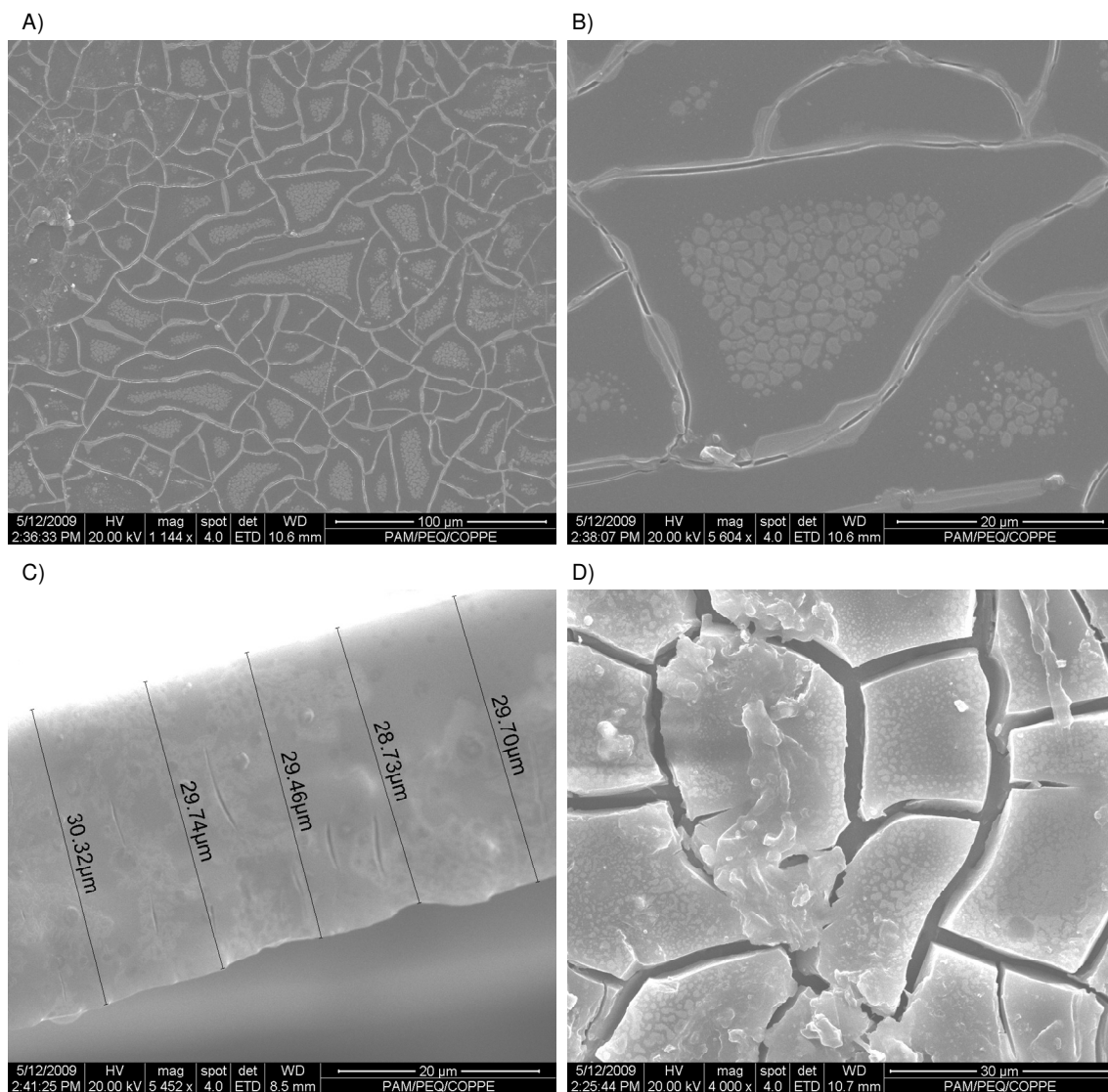
Figura 4.15. Fotomicrografias de MEV das membranas densas integrais de PVA/Hb. A) Camada superficial de PVA/oxiHb 8%; B) Detalhe da camada superficial de PVA/oxiHb 8%; C) Seção transversal de PVA/oxiHb 8%; D) Camada superficial de PVA/metHb 8%.
